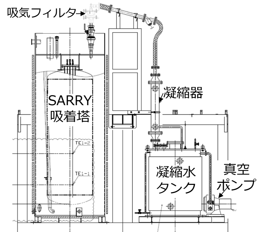
減圧乾燥設備概要
