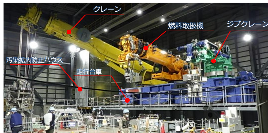
2号燃料取扱設備試験現場状況 (撮影：2025年9月8日)
