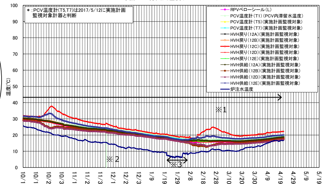
1号機 D/W雰囲気温度 (10/1~4/21)
