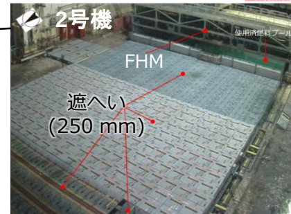
オペレーションフロアの遮へいの状況
