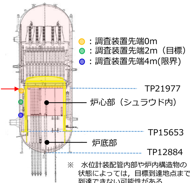
炉内構造物と調査範囲
