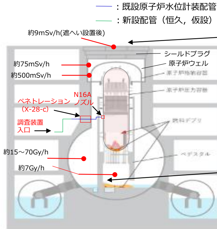
2号機原子炉建屋の状況（RPV内は未確認）
