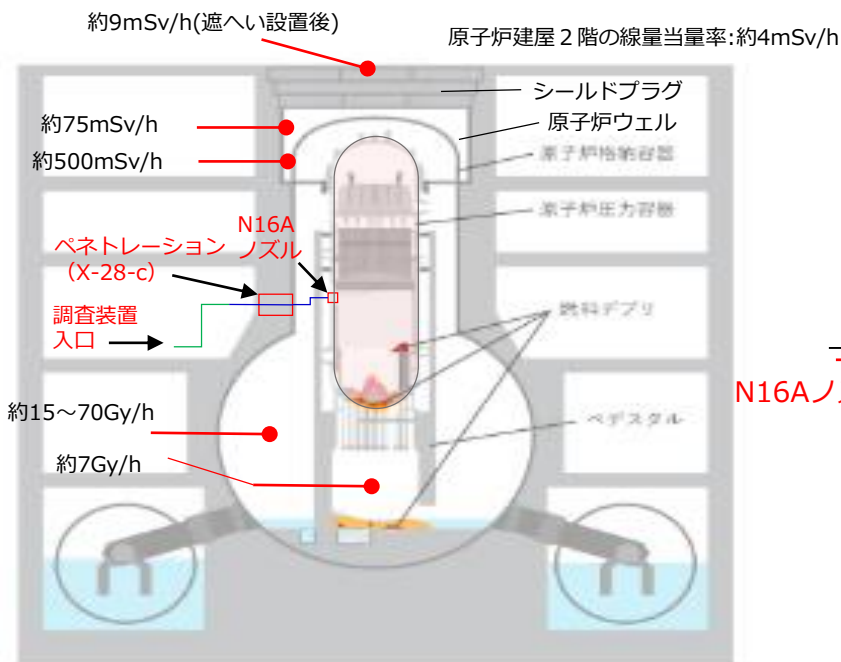
2号機原子炉建屋の状況
