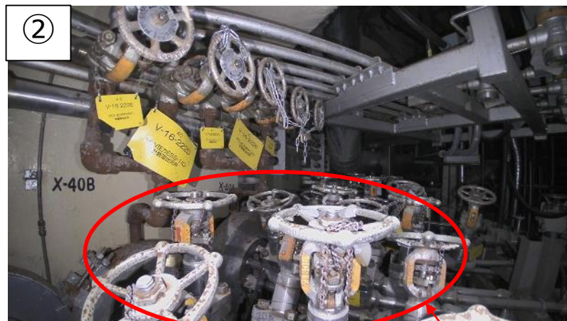
ジェットポンプ計装ライン
