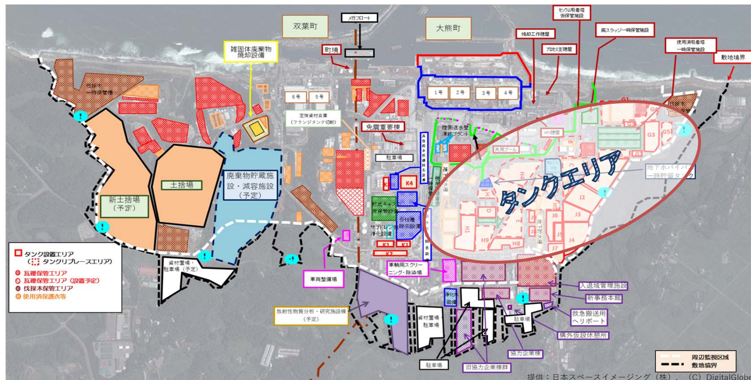
図 福島第一原発の構内図
