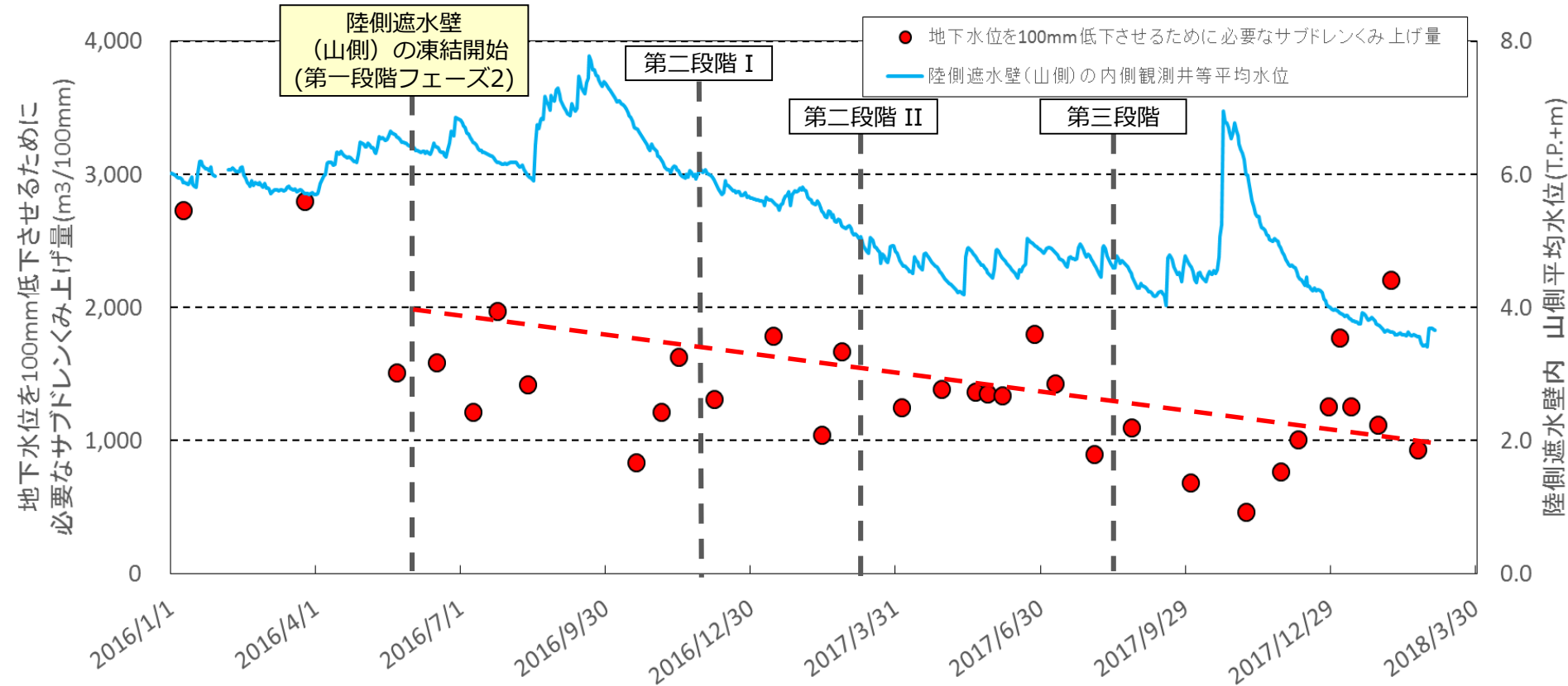
サブドレンのくみ上げ効率（陸側遮水壁（山側）の内側）
