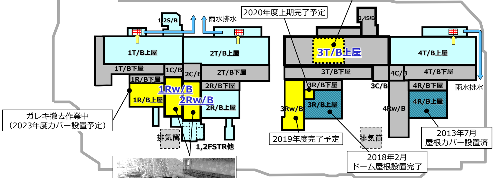
3T/B上屋 屋根状況 (2020年度上期完了予定)
