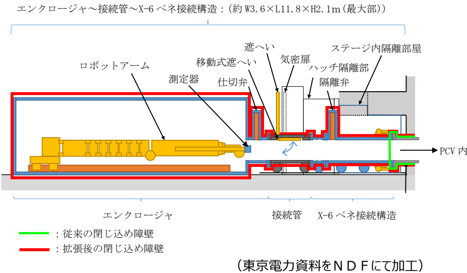
図 X-6 ペネ エンクロージャ等 構造概略図
