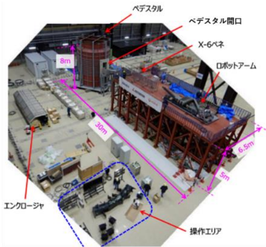
写真：櫛葉遠隔技術開発センター（JAEA）試験設備
