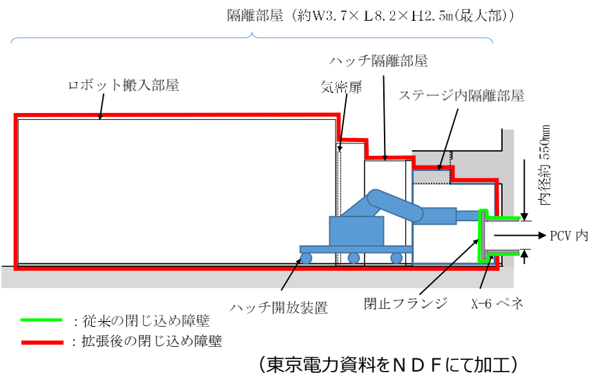
図 X-6 ペネ 隔離部屋 構造概略図
