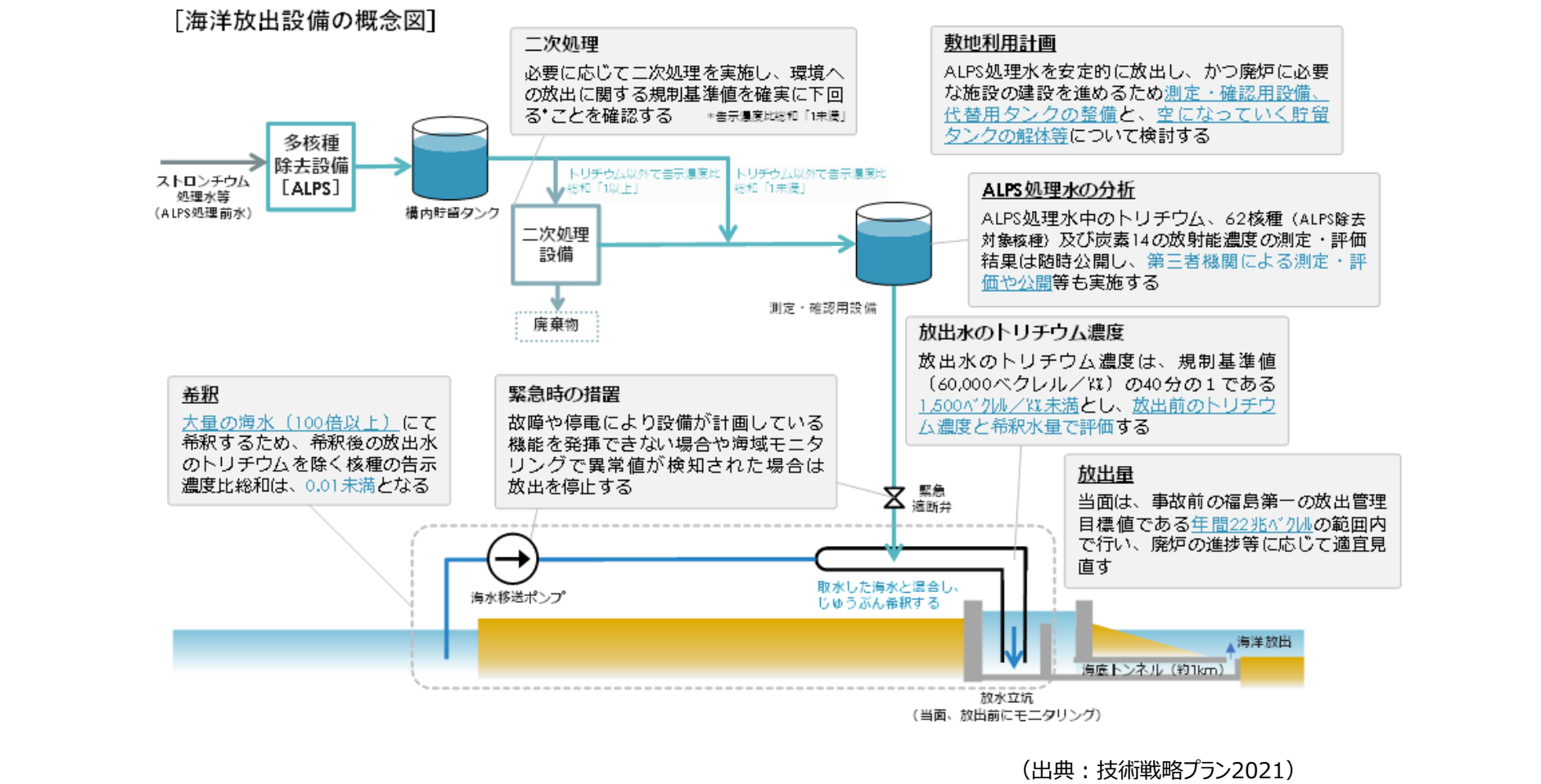
図 東京電力が計画する海洋放出設備の概念図
