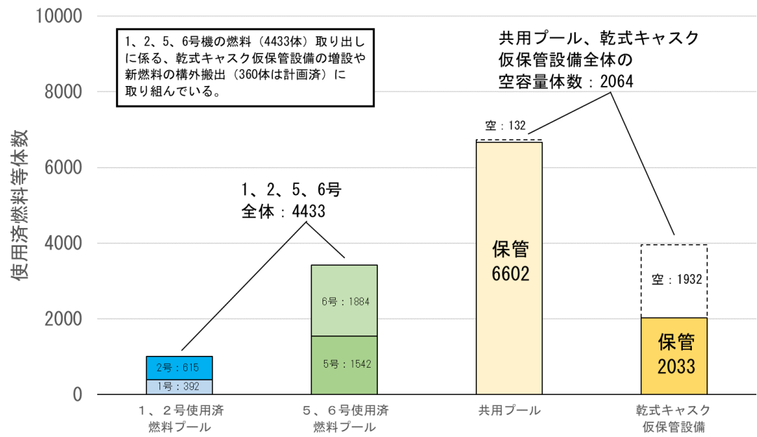
図 使用済燃料の保管状況（2022年5月時点）
