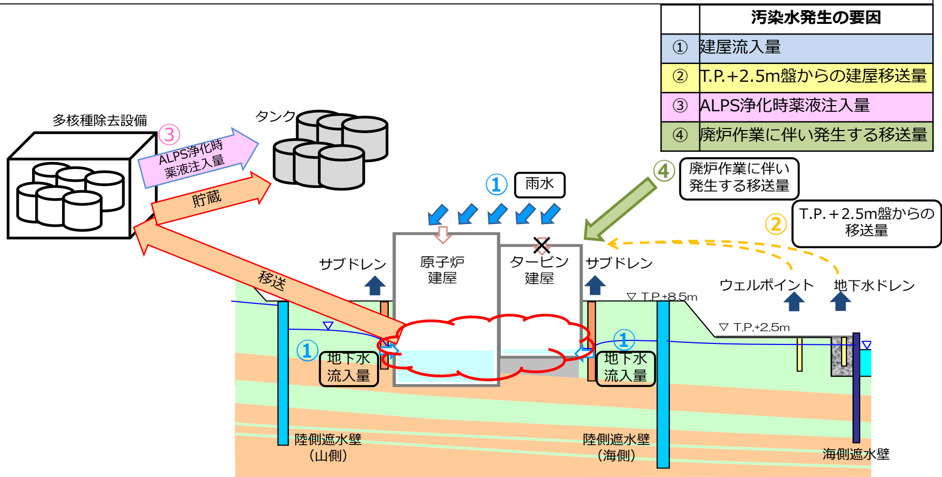
建屋周辺における水の出入り概念図
