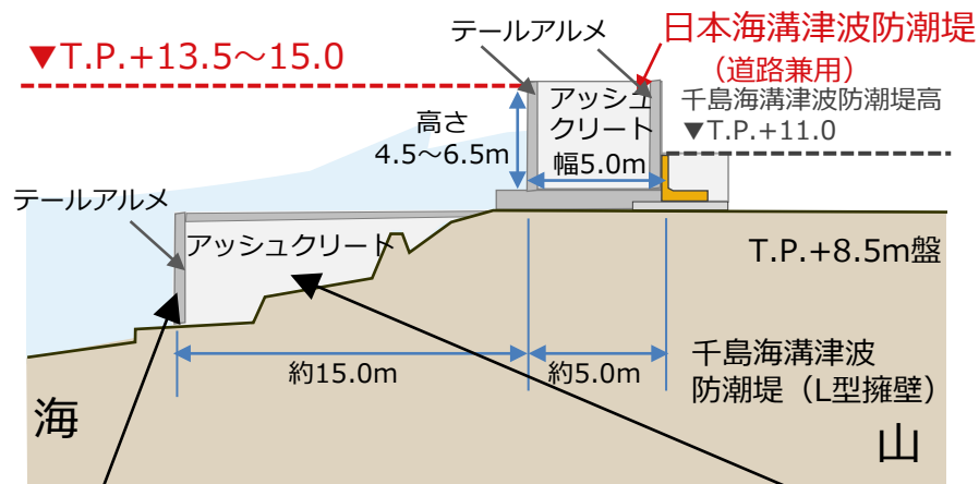
テールアルメ設置状況
