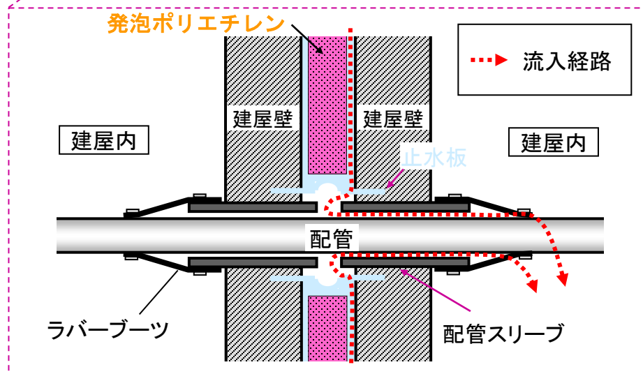
建屋間ギャップからの流入イメージ
