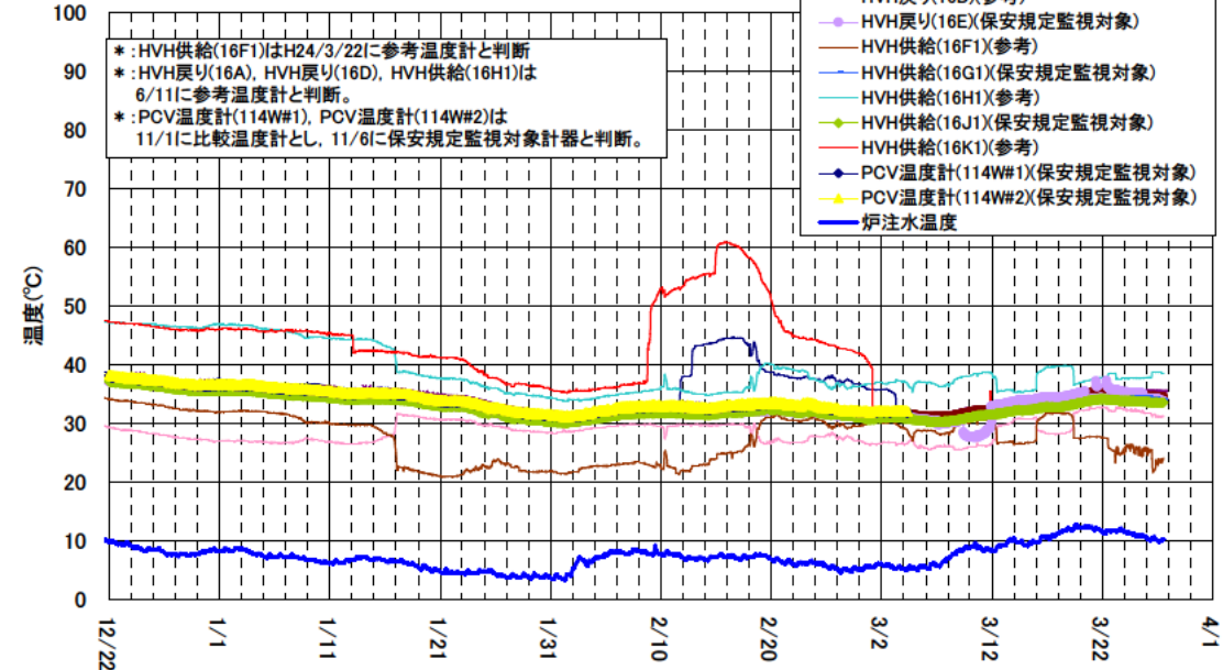
2号機 D/W雰囲気温度 (12/22~3/27)
