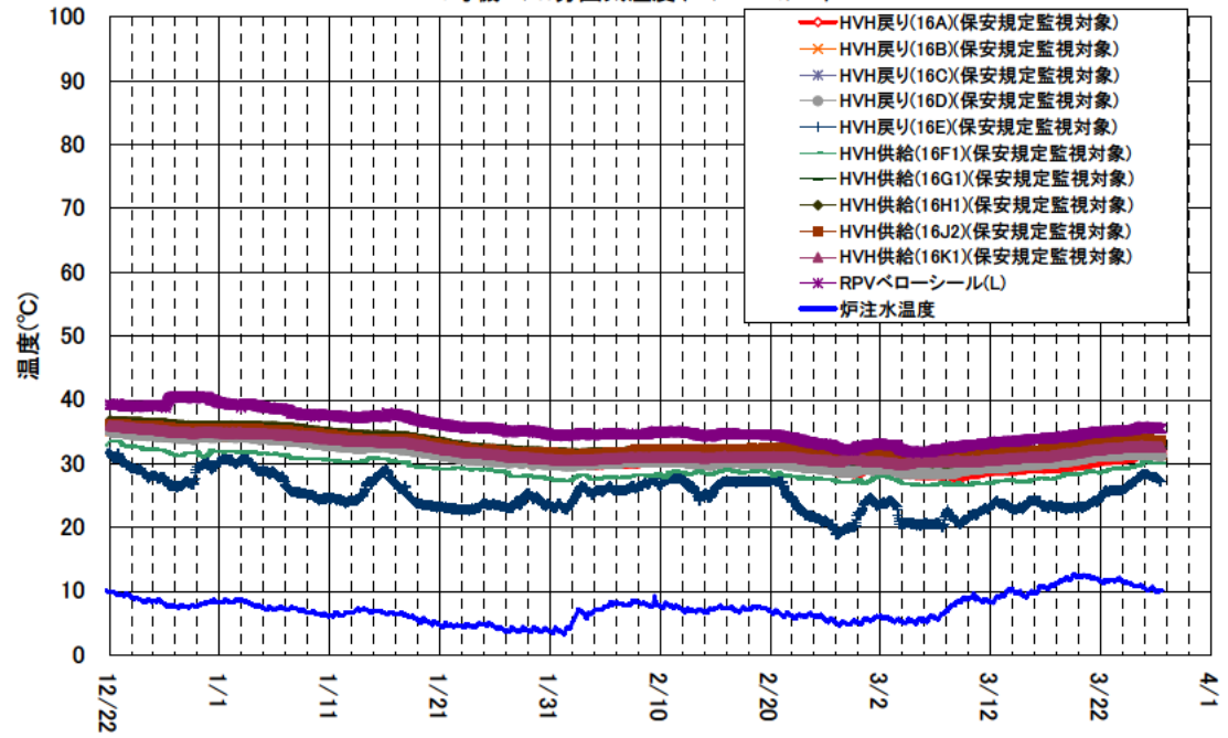
3号機 D/W雰囲気温度(12/22~3/27)
