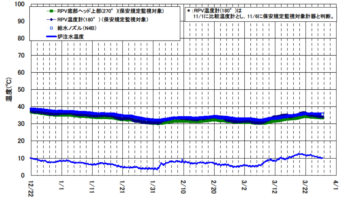
2号機 原子炉圧力容器まわり温度 (12/22~3/27)
