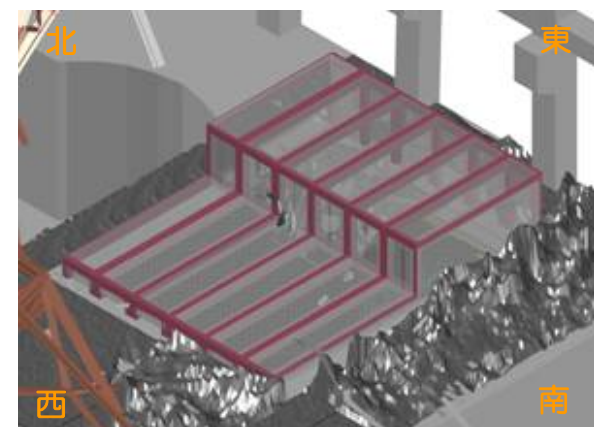
使用済燃料貯蔵プール養生（第二段階） イメージ図
