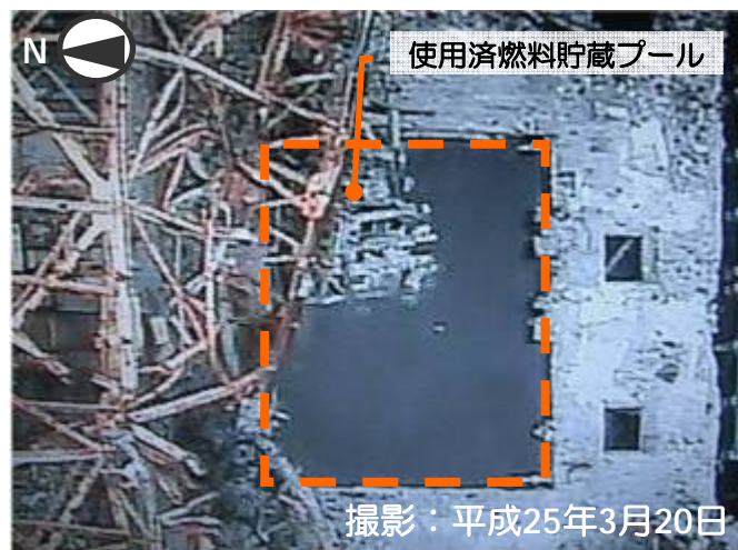
使用済燃料貯蔵プール養生（第一段階）設置前
