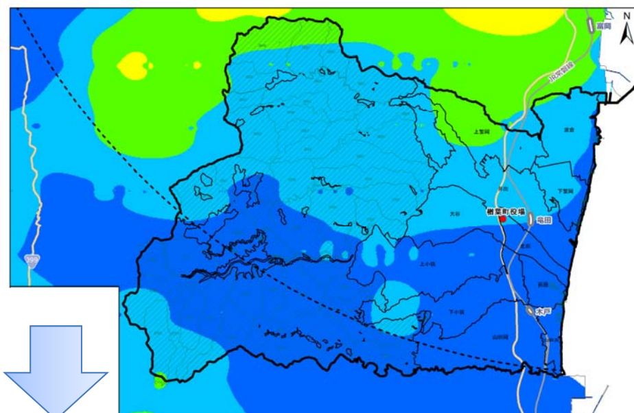
檜葉町 第5次航空機モニタリング結果(2012年6月28日時点の線量分布)
