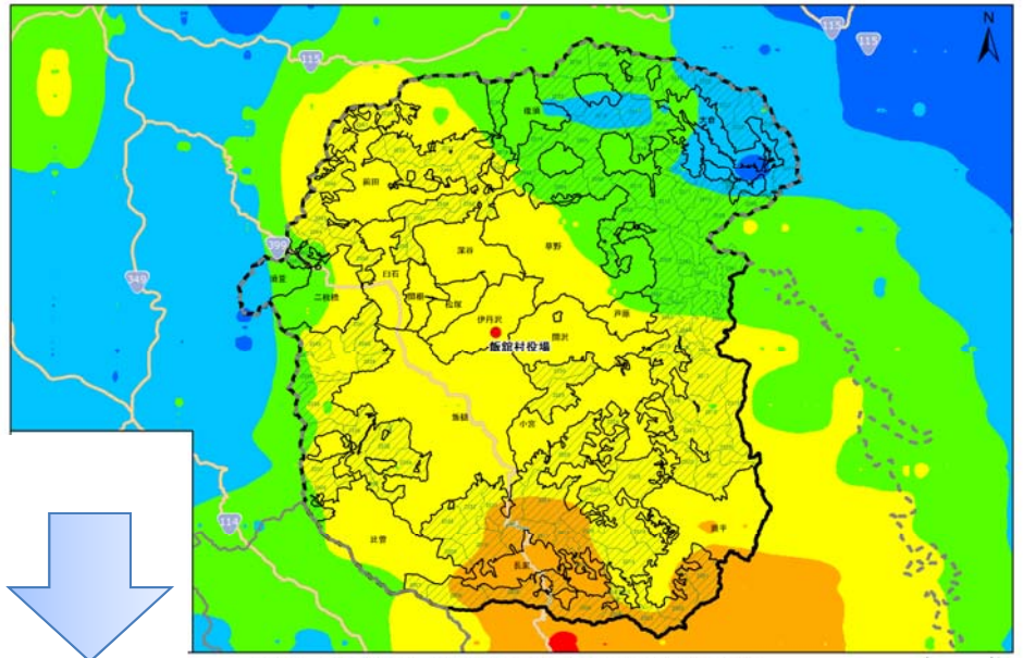
飯舘村 第4次航空機モニタリング結果(2011年11月5日時点の線量分布)
