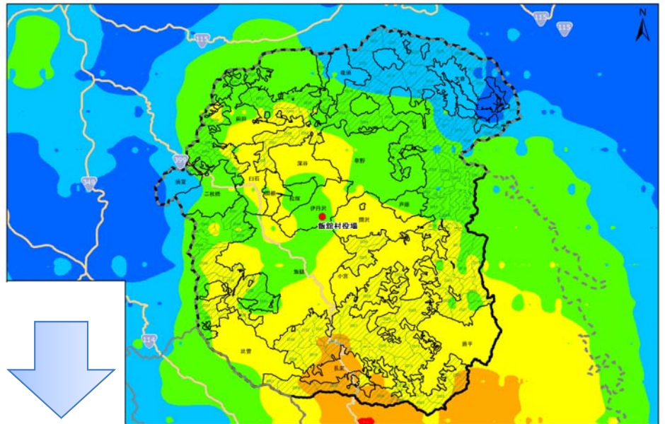
飯舘村 第5次航空機モニタリング結果(2012年6月28日時点の線量分布)
