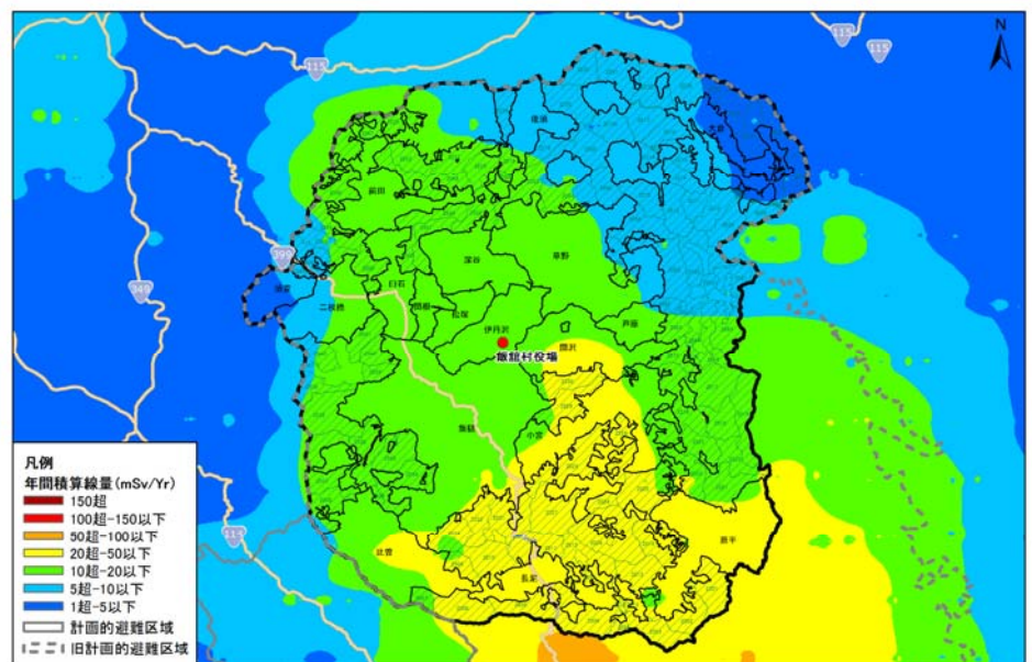
飯舘村 第6次航空機モニタリング結果(2012年11月16日時点の線量分布)
