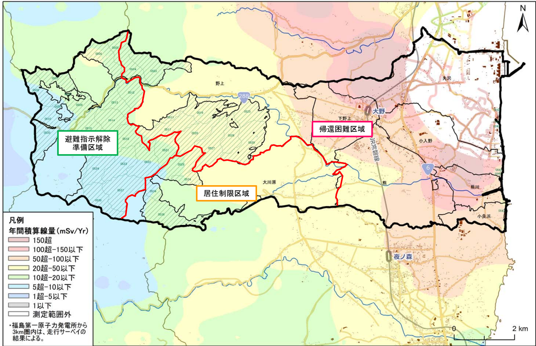
大熊町 2012年3月31日時点の線量分布(2012年2月の航空機モニタリング結果を基に予測)
