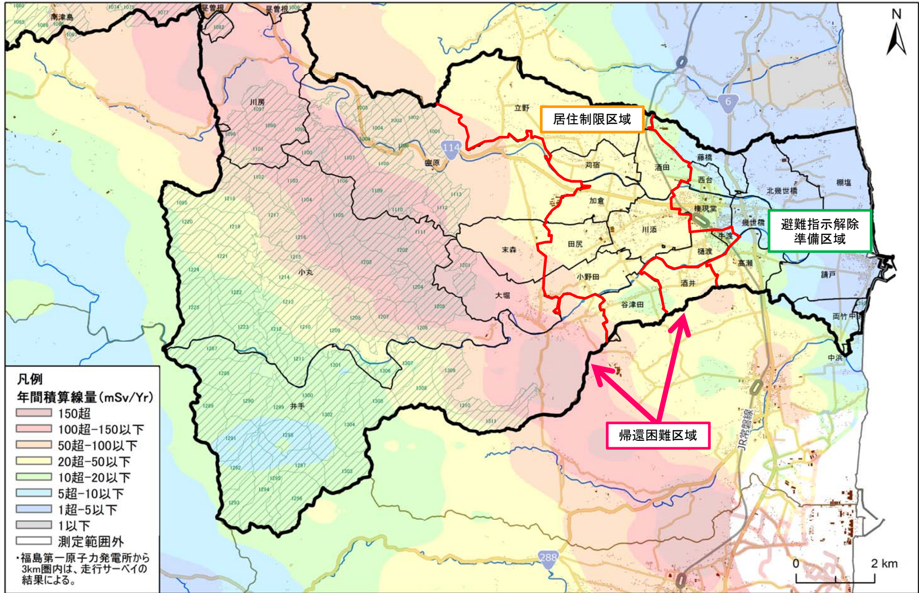
浪江町(その1) 2012年3月31日時点の線量分布(2012年2月の航空機モニタリング結果を基に予測)
