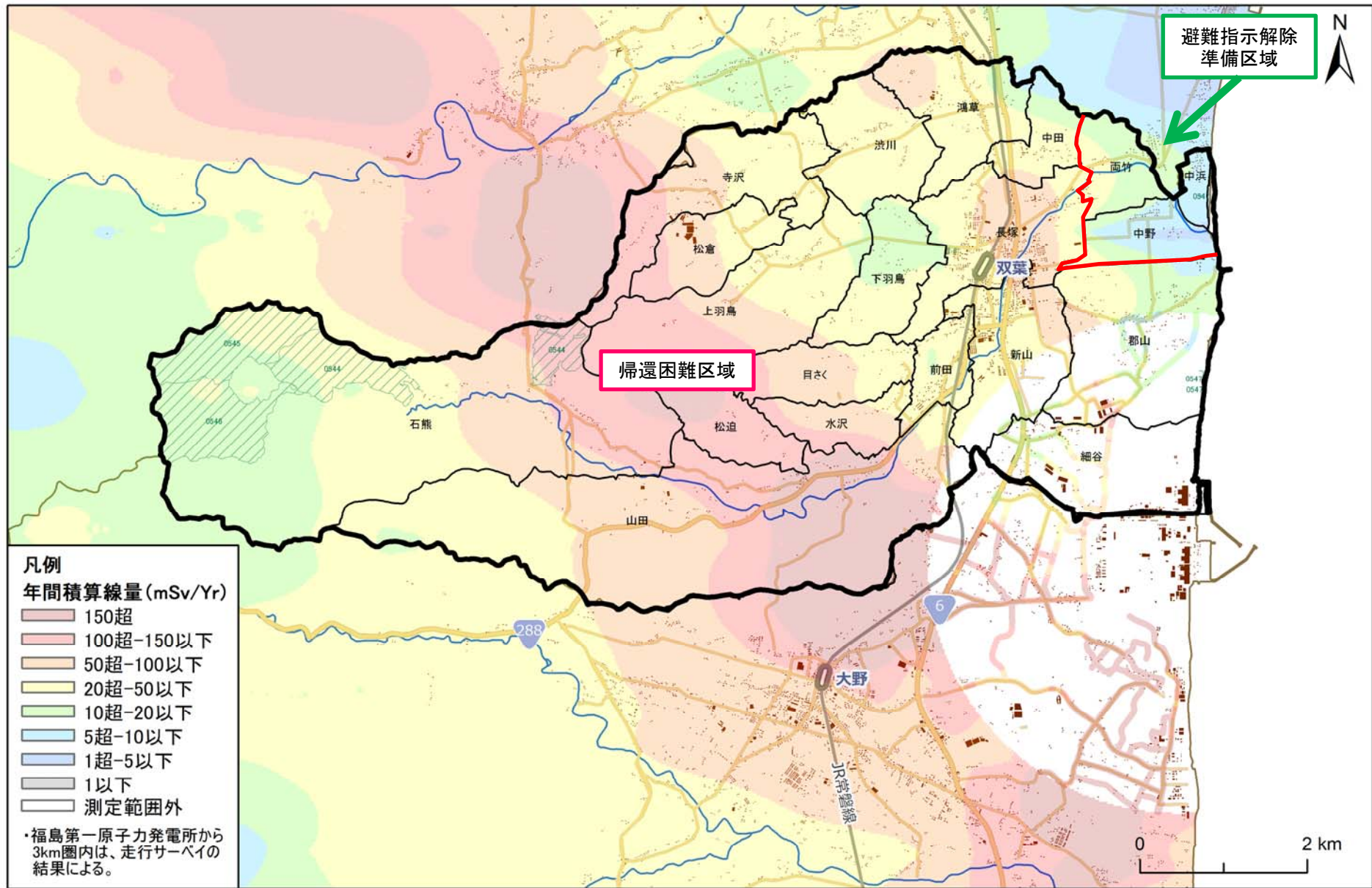
双葉町 2012年3月31日時点の線量分布(2012年2月の航空機モニタリング結果を基に予測)
