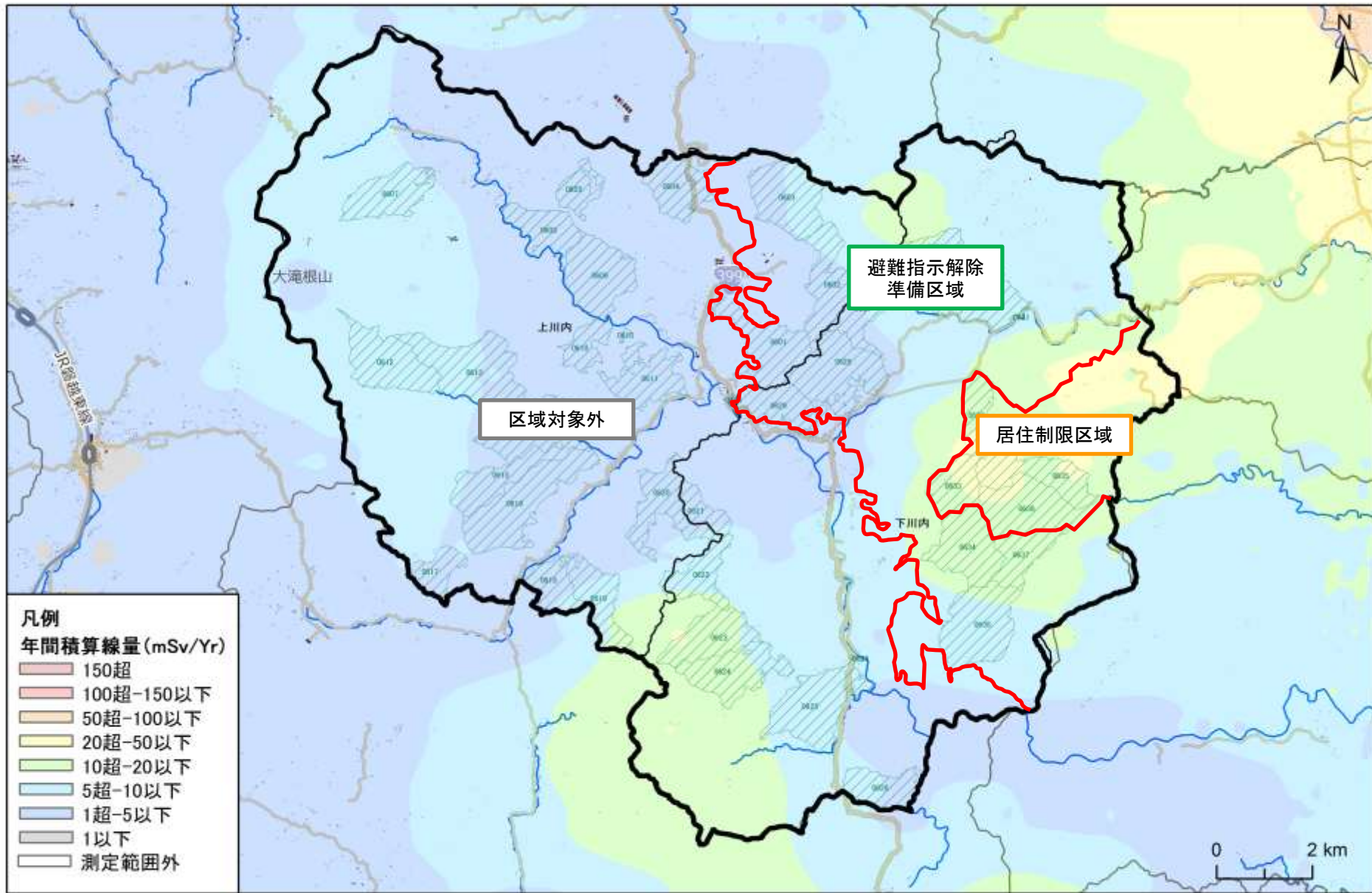
川内村 2012年3月31日時点の線量分布(2011年11月の航空機モニタリング結果を基に予測)
