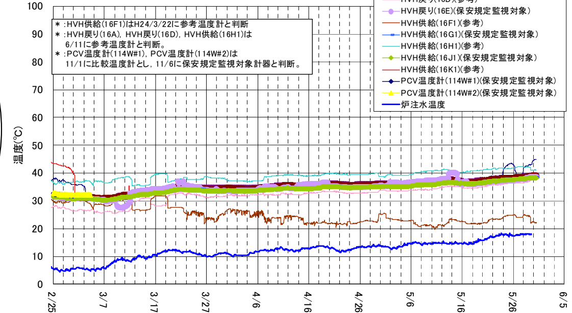
2号機 D/W雰囲気温度(2/25~5/29)
