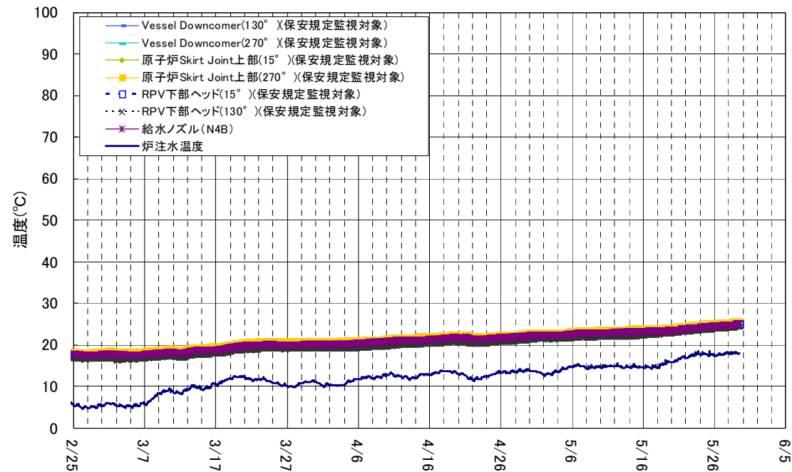
1号機 原子炉圧力容器まわり温度(2/25~5/29)
