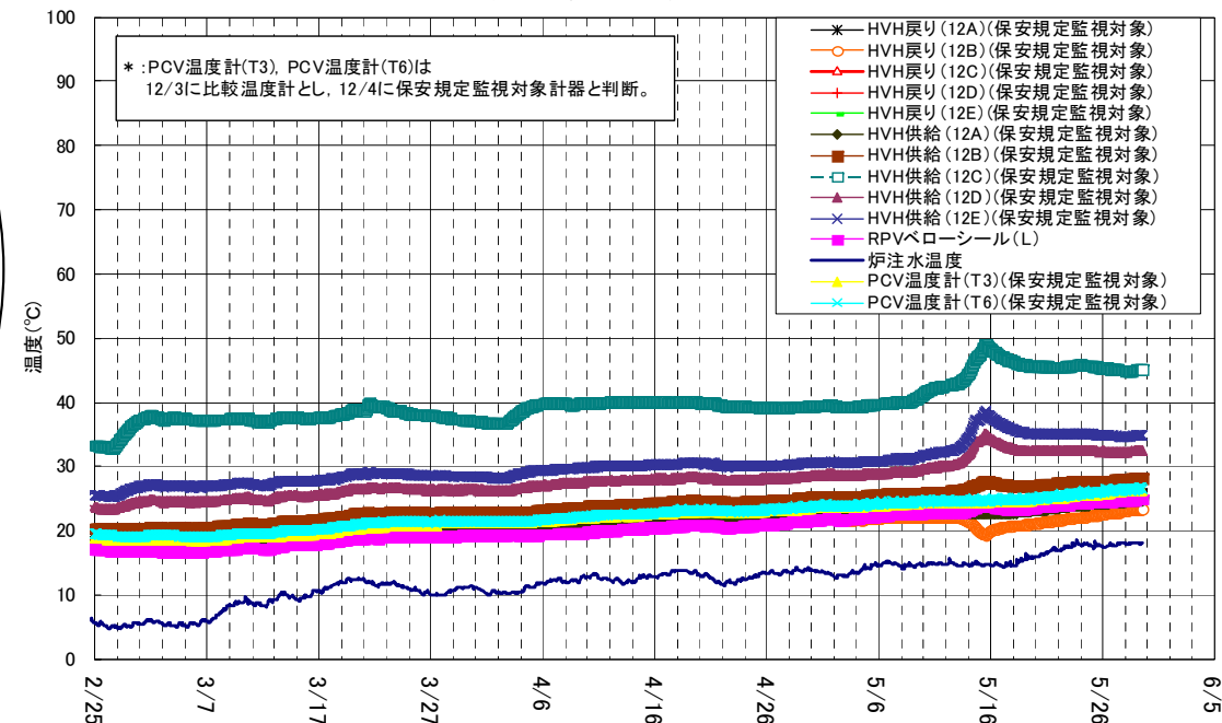
1号機 D/W雰囲気温度(2/25~5/29)
