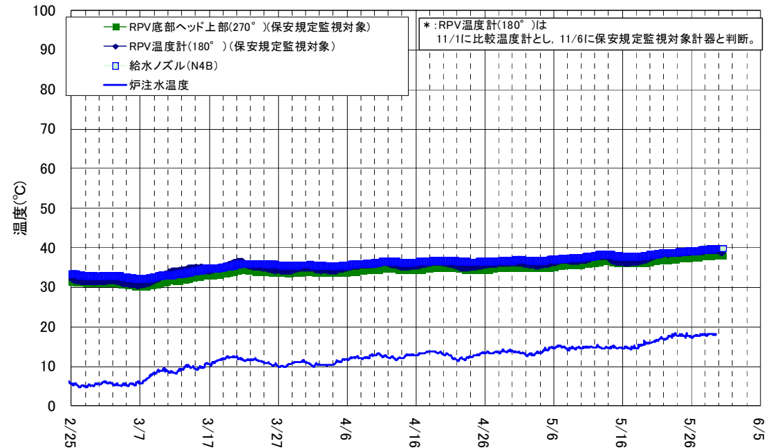
2号機 原子炉圧力容器まわり温度(2/25~5/29)
