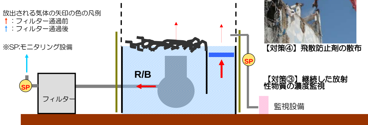
概略構成図
