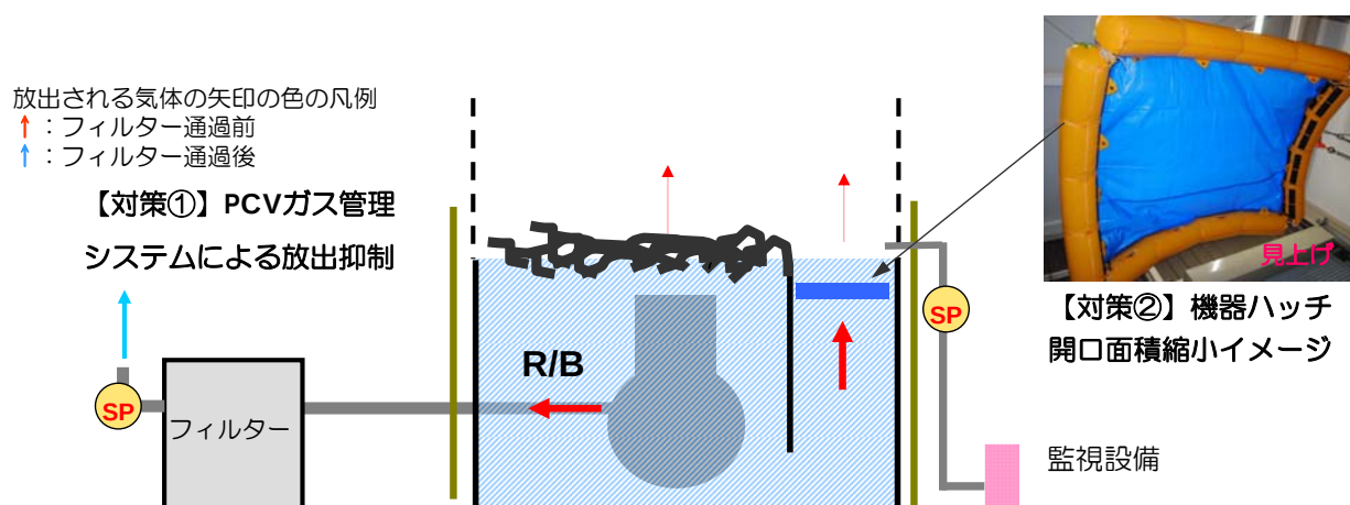
概略構成図
