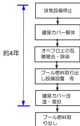
プール燃料取り出しフロー
