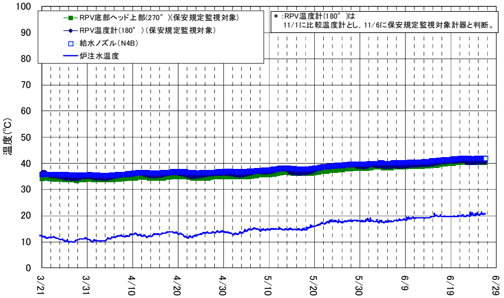
2号機 原子炉圧力容器まわり温度(3/21~6/26)
