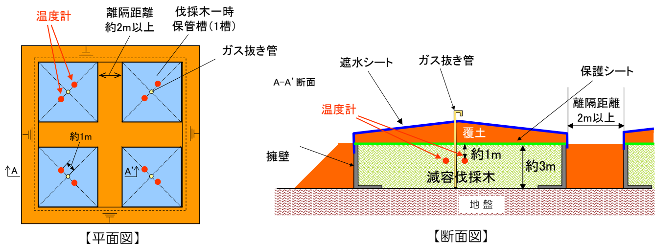
伐採木一時保管槽 溫度計位置概略図
