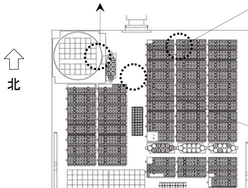
SFP内 キャスケピット内 (炉内機器移動ルート確認)
