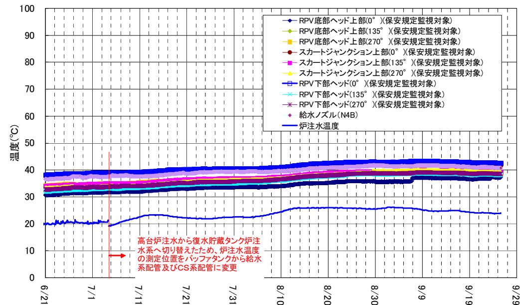
3号機 原子炉压力容器まわり温度 (6/21~9/25)
