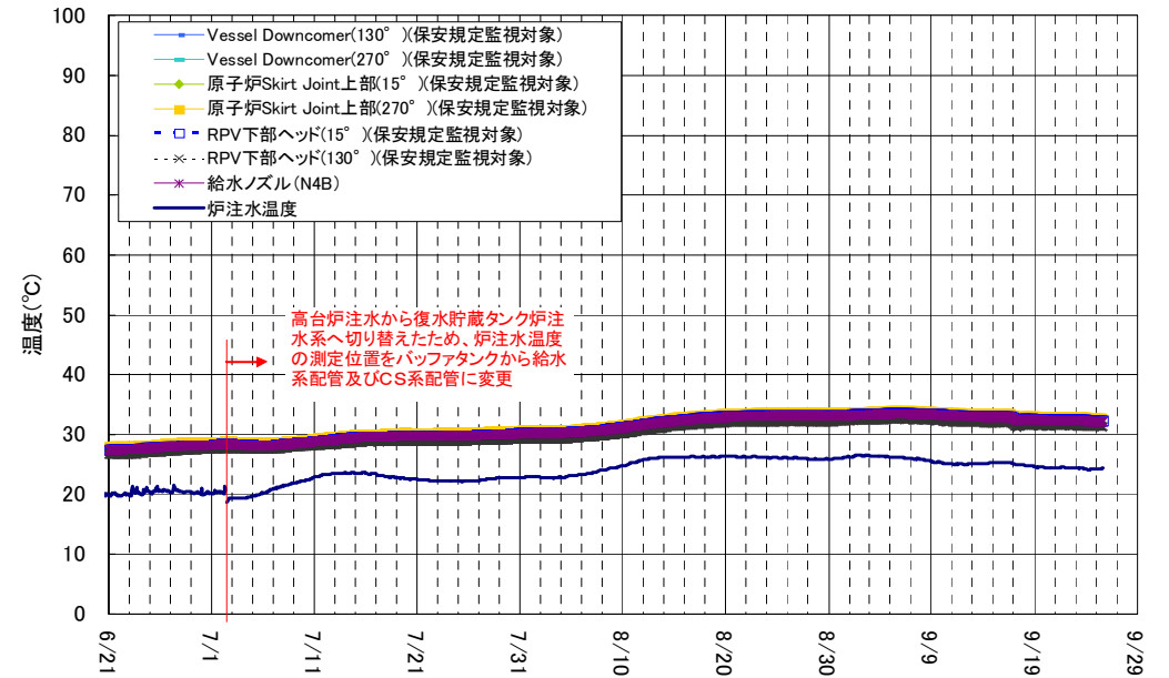
1号機 原子炉圧力容器まわり温度 (6/21~9/25)
