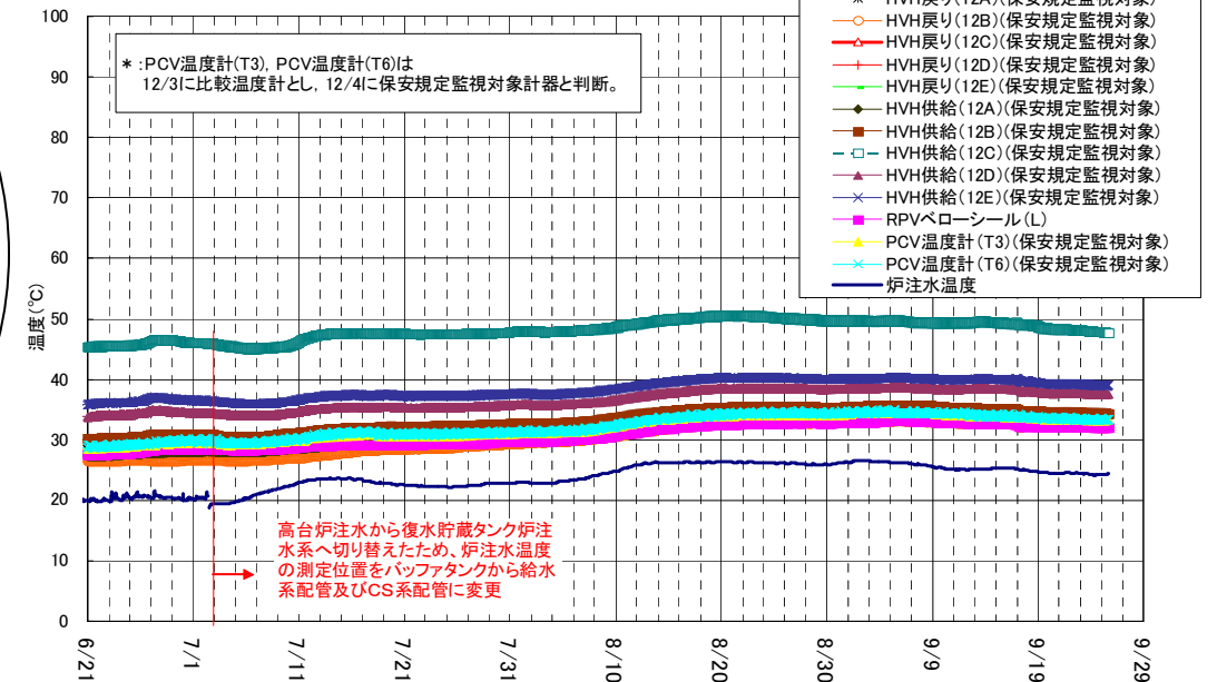
1号機 D/W雰囲気温度 (6/21~9/25)
