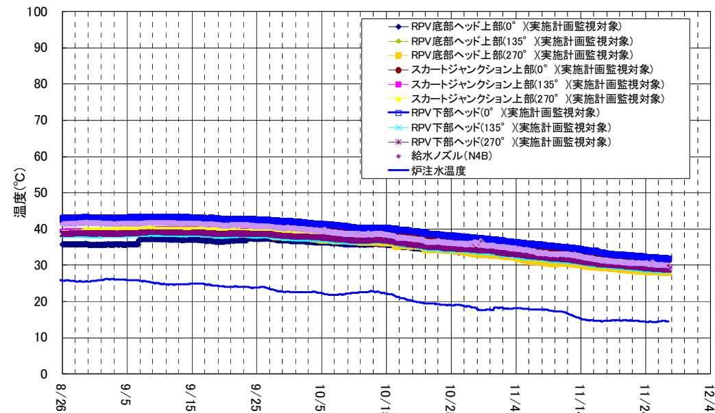
3号機 原子炉圧力容器まわり温度 (8/26~11/27)
