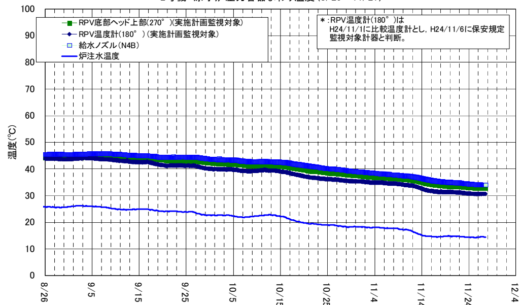
2号機 原子炉圧力容器まわり温度 (8/26～11/27)
