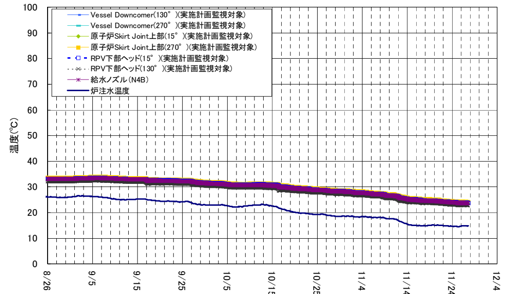
1号機 原子炉圧力容器まわり温度 (8/26～11/27)
