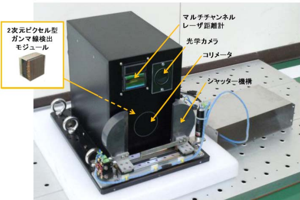
図4 ガンマカメラ外観
