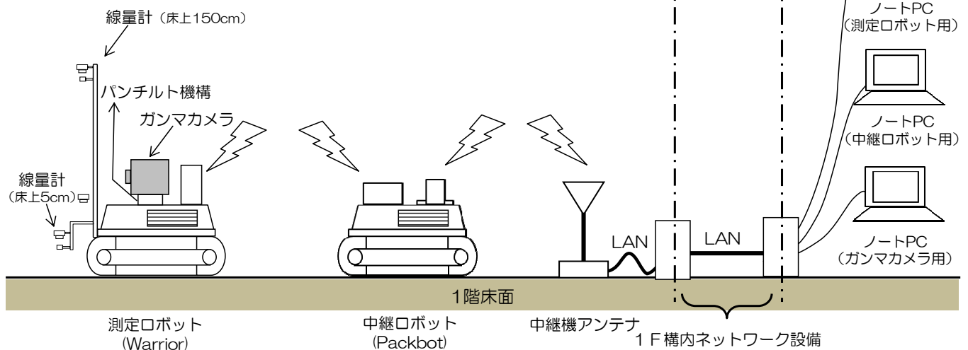
図3 調査装置構成
