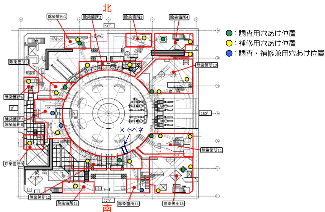
図6 PCV調査・補修のための穴あけ予定位置
