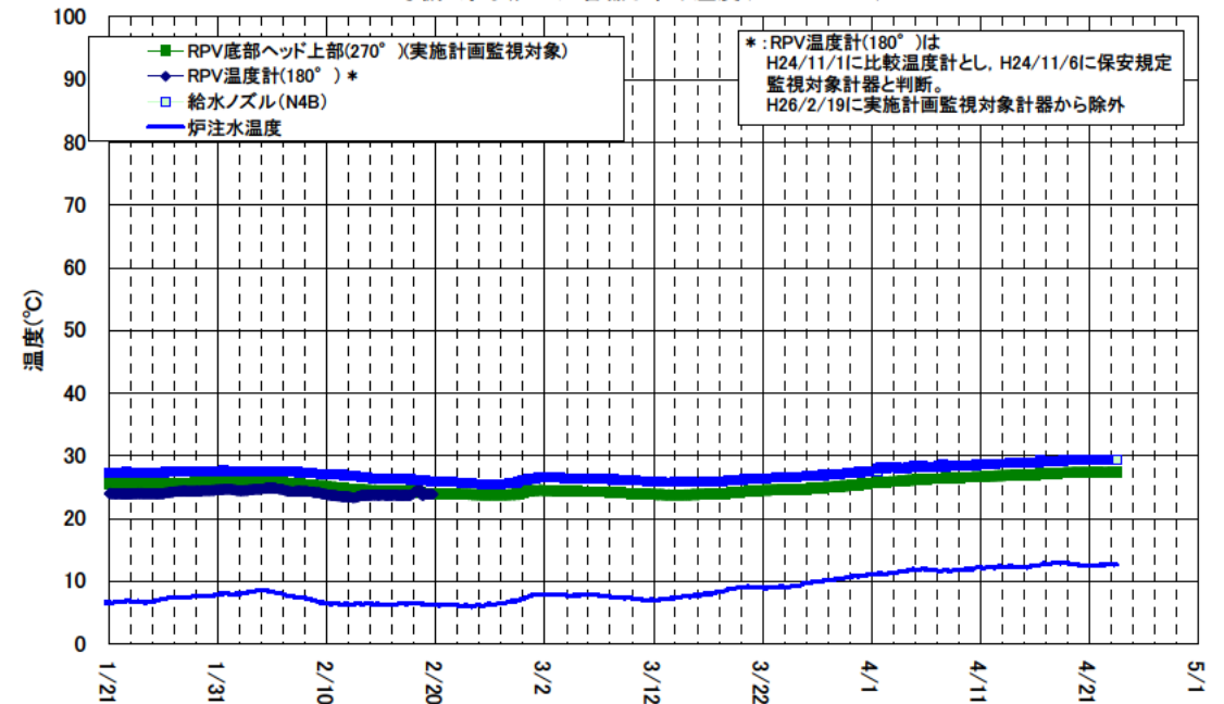
2号機 原子炉圧力容器まわり温度(1/21~4/23)
