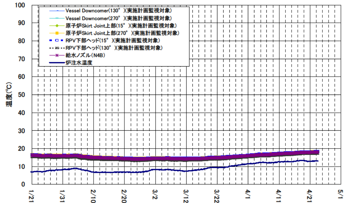
1号機 原子炉圧力容器まわり温度(1/21~4/23)
