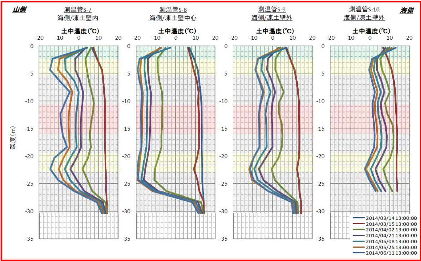
■測定データ【海側凍土壁面 中心測線】
