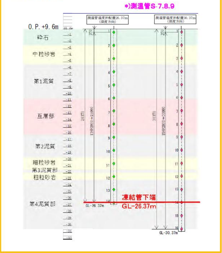
■測温管構造
