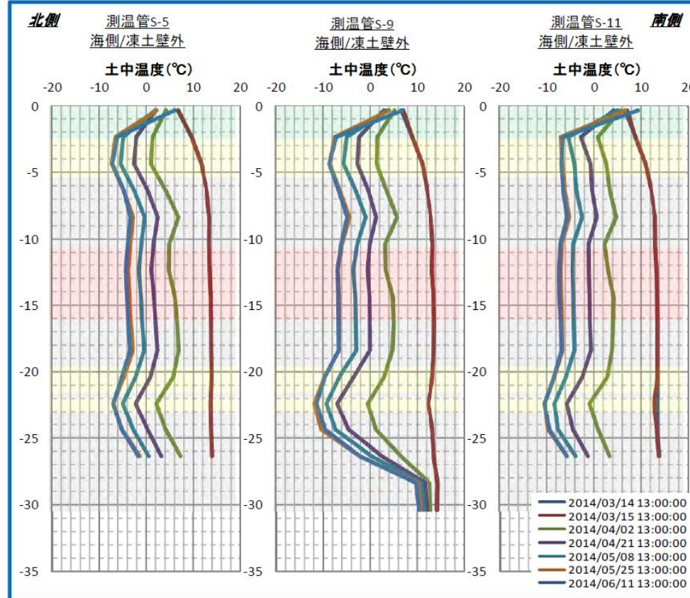
■測定データ【海側凍土壁面】
