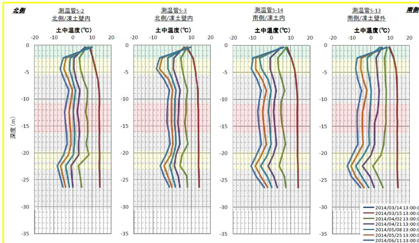
■測定データ【南北凍土壁面 中心測線】
