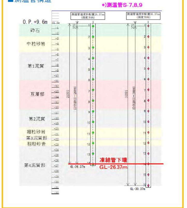
■測温管構造
