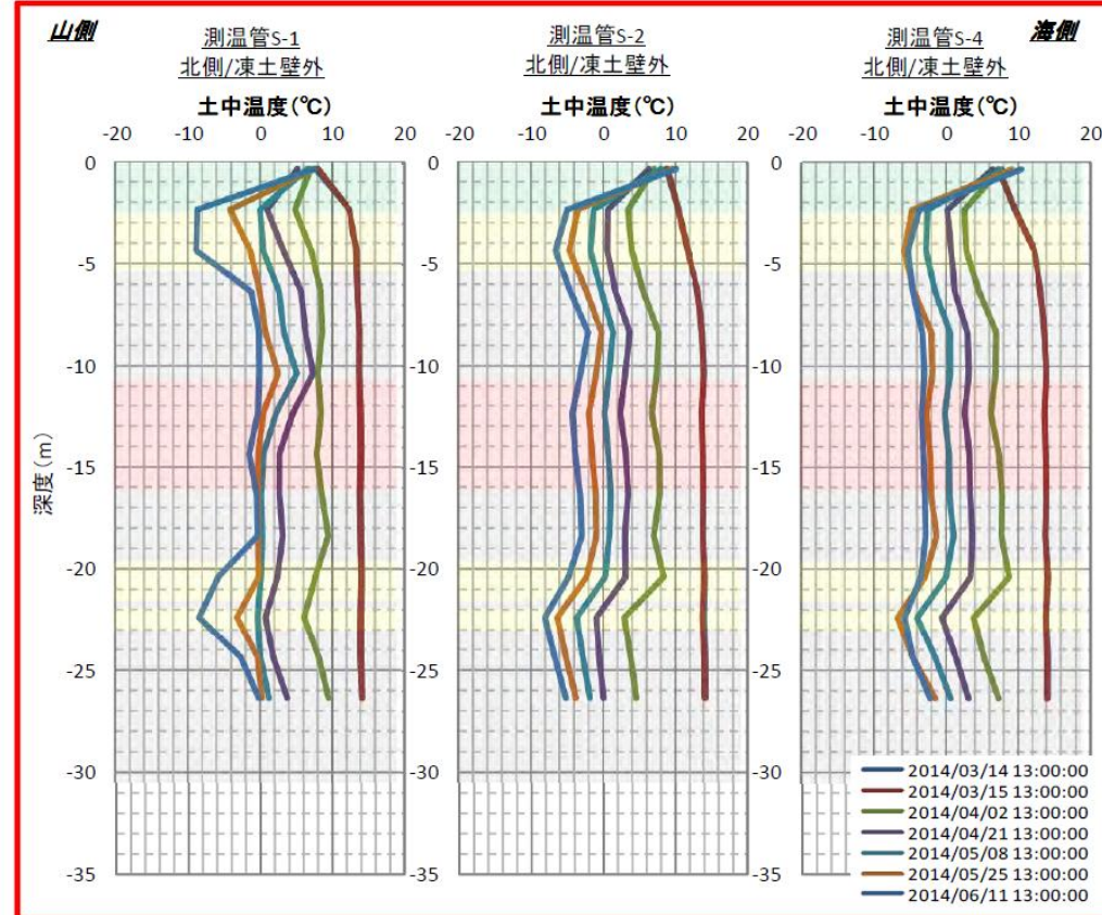
■測定データ【北側凍土壁面】
