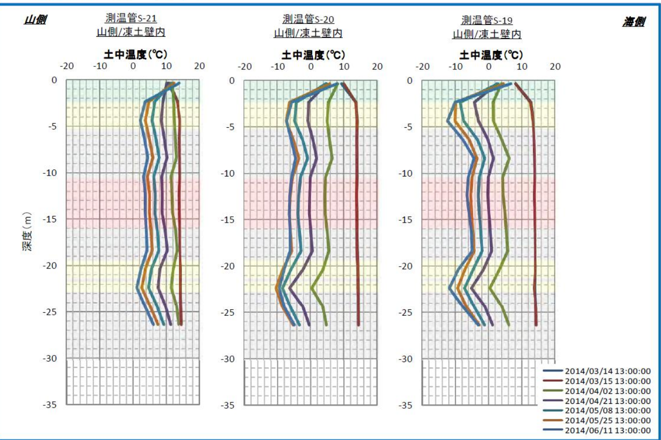
■測定データ【山側凍土壁面 中心測線】
