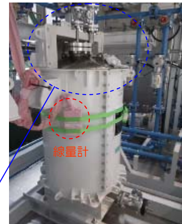
吸着塔
