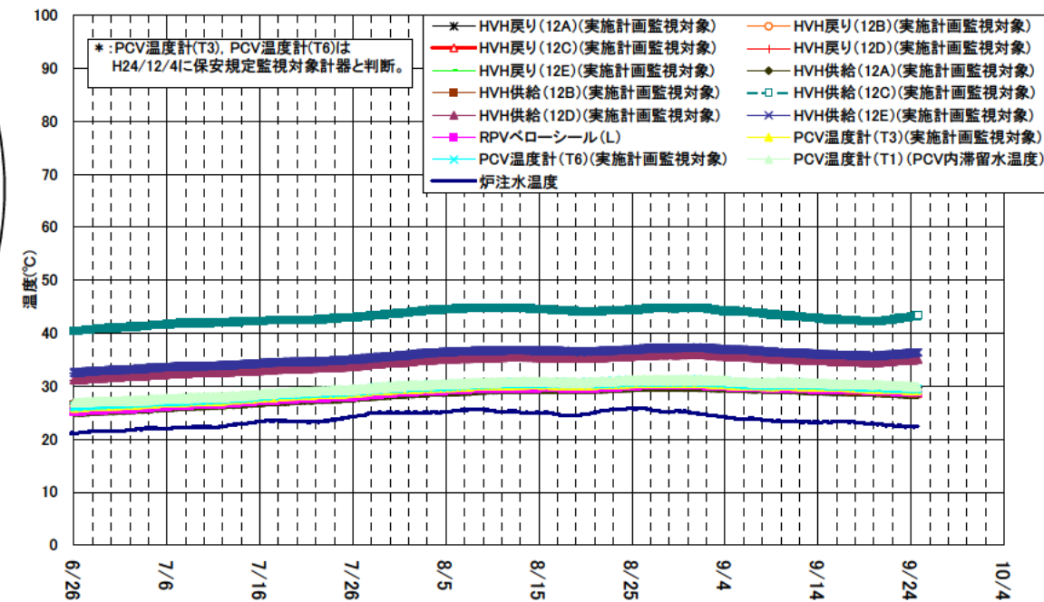
1号機 D/W雰囲気温度(6/26~9/24)
