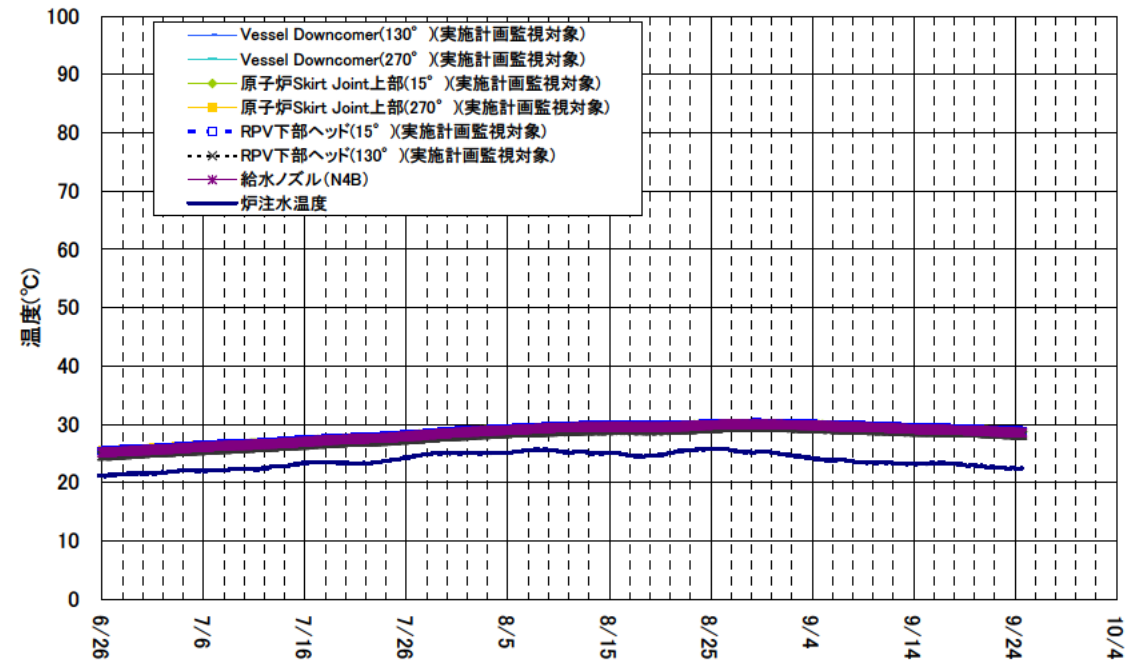
1号機 原子炉圧力容器まわり温度(6/26~9/24)
