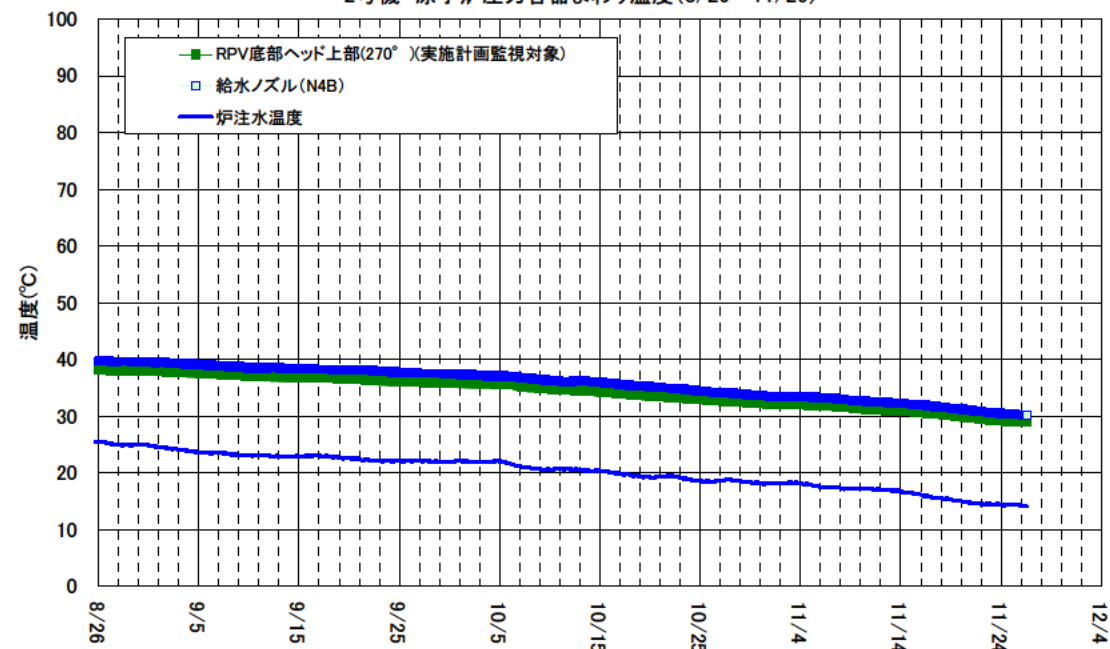
2号機 原子炉圧力容器まわり温度(8/26～11/26)
