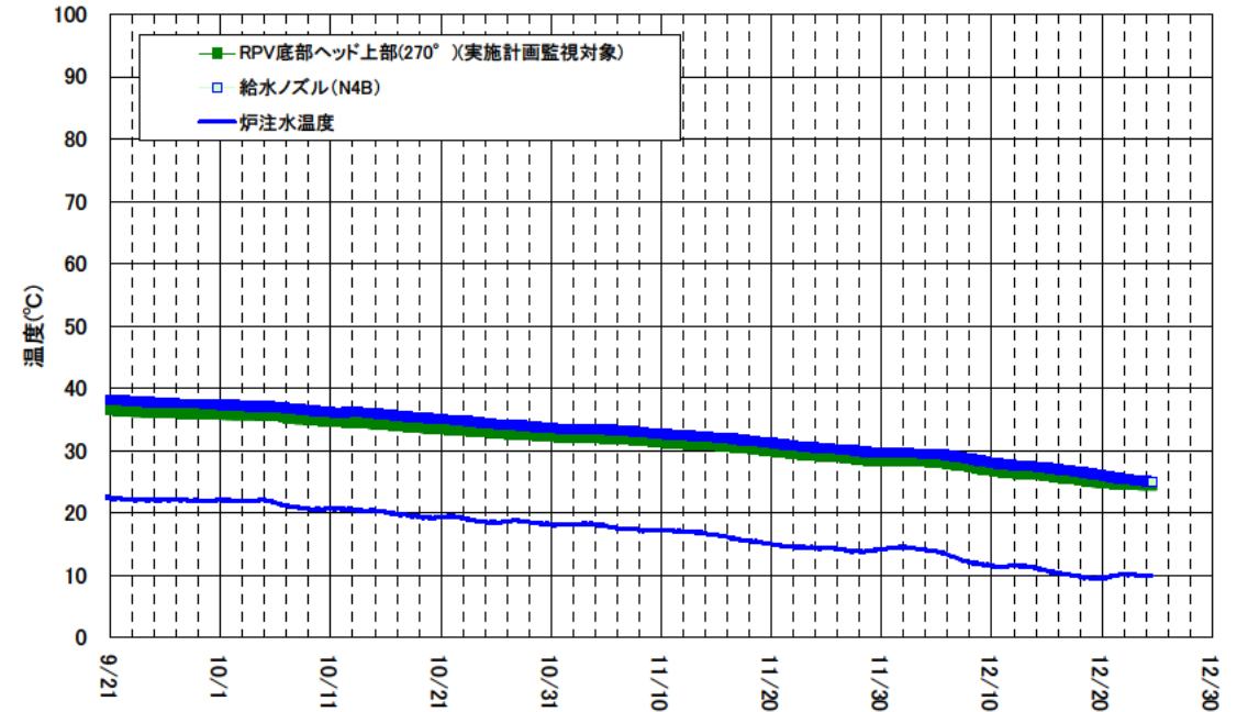
2号機 原子炉圧力容器まわり温度(9/21~12/24)
