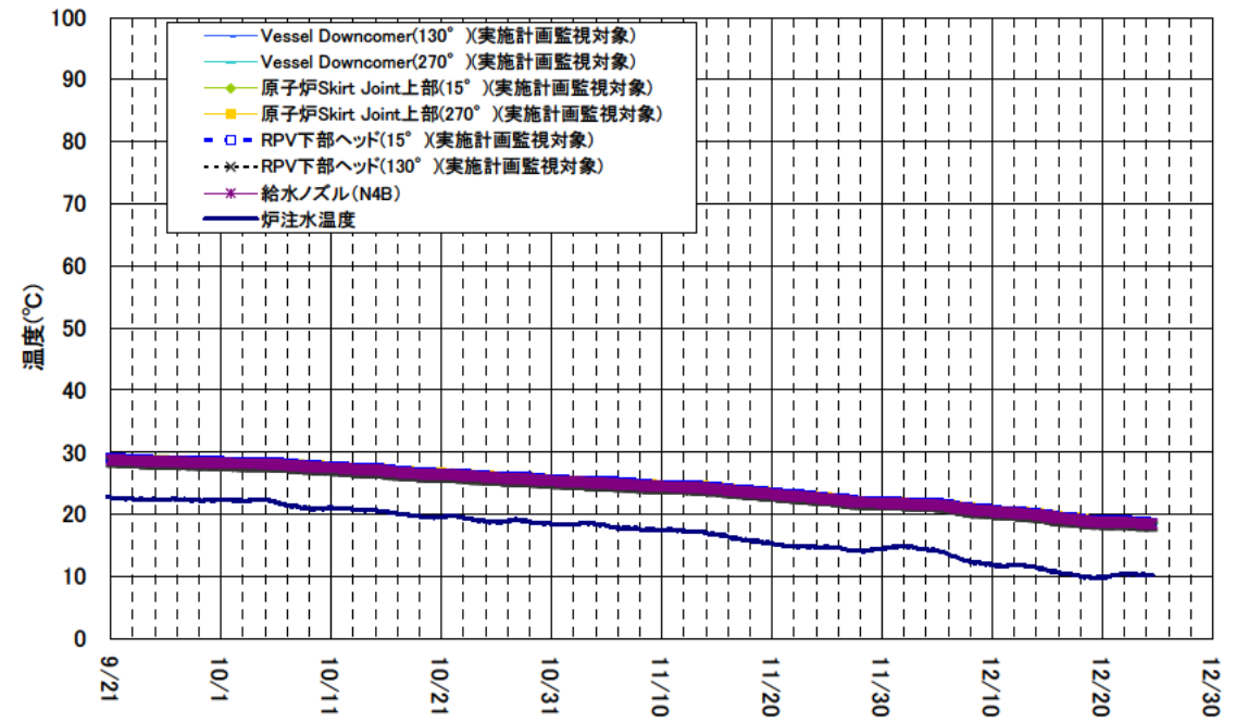
1号機 原子炉圧力容器まわり温度(9/21~12/24)
