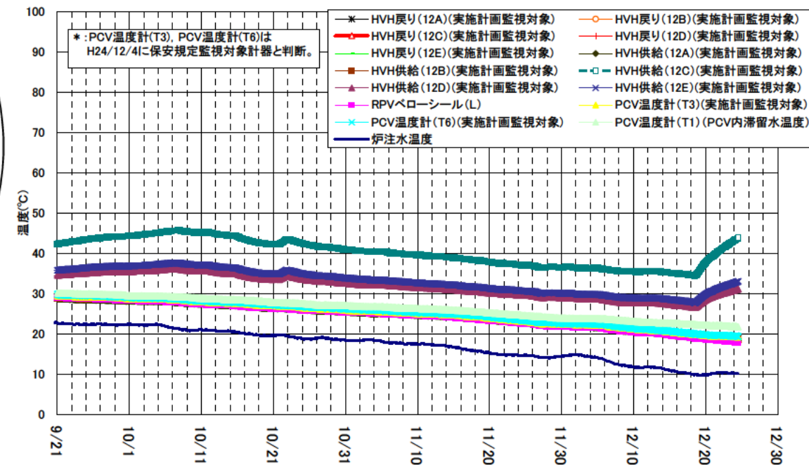
1号機 D/W雰囲気温度(9/21~12/24)
