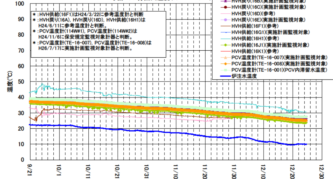
2号機 D/W雰囲気温度(9/21~12/24)
