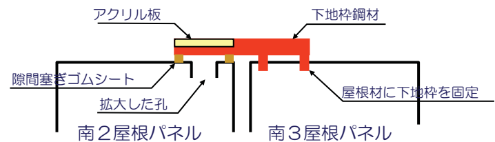
概念図（断面図）
