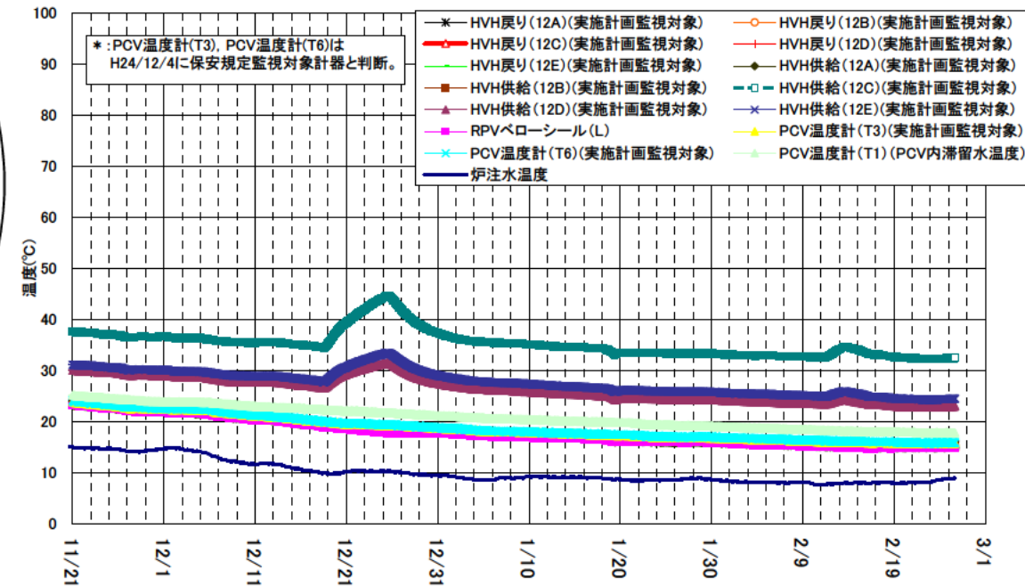
1号機 D/W雰囲気温度(11/21~2/25)
