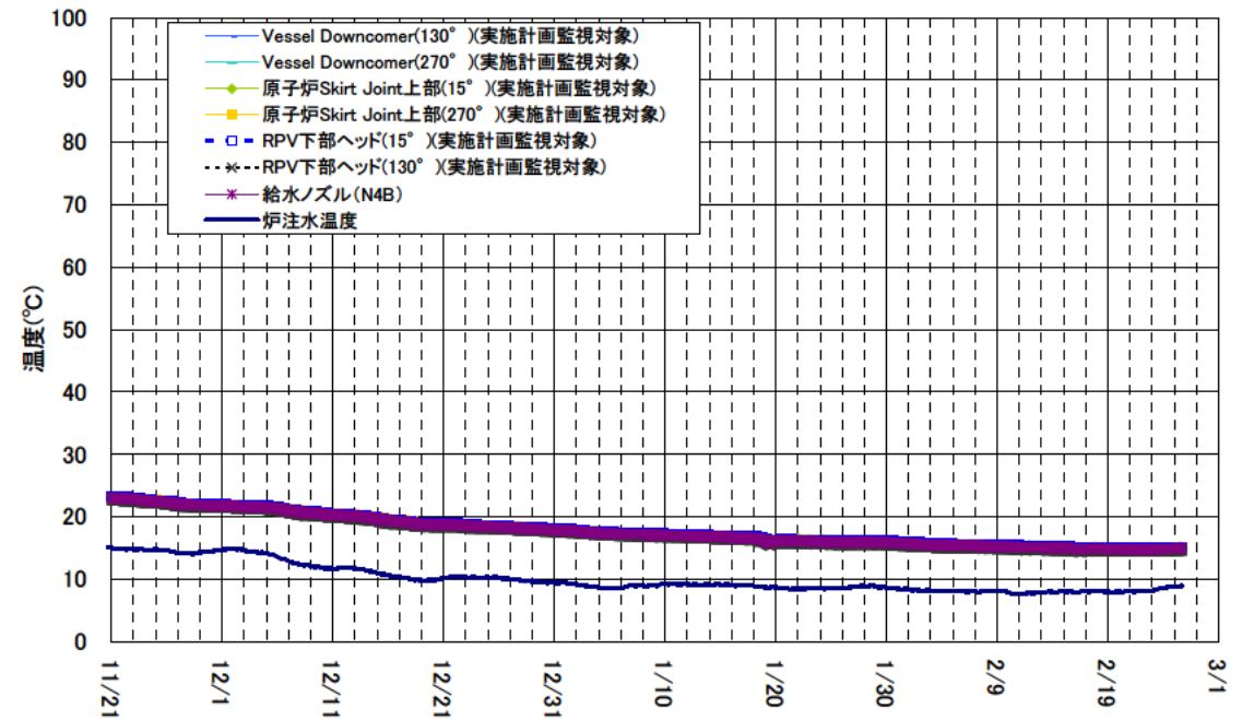
1号機 原子炉圧力容器まわり温度(11/21~2/25)
