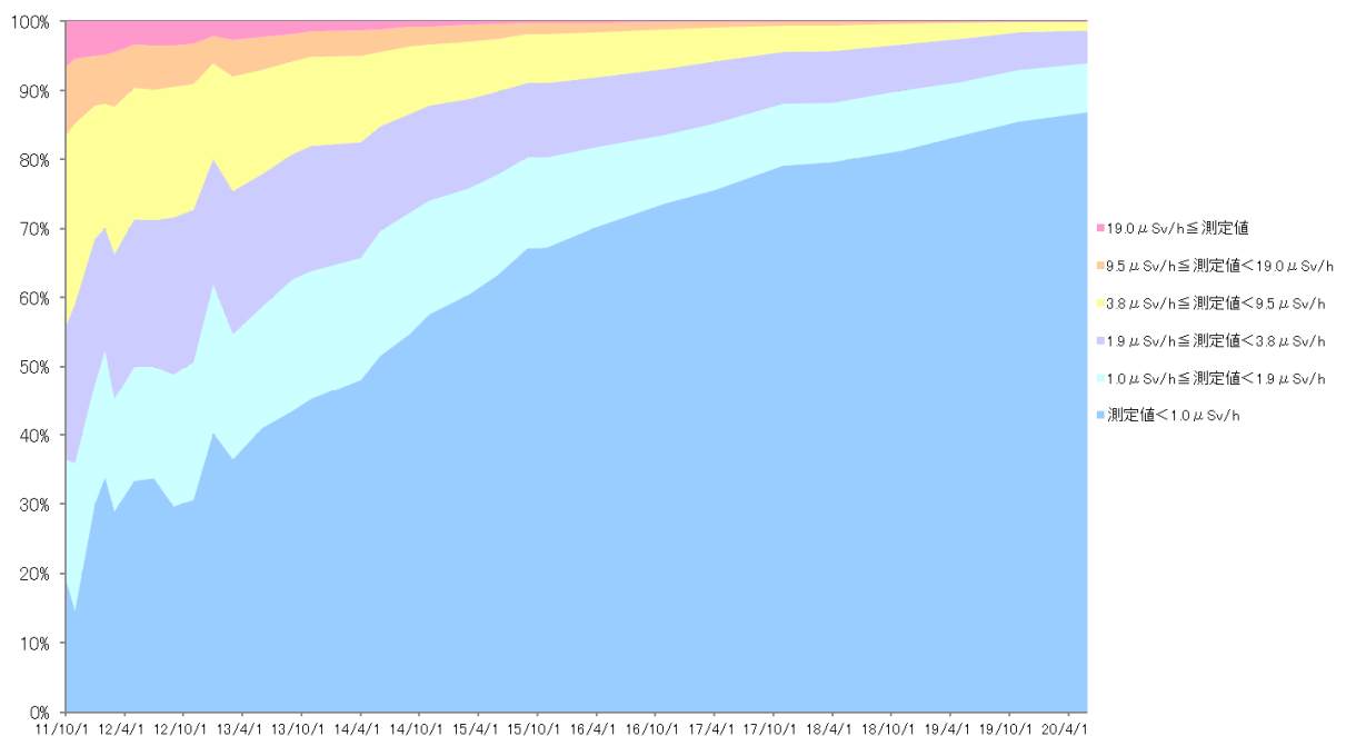
図 1 空間線量率の度数分布の変化
