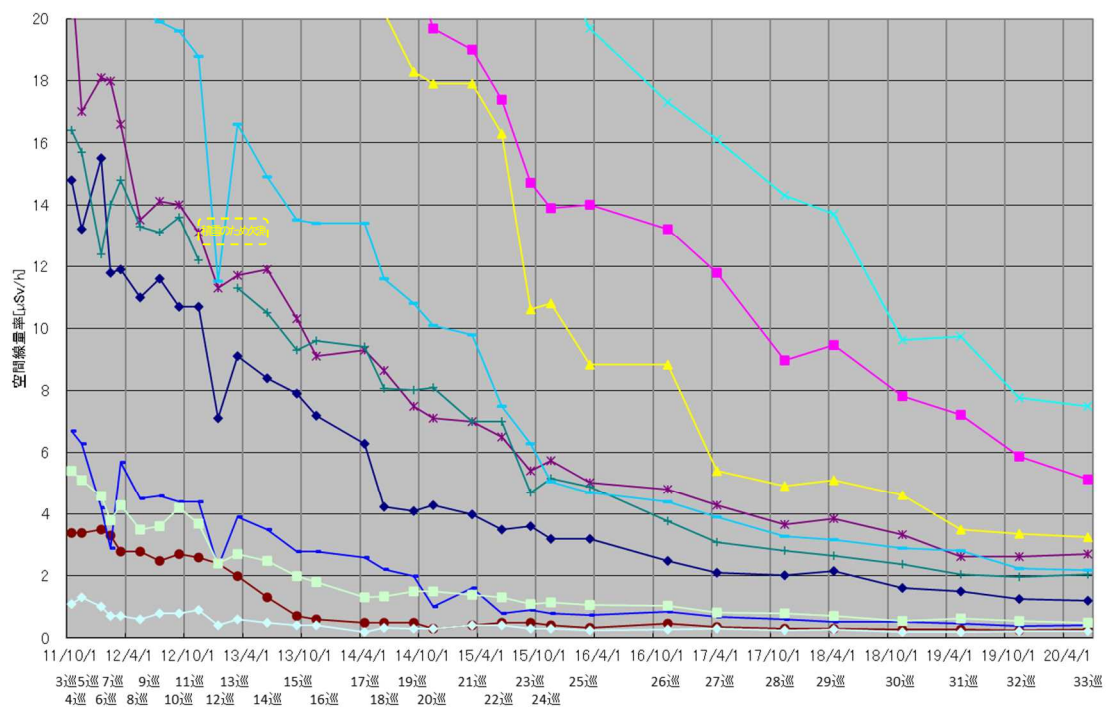
図3 図2のうち20 \mu Sv/h以下の拡大
