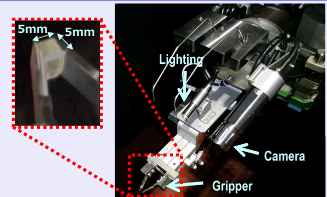
< Gripper-type edge tool >
