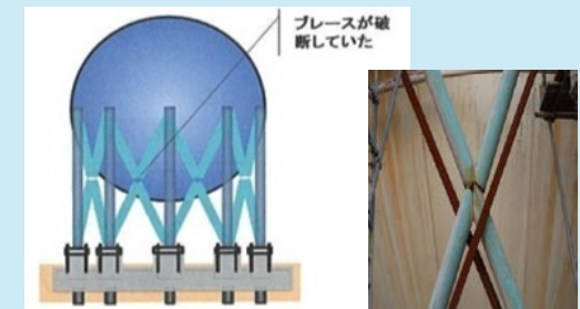
【耐震基準の見直しを実施した球形タンクを支える脚部（ブレース）の補強等対策】
