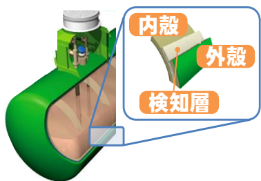
＜地下タンクの入換・大型化＞
