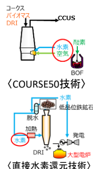
＜直接水素還元技術＞
