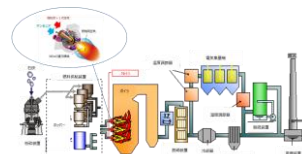
＜混焼バーナーイメージ＞
