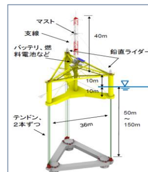
風況観測設備のイメージ
