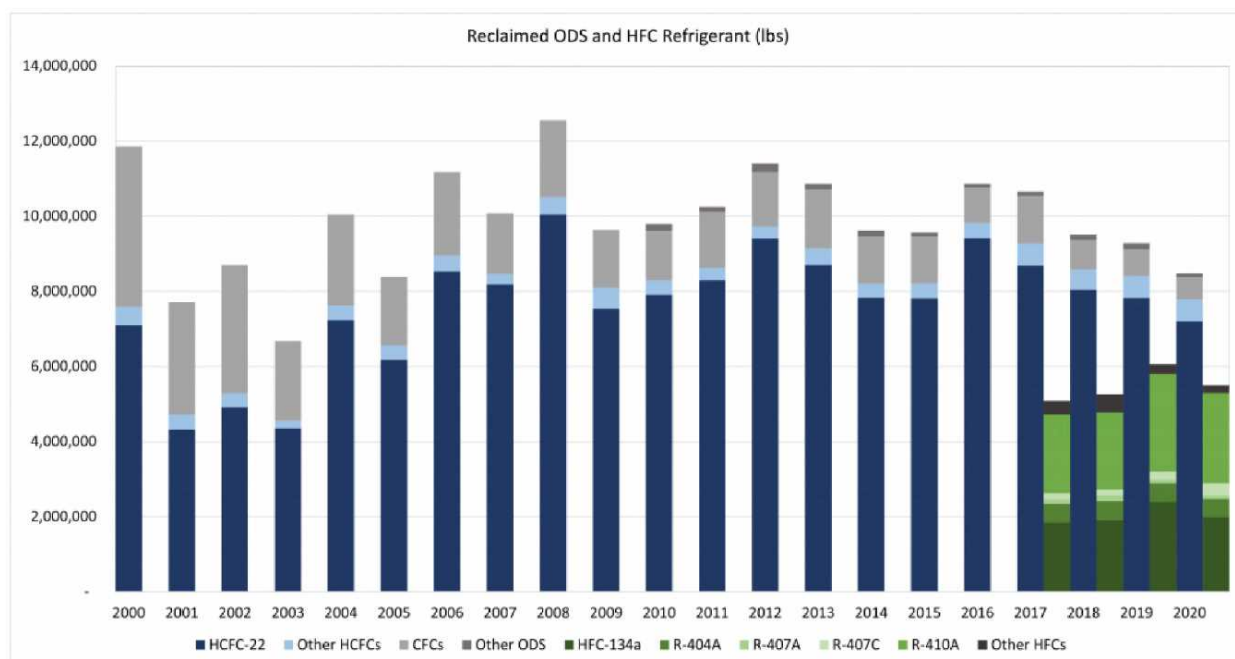
図表 5 再生のために回収された ODS 及び HFC 冷媒の量
