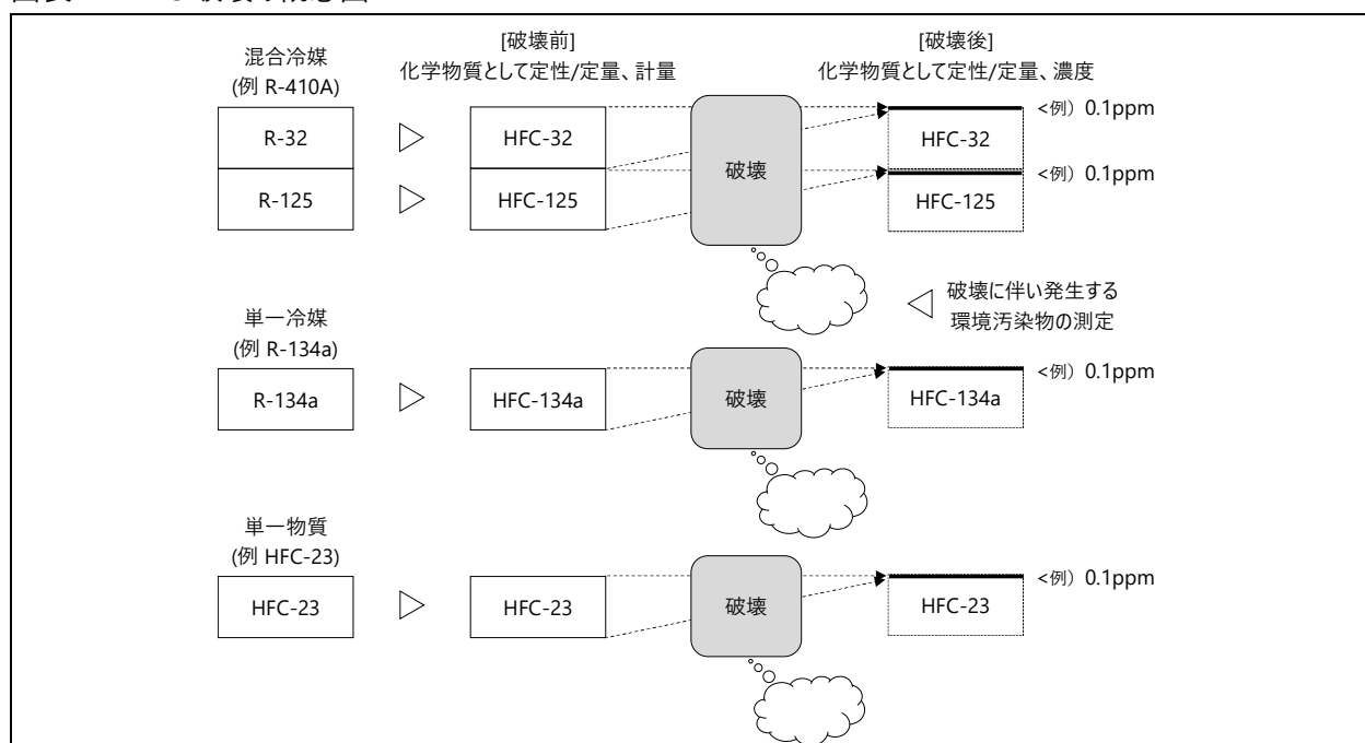
図表 12 HFC 破壊の概念図
