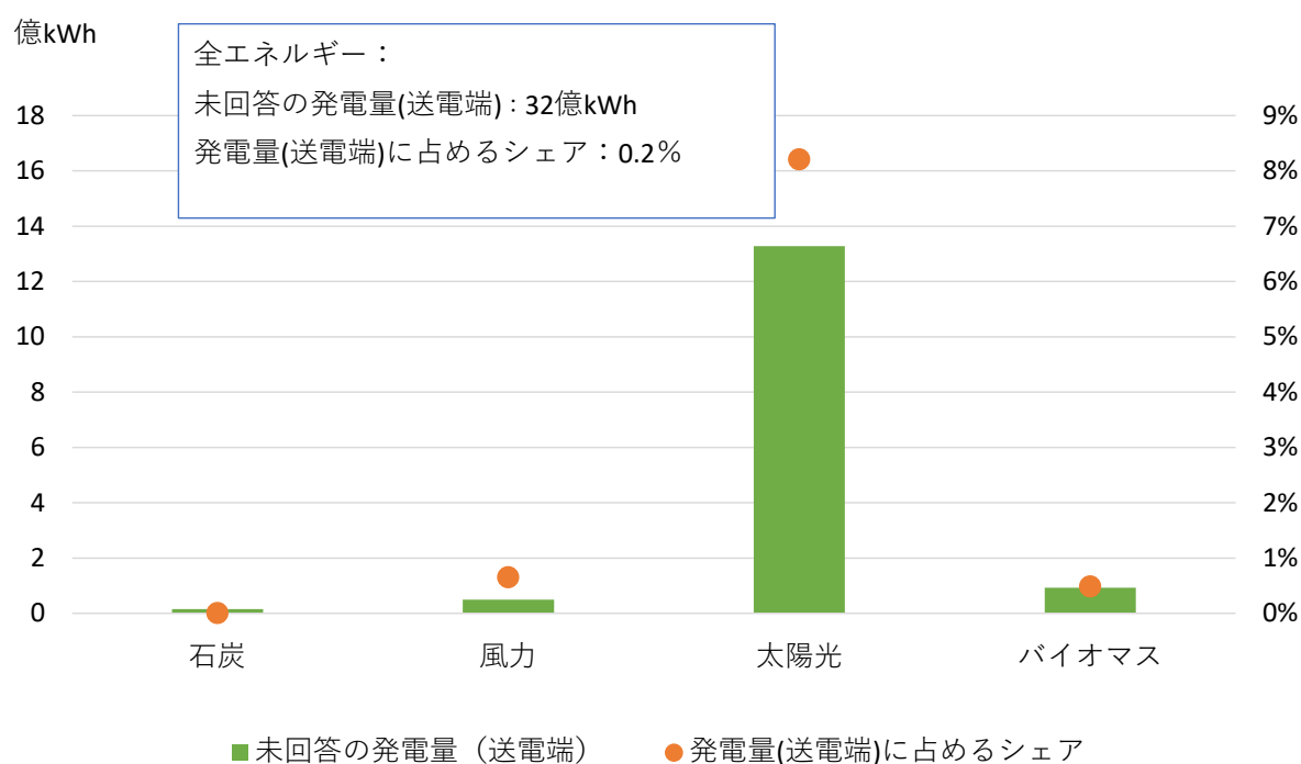
図2.5-1 未回答の事業者の発電量(送電端)と発電量に占めるシェア(2020年度)
