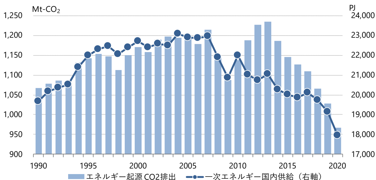
図6.1-1 一次エネルギー国内供給とエネルギー起源CO 2 排出量
