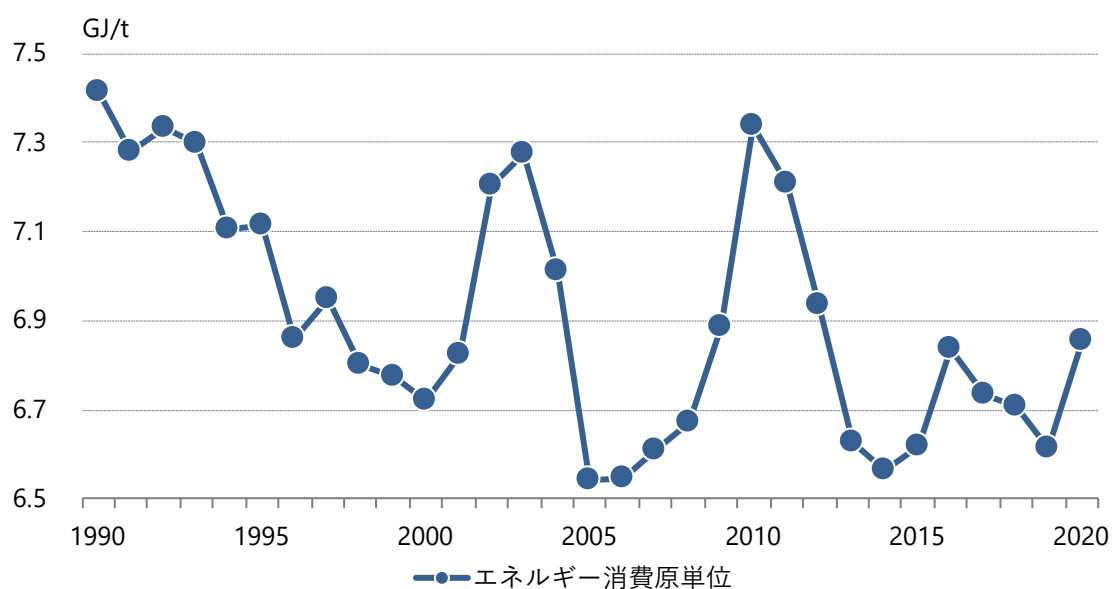
図3.1-37 窯業・土石製品工業のセメント生産量あたりエネルギー消費原単位
