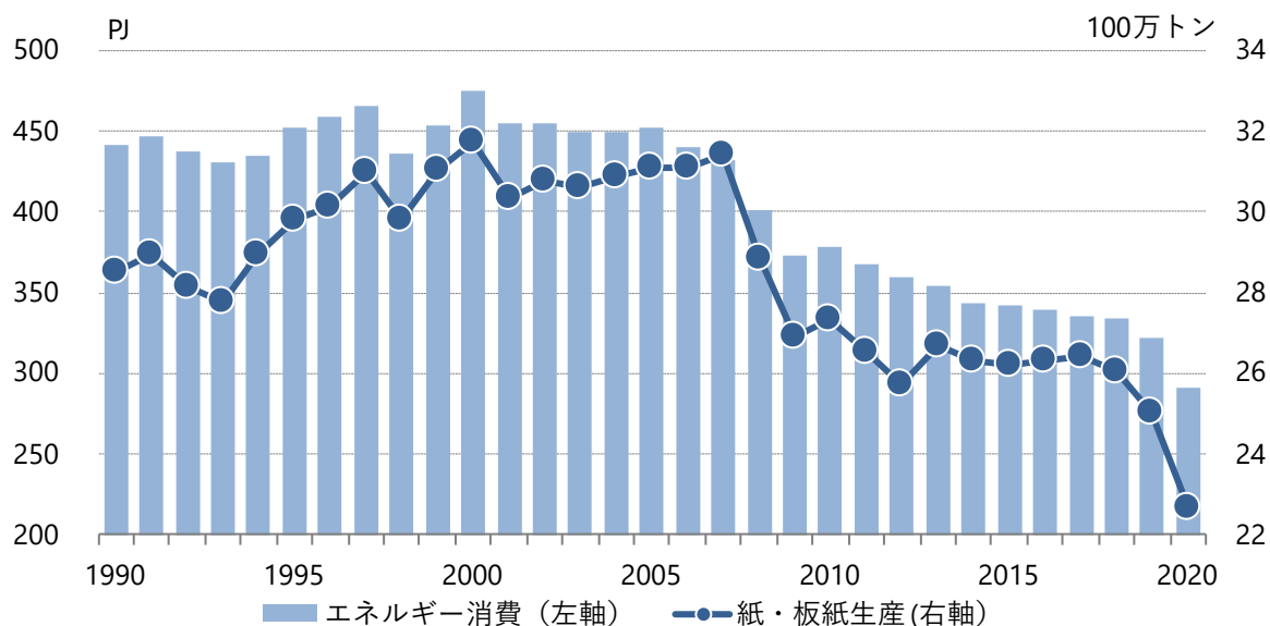
図3.1-28 パルプ・紙・紙加工品工業の最終エネルギー消費と紙・板紙生産量
