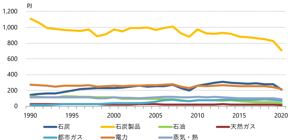
図3.1-14 鉄鋼業の最終エネルギー消費(主要エネルギー源別)
