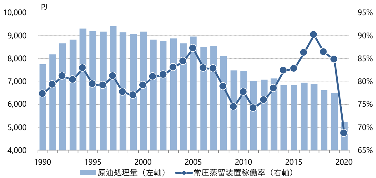
図4.1-1 原油処理量および製油所稼働率
