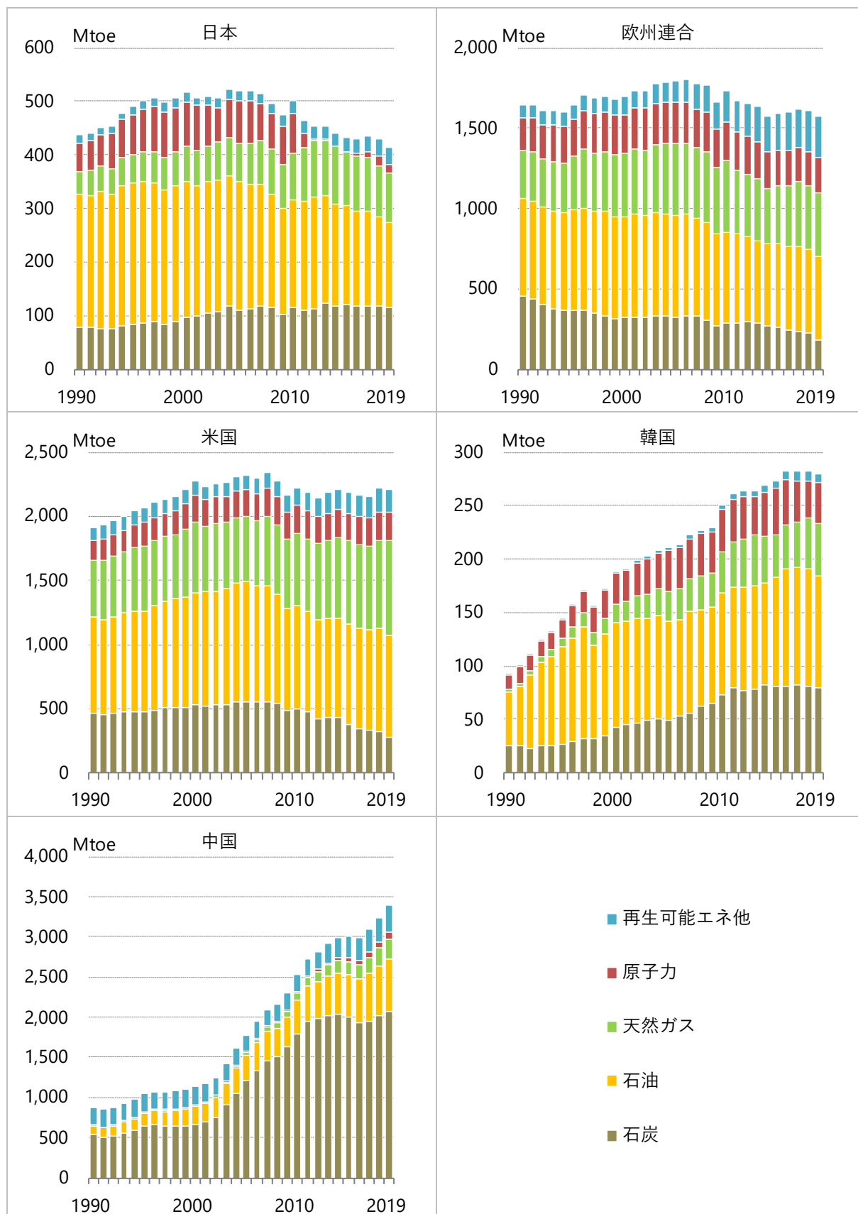
図1.6-1 主要国の一次エネルギー国内供給のエネルギー構成
