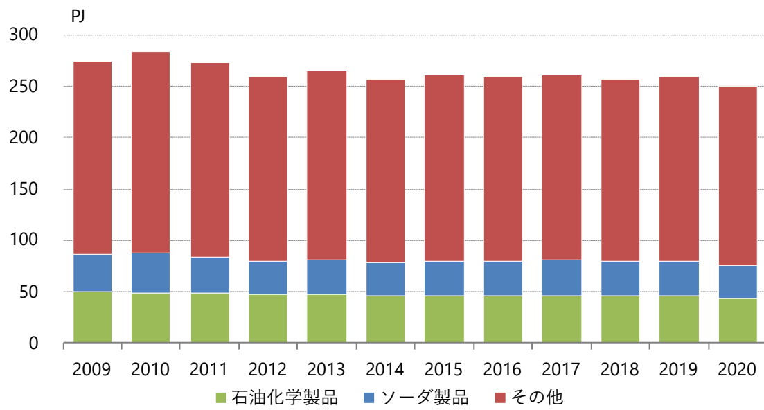
図3.1-26 化学工業の電力消費(製品別)
