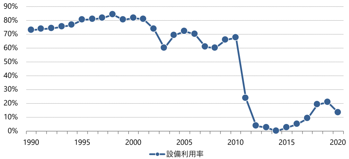
図5.3-8 原子力発電所設備利用率
