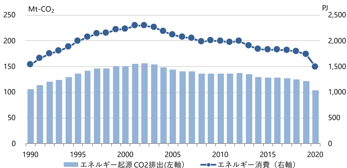
図6.3-13 旅客部門のエネルギー消費量とCO 2 排出量(電力・熱配分後)
