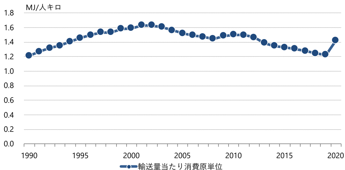
図3.3-6 旅客部門の輸送量あたりエネルギー消費原単位
