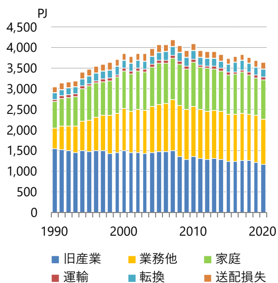
図4.2-1 電力需要(部門別)
