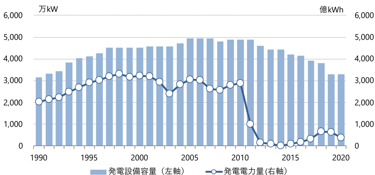
図5.3-7 原子力発電設備容量(年度末)と発電電力量
