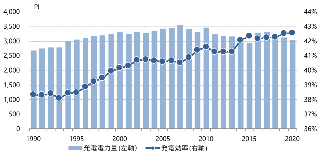
図4.2-7 事業用発電電力量と発電効率
