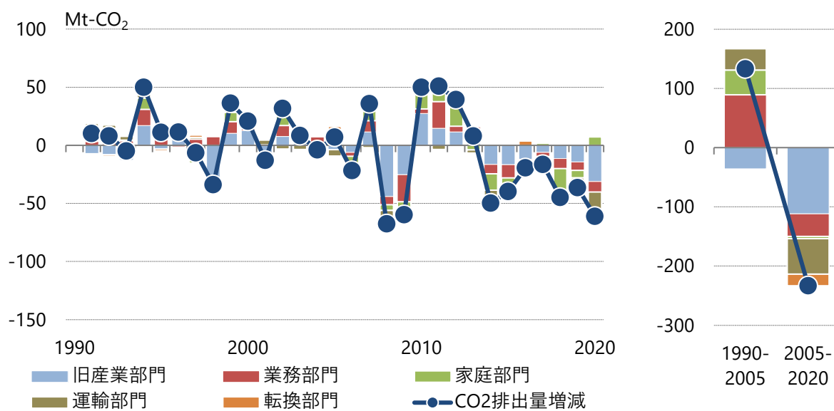
図6.2-2 エネルギー起源CO 2 排出量の部門別要因分解
