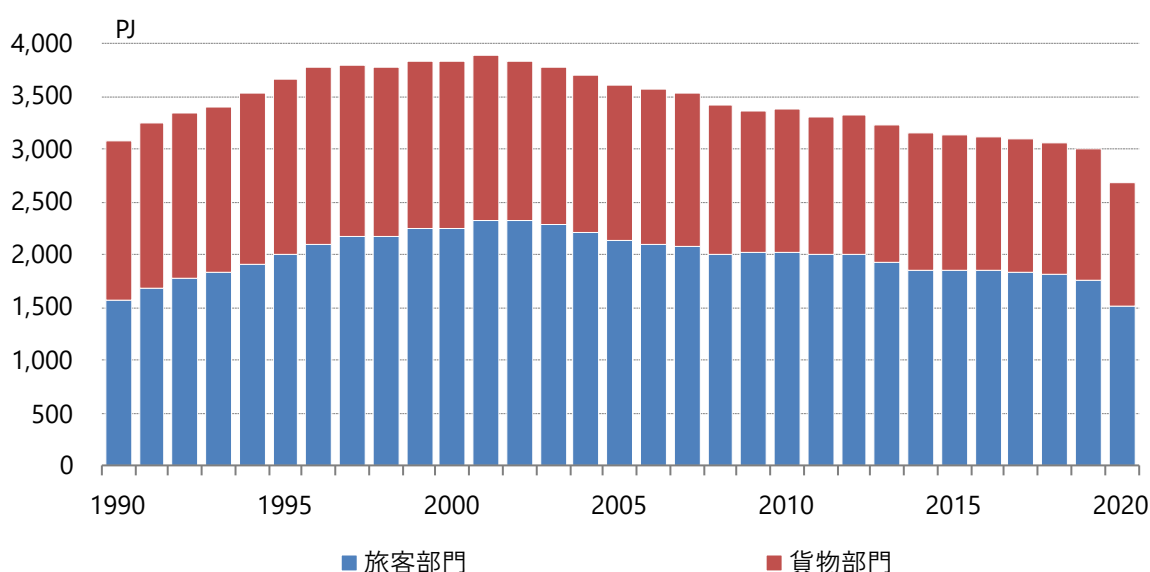
図3.3-1 運輸部門の最終エネルギー消費
