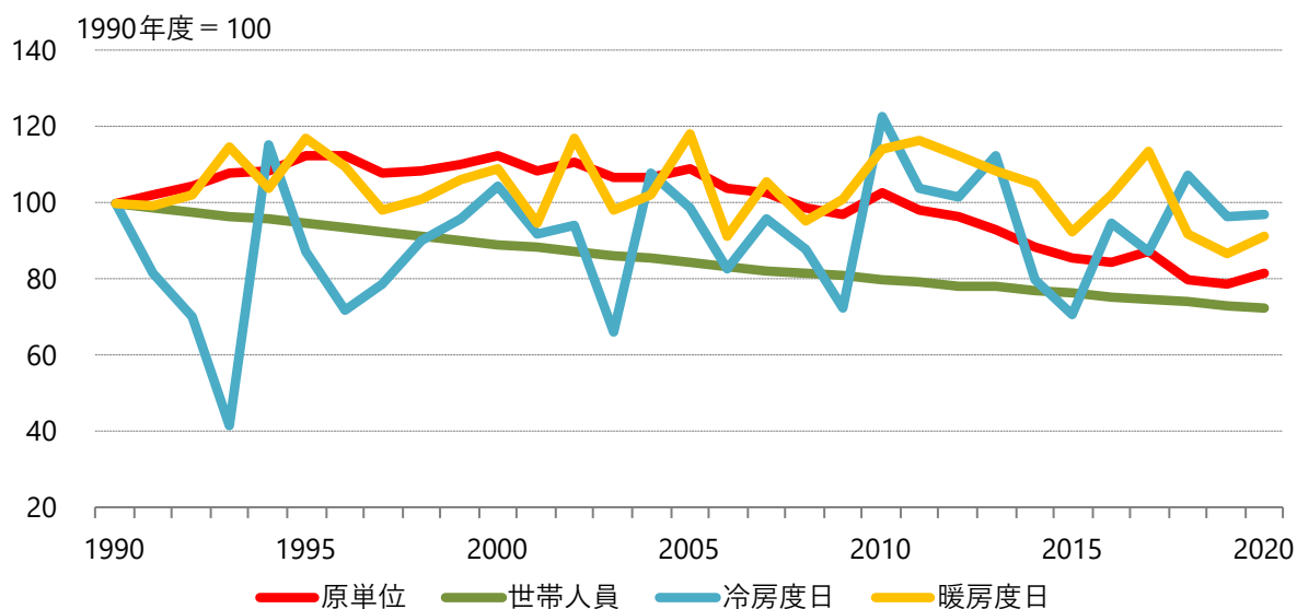
図3.2-7 家庭部門のエネルギー消費原単位の関連指標
