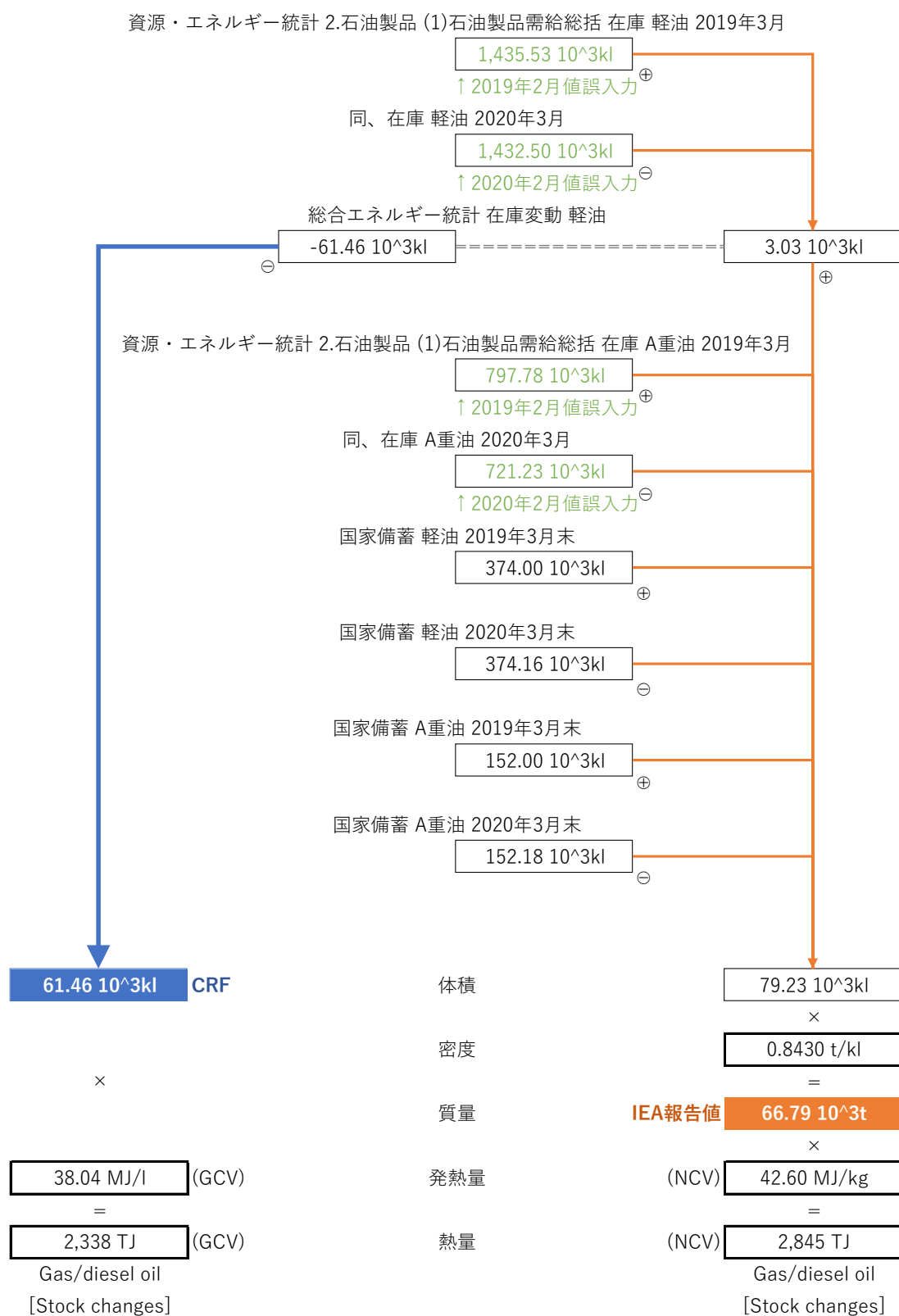
図9.2-11 Gas/diesel oilの在庫変動量(2019年度)
