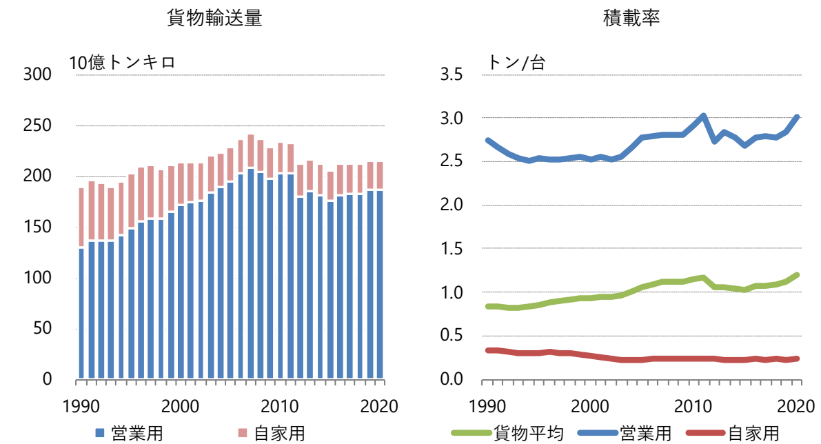
図3.3-20 自家用・営業用別の貨物輸送量と積載率
