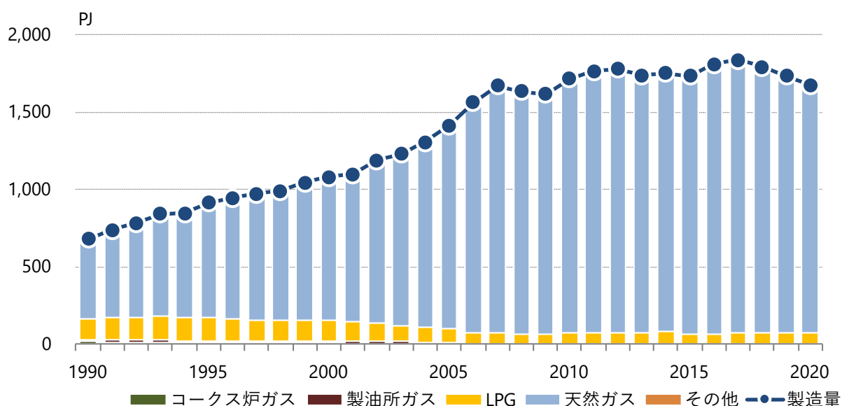
図4.3-2 都市ガス製造量と原料投入量
