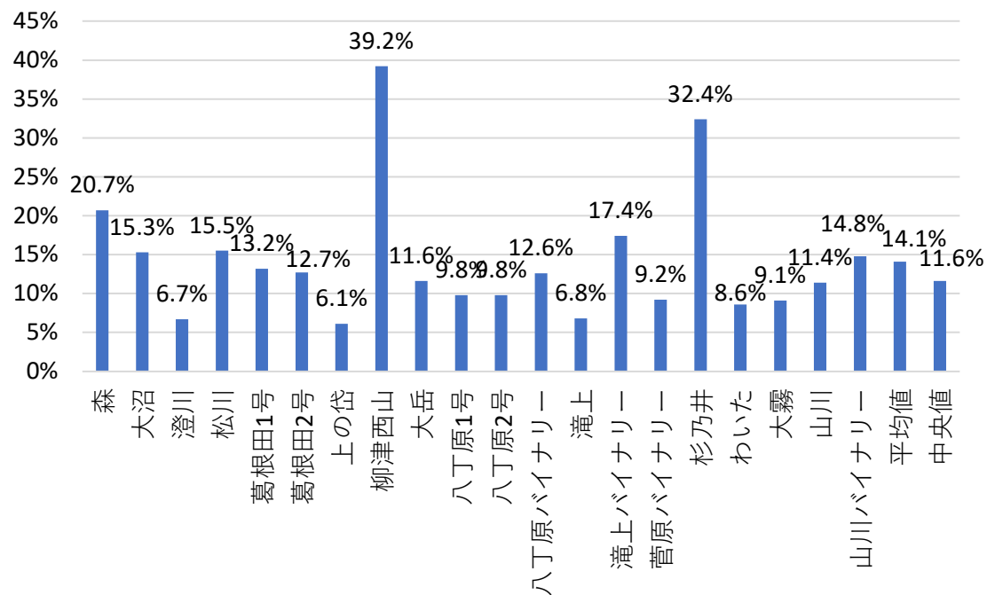
図2.7-5 1,000kW以上の地熱発電所の所内率(2019年度)
