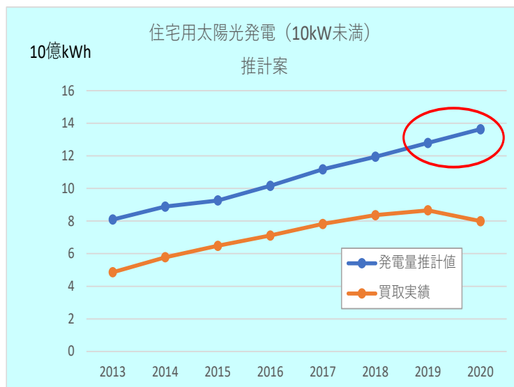
図5.1-1 住宅太陽光発電量の推計値
