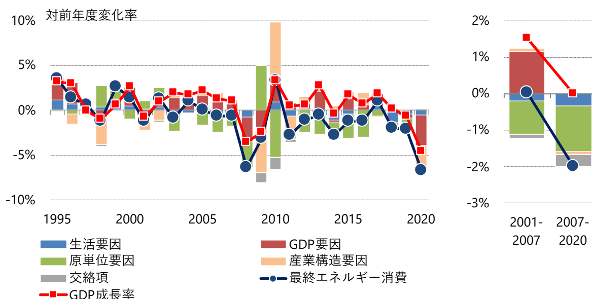
図1.4-2 最終エネルギー消費変化率の要因分解(寄与度)
