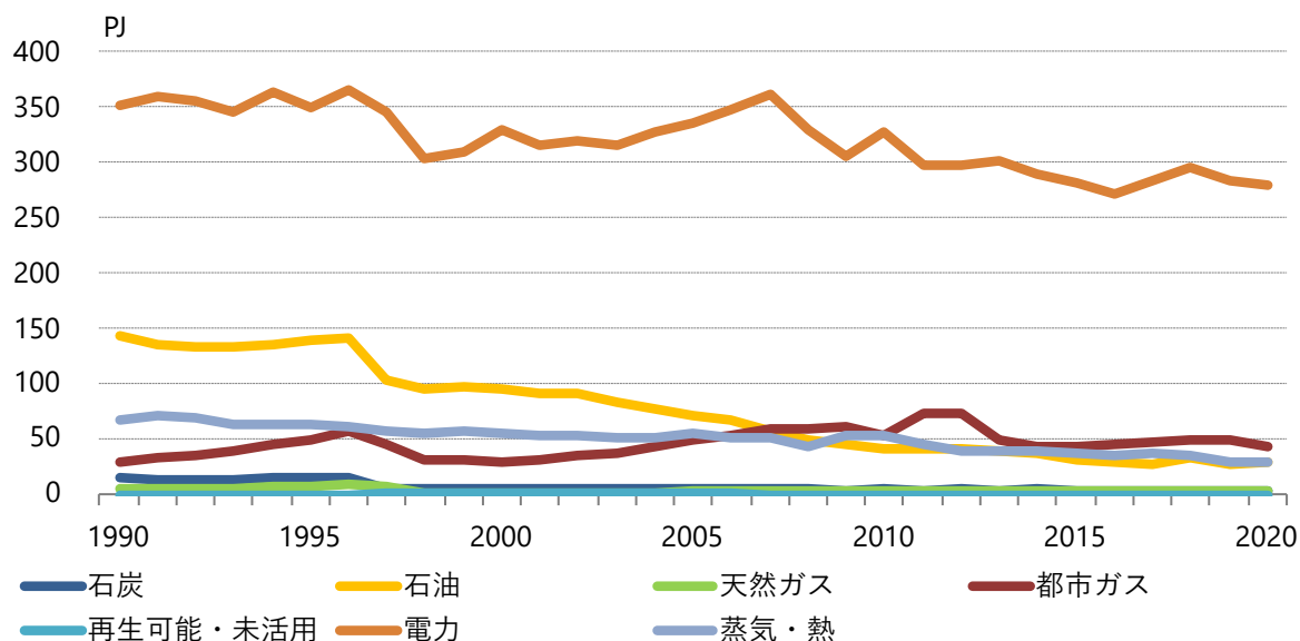
図3.1-46 機械工業の最終エネルギー消費(エネルギー源別)
