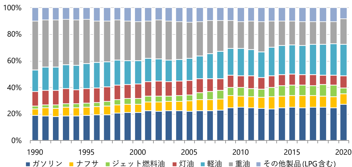
図4.1-5 石油製品の生産得率(製品別構成比)
