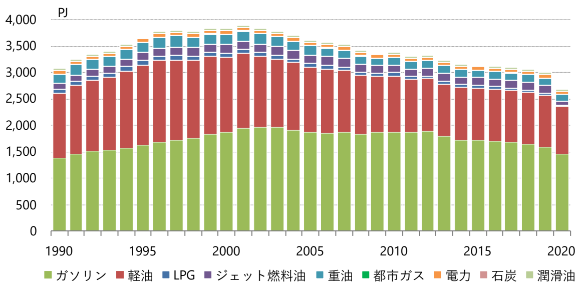
図3.3-3 運輸部門の最終エネルギー消費(エネルギー源別)
