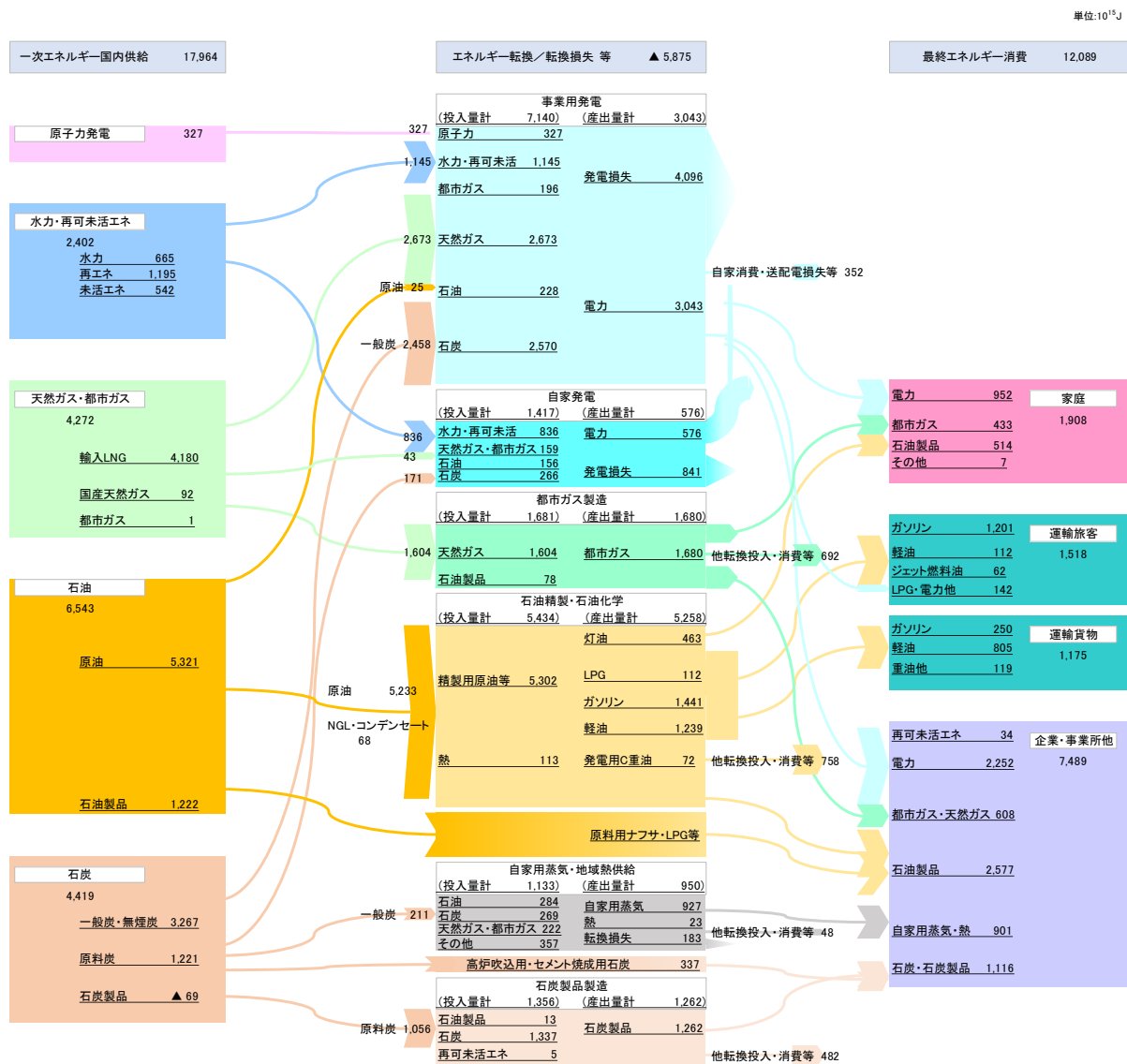
図10.6-1 わが国のエネルギーバランス・フロー概要
