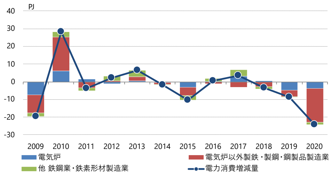
図3.1-16 鉄鋼業の電力消費増減(前年度比)
