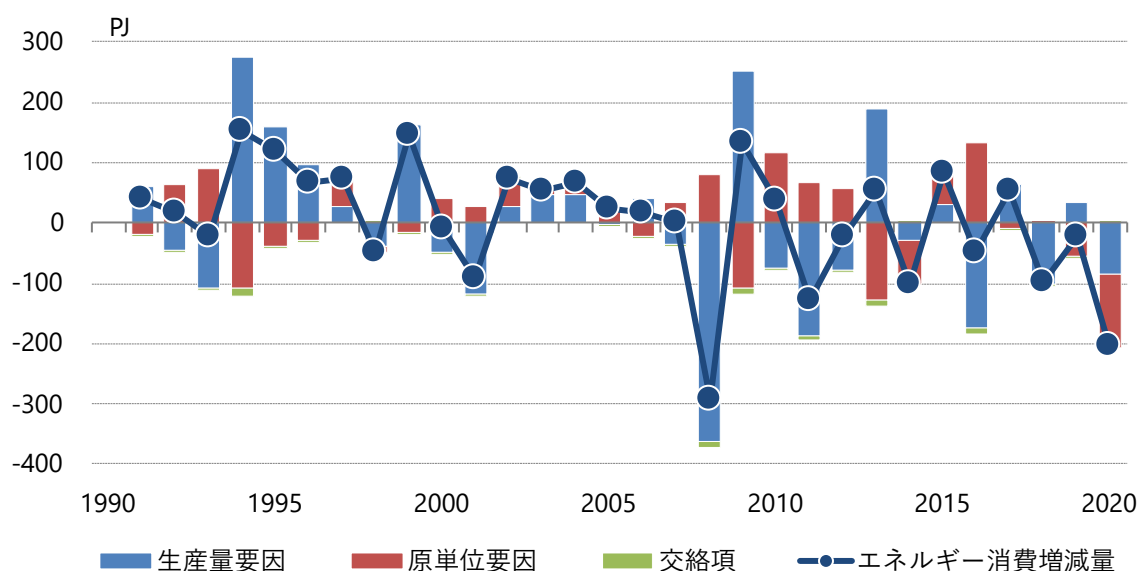
図3.1-22 化学工業の最終エネルギー消費の要因分解(前年度比)
