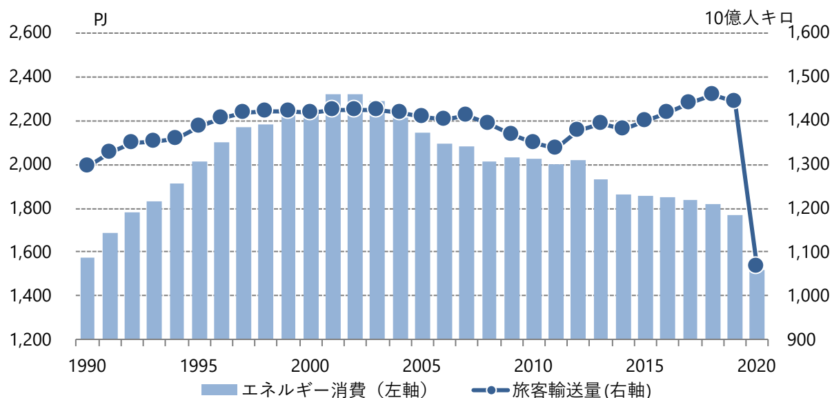
図3.3-4 旅客部門の最終エネルギー消費と旅客輸送量(人キロ)
