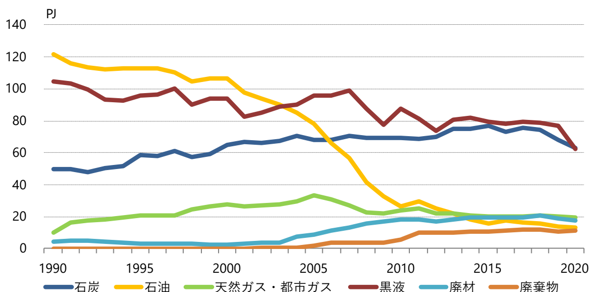
図3.1-32 パルプ・紙・紙加工品工業の自家用蒸気のエネルギー投入(エネルギー源別)
