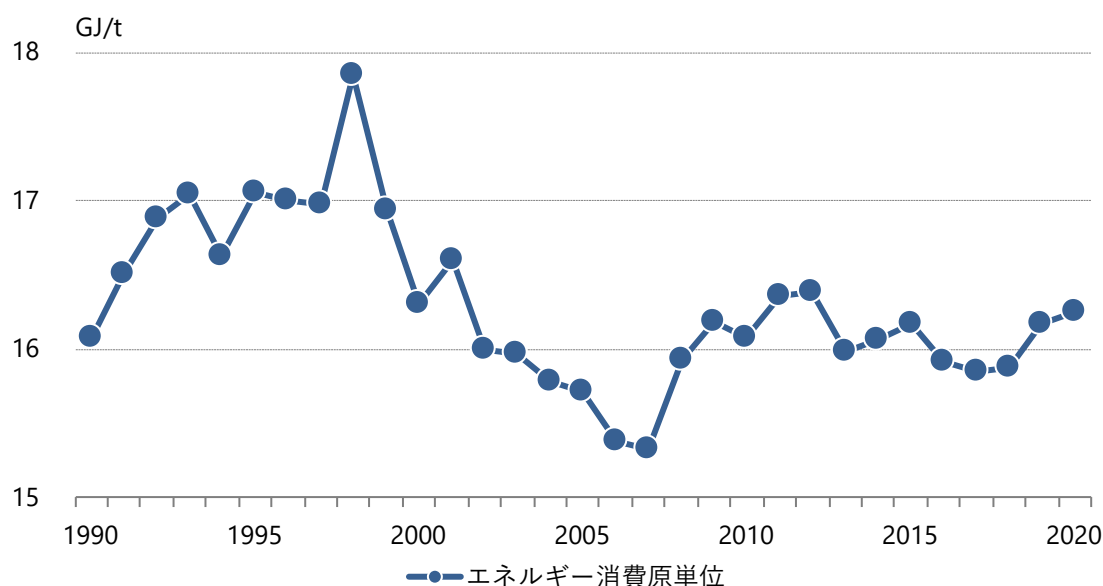
図3.1-12 鉄鋼業の粗鋼生産量あたりエネルギー消費原単位
