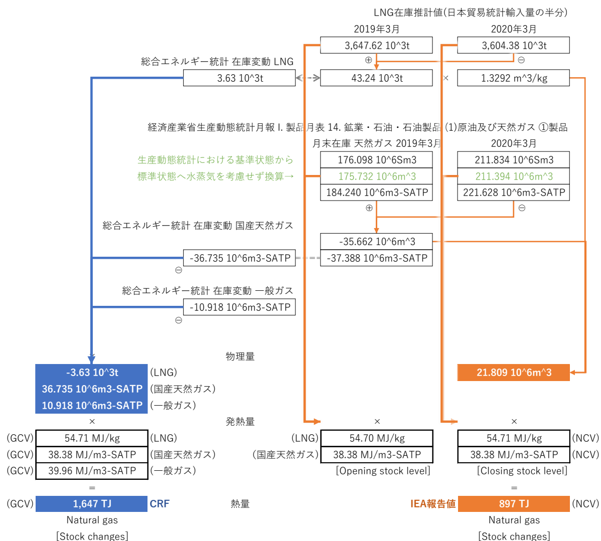
図9.2-19 天然ガスの在庫変動量(2019年度)
