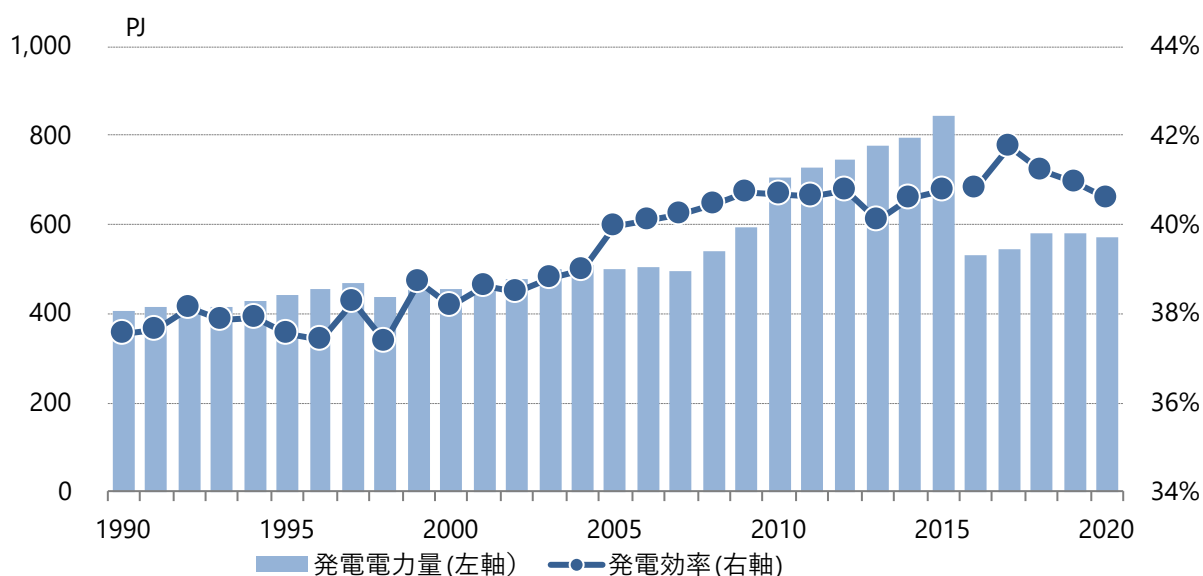
図4.2-9 自家用発電電力量と発電効率
