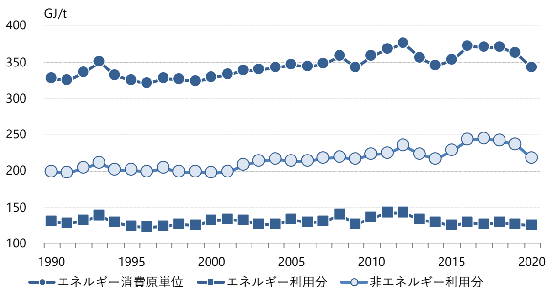
図3.1-19 化学工業のエチレン生産量あたりエネルギー消費原単位
