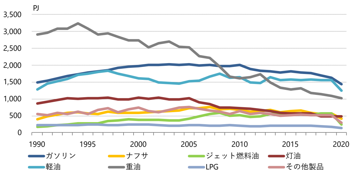
図4.1-4 石油製品別生産量
