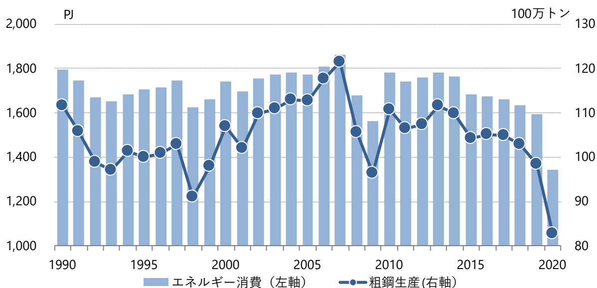
図3.1-11 鉄鋼業の最終エネルギー消費と粗鋼生産量
