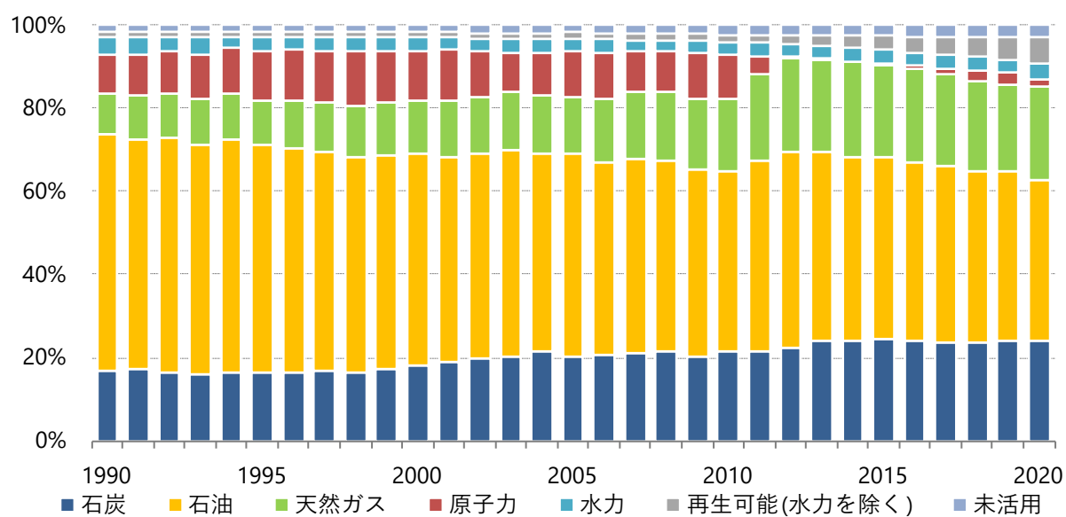
図5.4-4 一次エネルギー総供給(エネルギー源別構成比)
