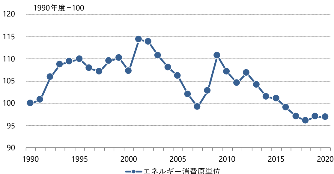
図3.1-4 製造業の生産指数あたりエネルギー消費原単位
