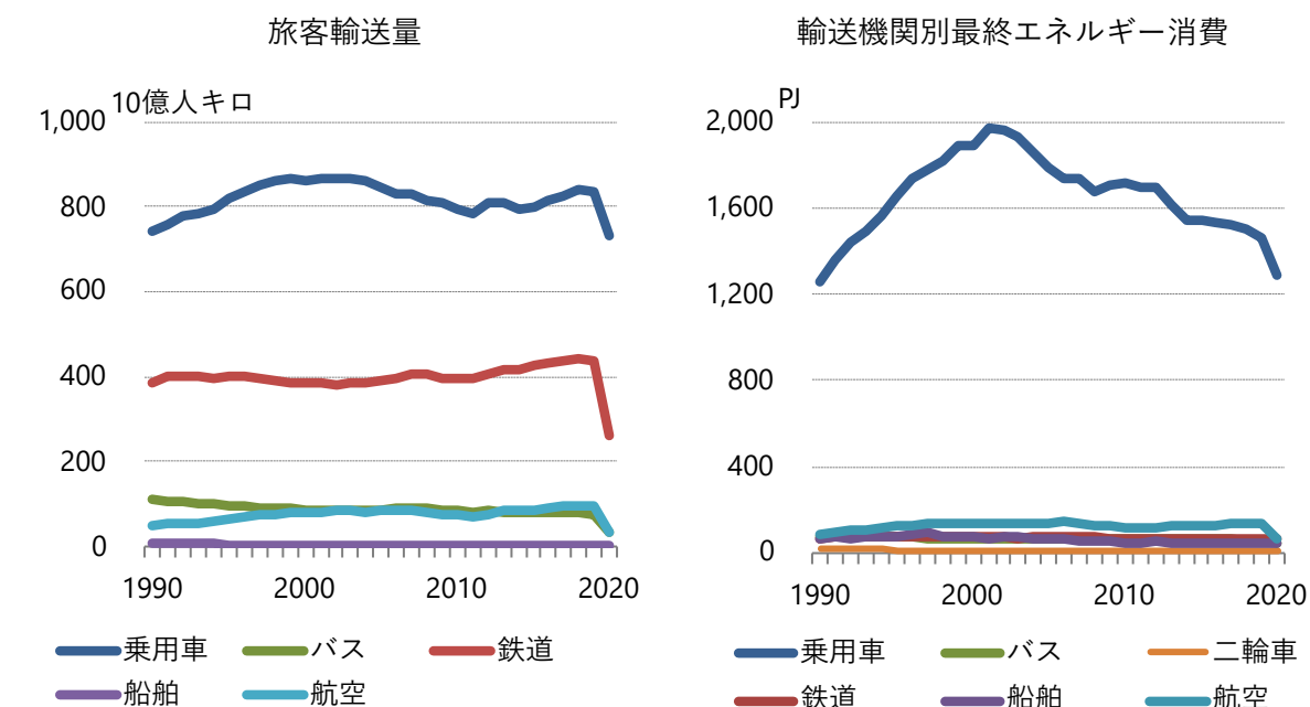
図3.3-7 旅客部門の旅客輸送量と最終エネルギー消費
