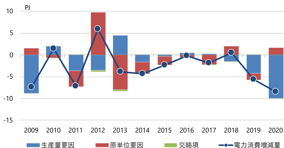
図3.1-33 パルプ・紙・紙加工品工業の電力消費の要因分解(前年度比)
