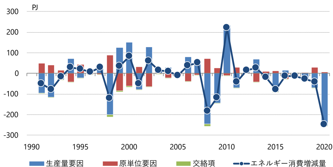
図3.1-13 鉄鋼業の最終エネルギー消費の要因分解(前年度比)
