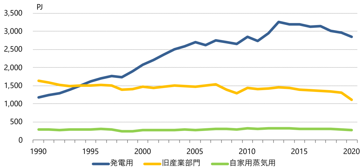
図5.3-4 石炭の国内需要
