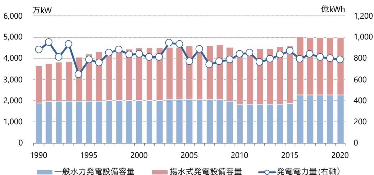
図5.3-9 水力発電設備容量(年度末)と発電電力量
