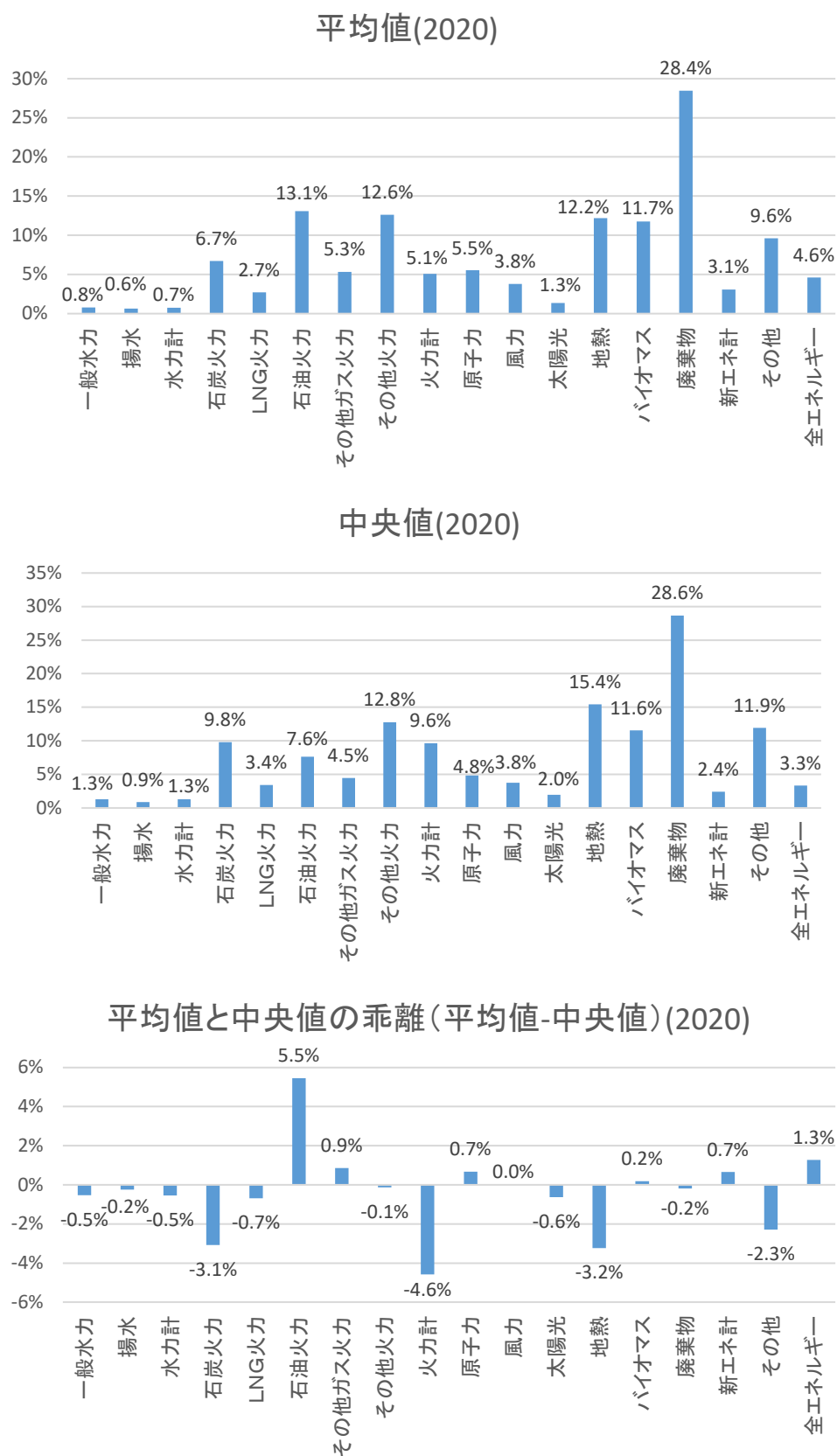
図2.4-1 各電源の2020年度の所内率の平均値と中央値(外れ値補正前)
