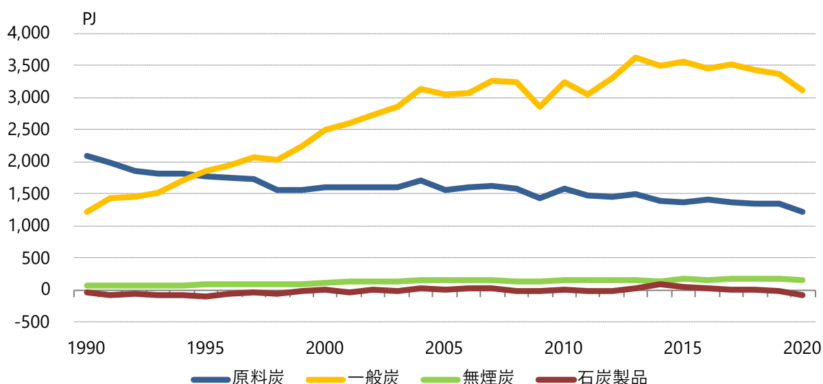
図5.3-3 石炭の国内供給
