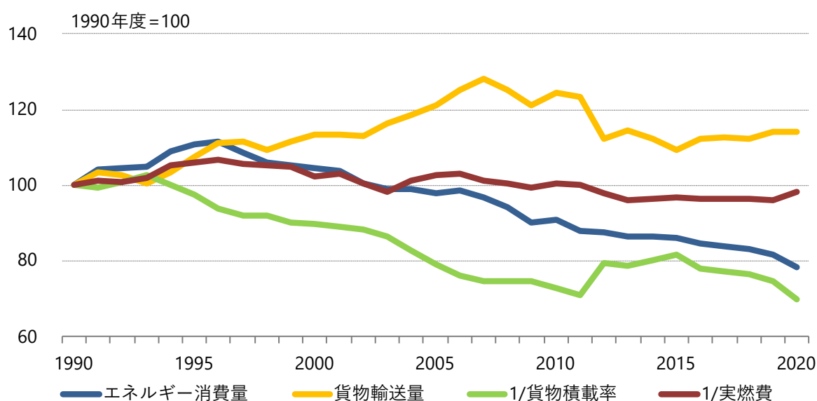
図3.3-19 貨物自動車燃料消費の関連指標
