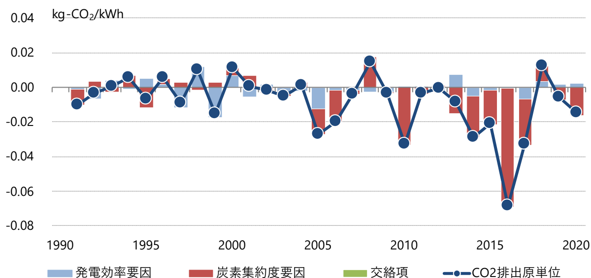
図6.3-24 自家用発電のCO 2 排出原単位(発電端)の要因分解(前年度比)
