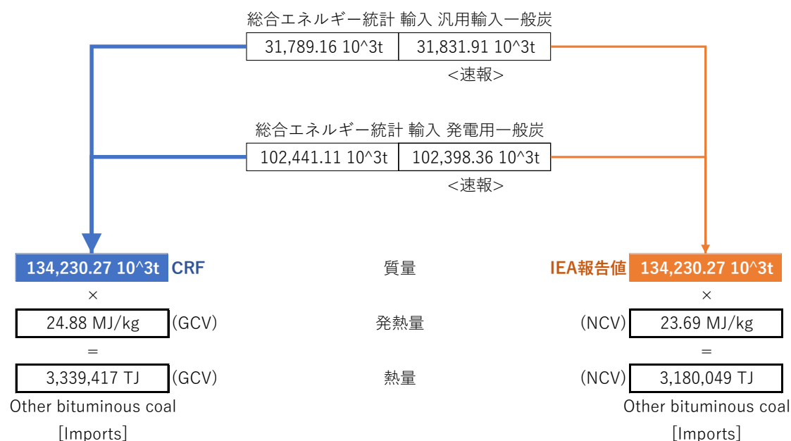
図9.2-5 一般炭輸入量の差異(2019年度)
