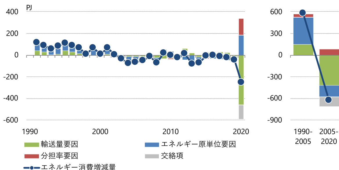
図3.3-8 旅客部門(除自動二輪車)の最終エネルギー消費の要因分解(前年度比)
