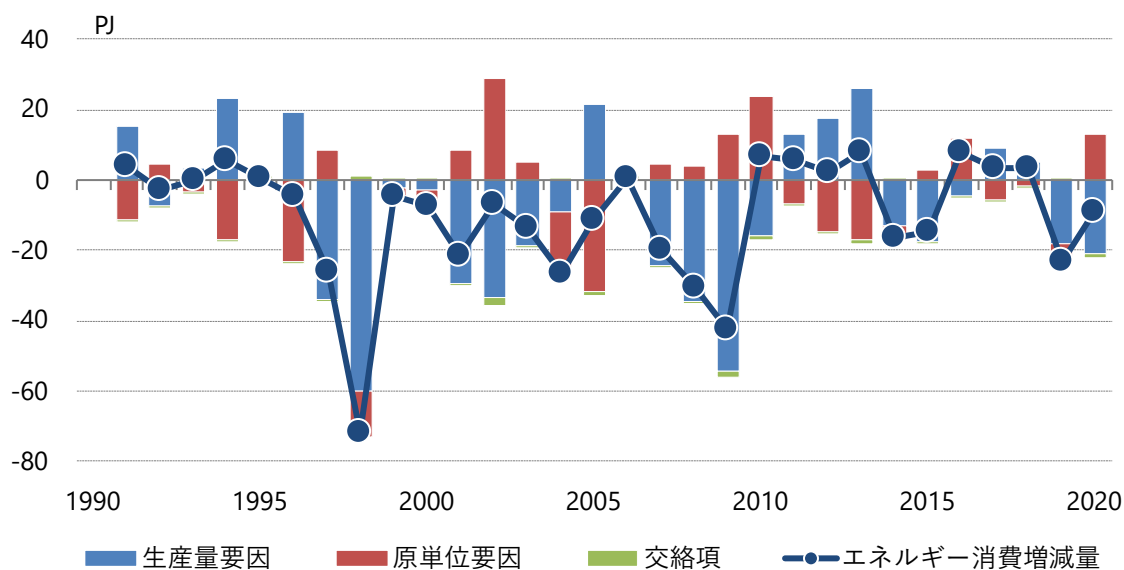
図3.1-38 窯業・土石製品工業の最終エネルギー消費の要因分解(前年度比)
