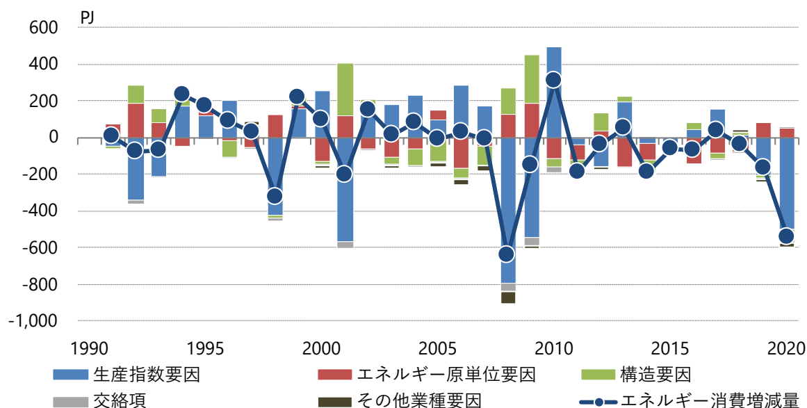
図3.1-5 製造業の最終エネルギー消費の要因分解(前年度比)
