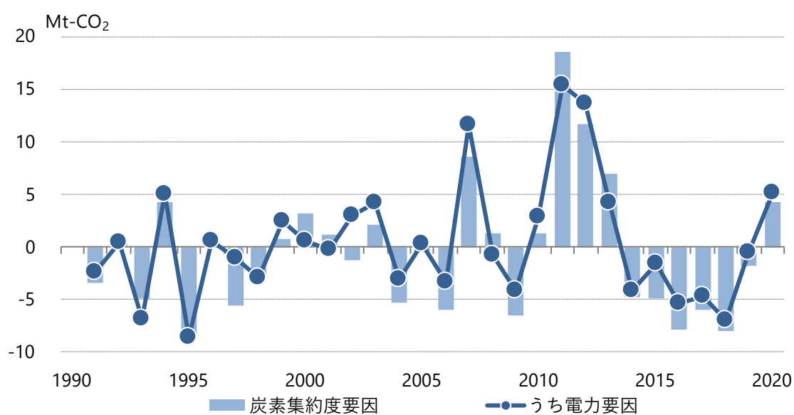
図6.3-4 旧産業部門の炭素集約度要因の分解(前年度比)
