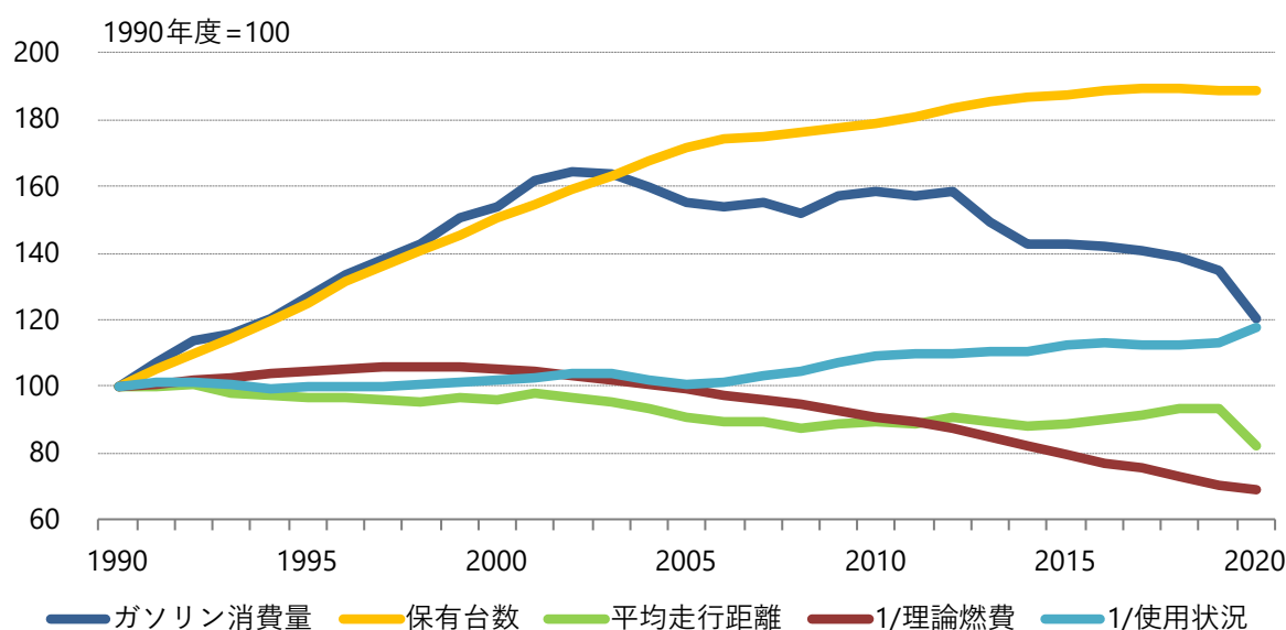
図3.3-11 乗用車ガソリン消費の関連指標
