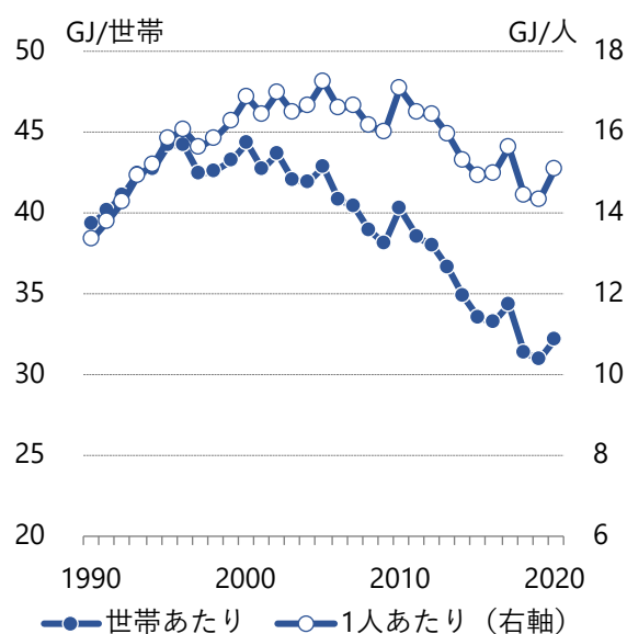
図3.2-2 家庭部門の世帯あたり・1人あたり最終エネルギー消費原単位
