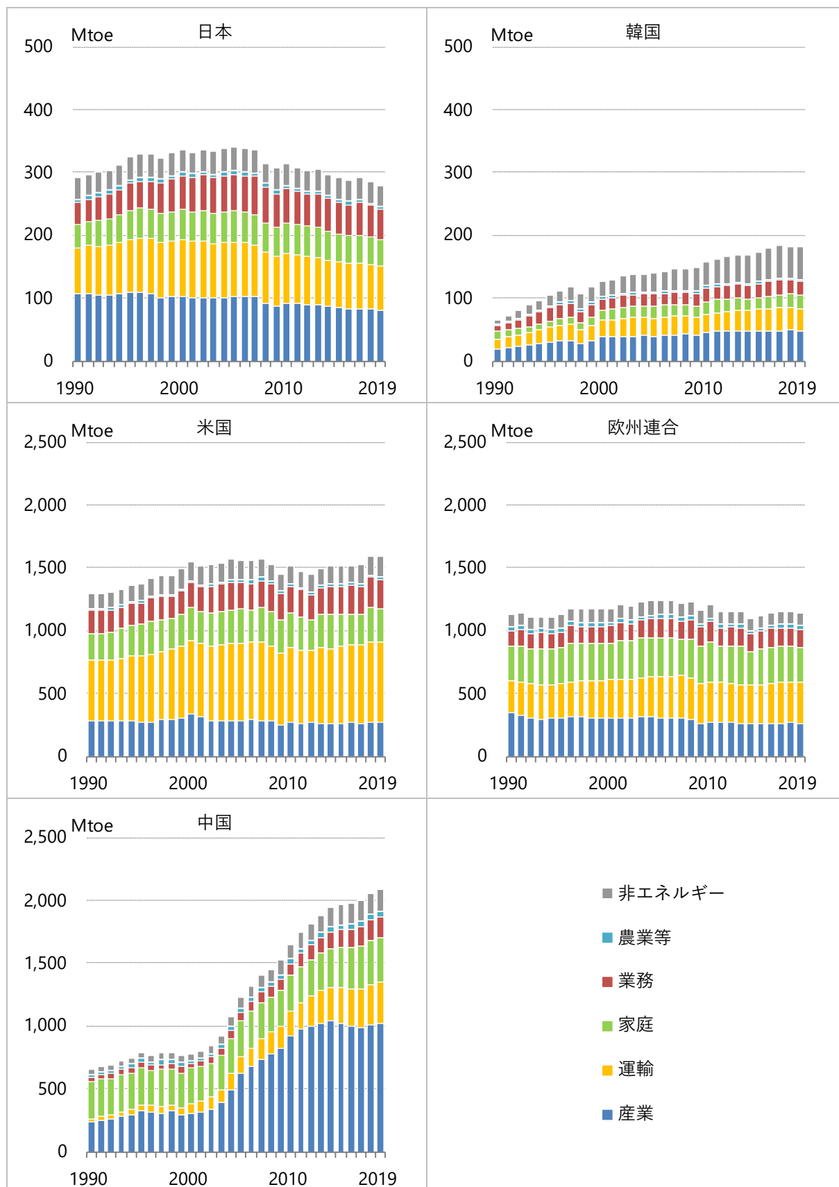
図2.2-3 主要国の最終エネルギー消費の部門構成
