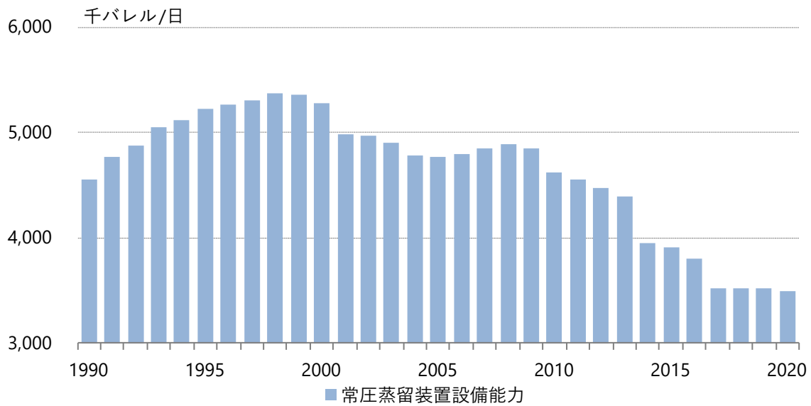
図4.1-2 常圧蒸留装置設備能力
