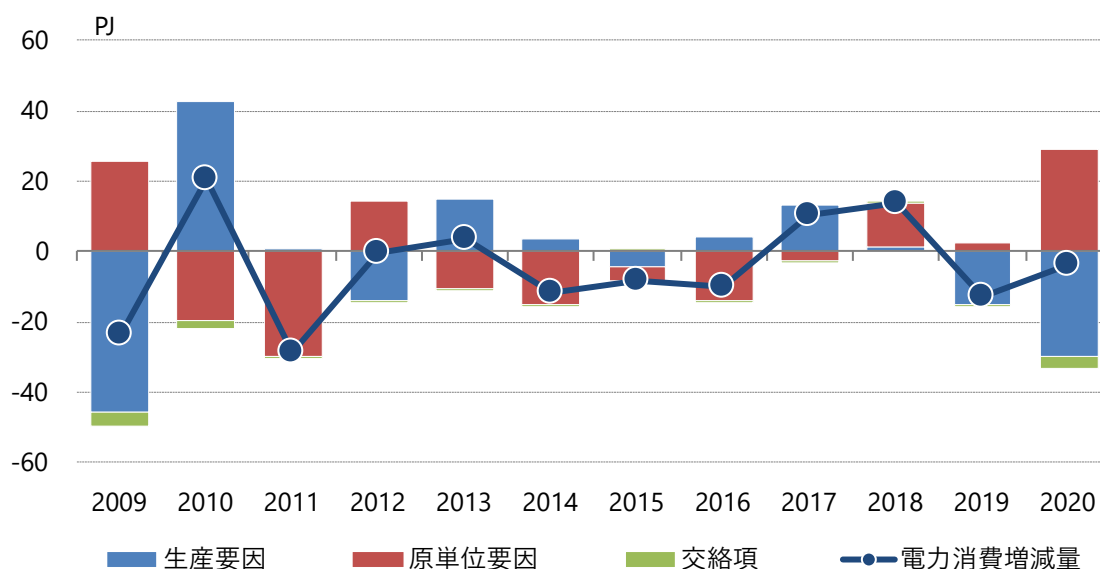
図3.1-47 機械工業の電力消費の要因分解(前年度比)
