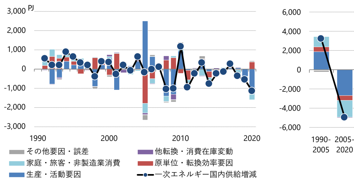
図5.2-1 一次エネルギー国内供給増減の要因別寄与
