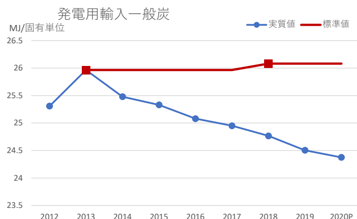
図4.2-1 発電用輸入一般炭の標準、実質発熱量比較
