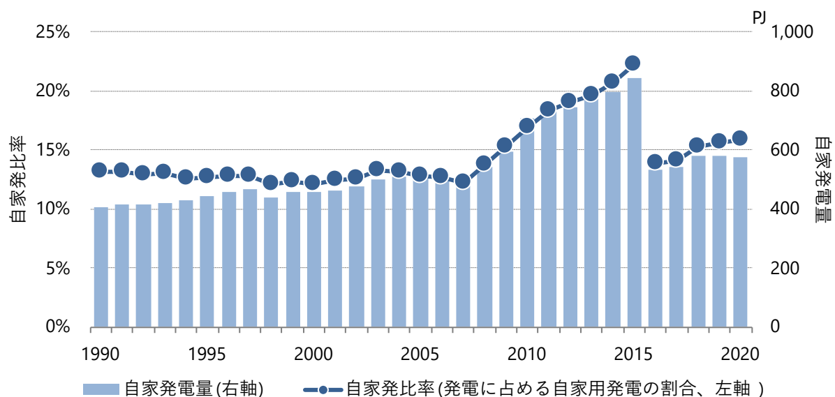
図4.2-6 自家発比率(全発電量に占める自家用発電量の比率)
