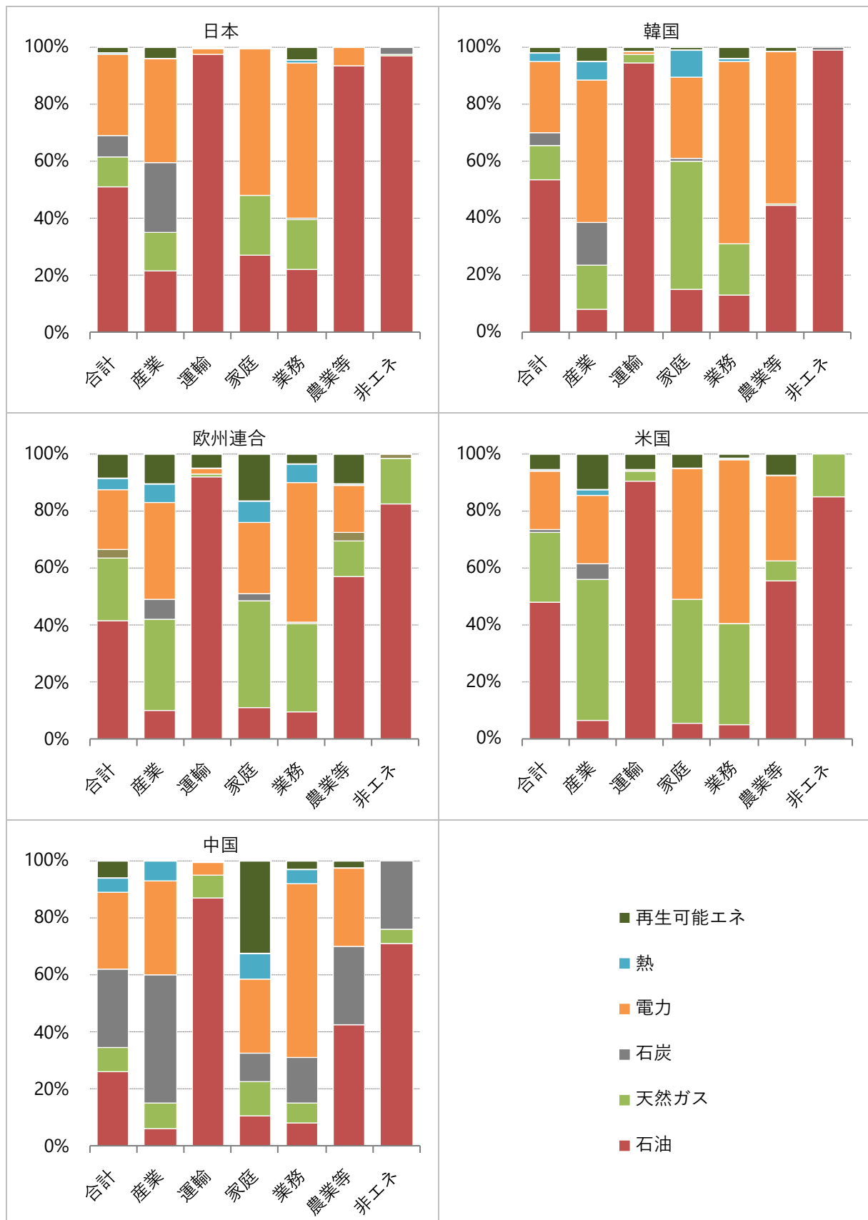
図2.4-1 主要国の部門別エネルギー源別構成比(2019年)
