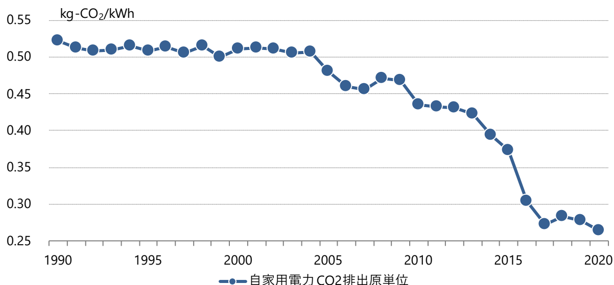
図6.3-23 自家用電力のCO 2 排出原単位(発電端)
