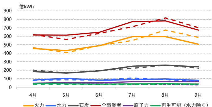
図4.2-12 発電電力量の電源構成(2021年度上期)
