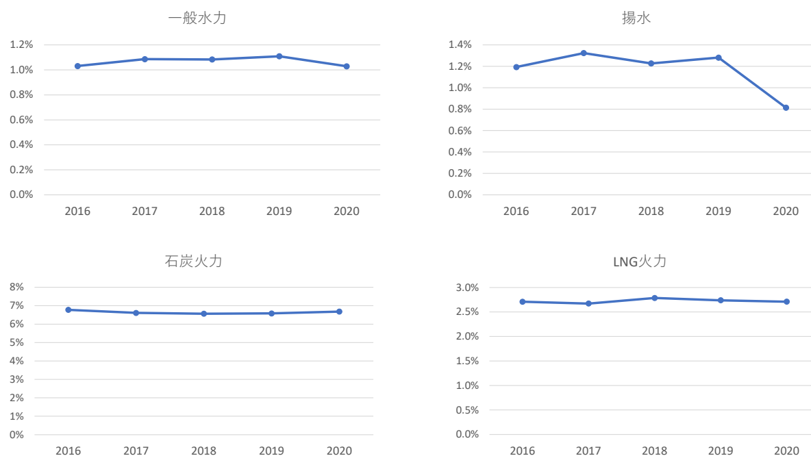
図2.4-5 電源種別所内率の推移
