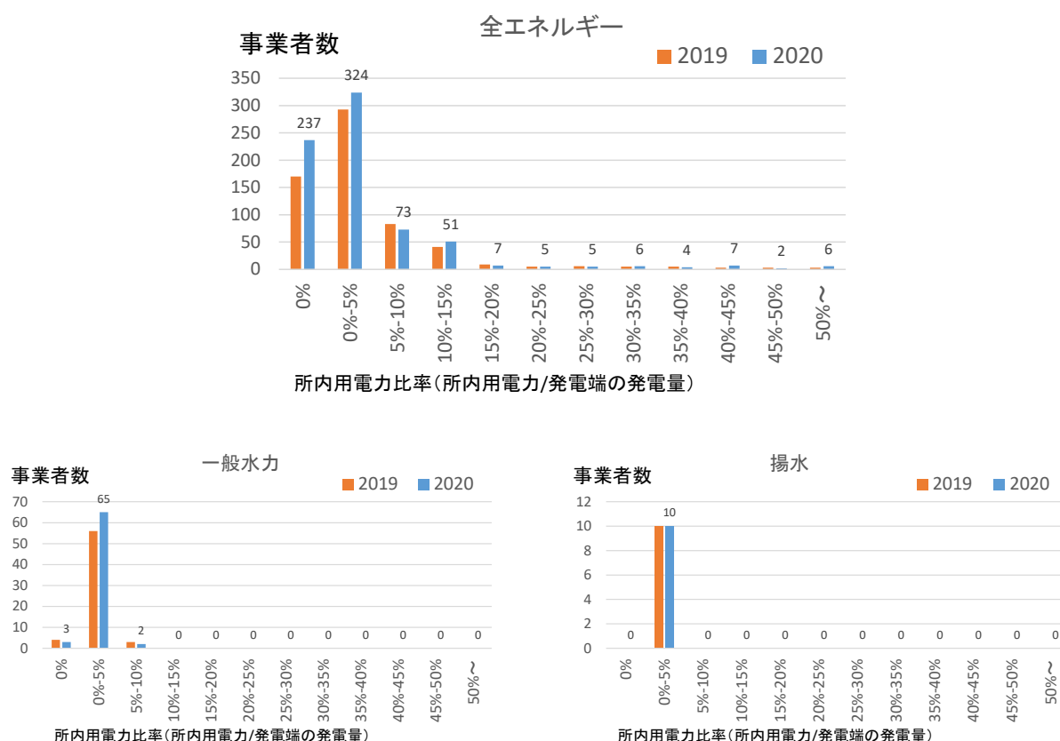
図2.4-4 2019、2020年度の電源種別所内率の分布
