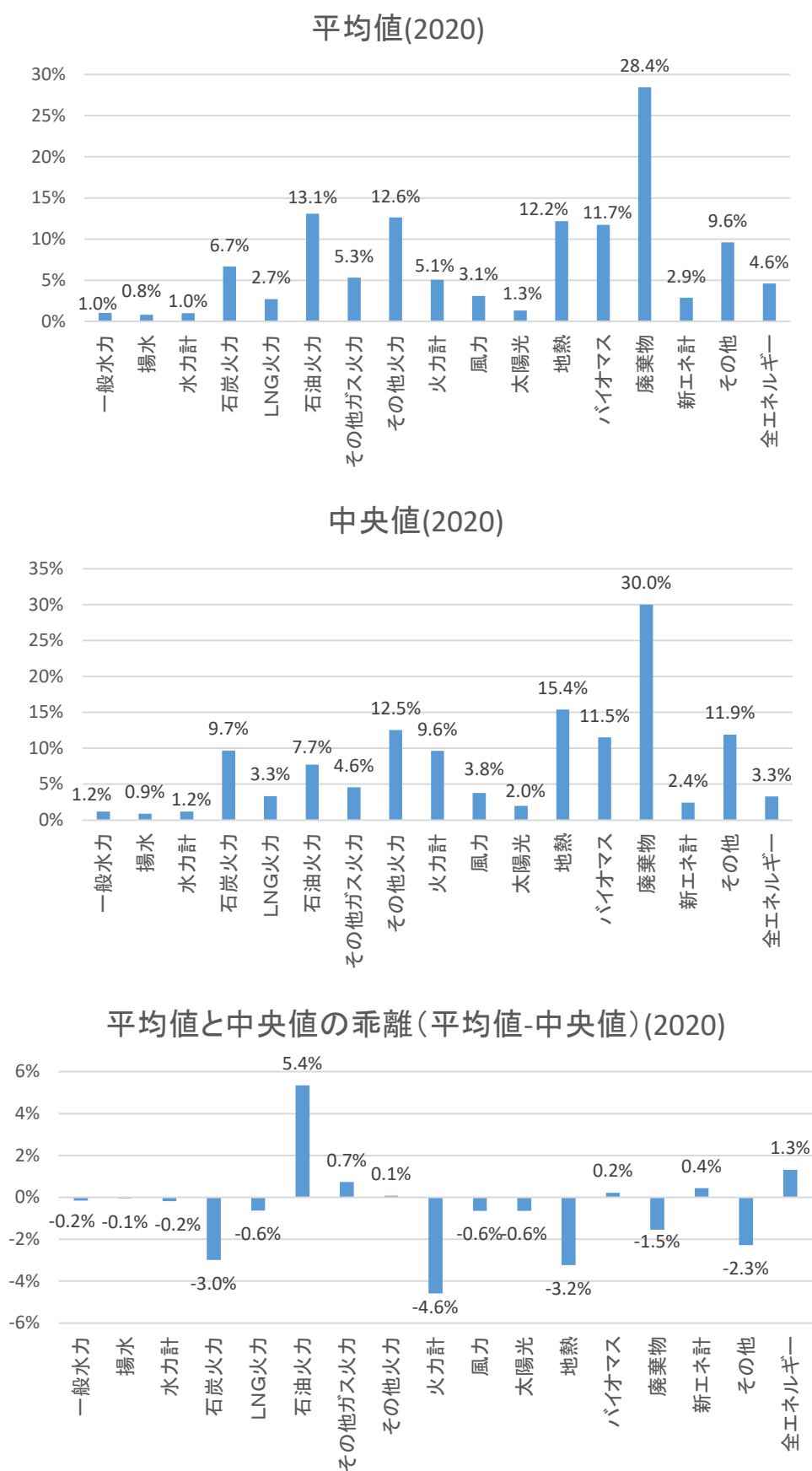
図2.4-2 各電源の2020年度の所内率の平均値と中央値(外れ値補正後)
