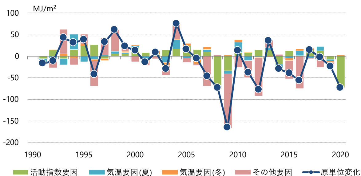
図3.1-56 業務他部門エネルギー原単位(対延床面積)の要因分解(前年度比)
