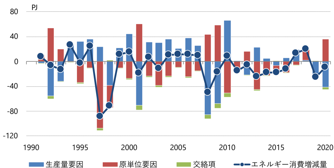
図3.1-45 機械工業の最終エネルギー消費の要因分解(前年度比)
