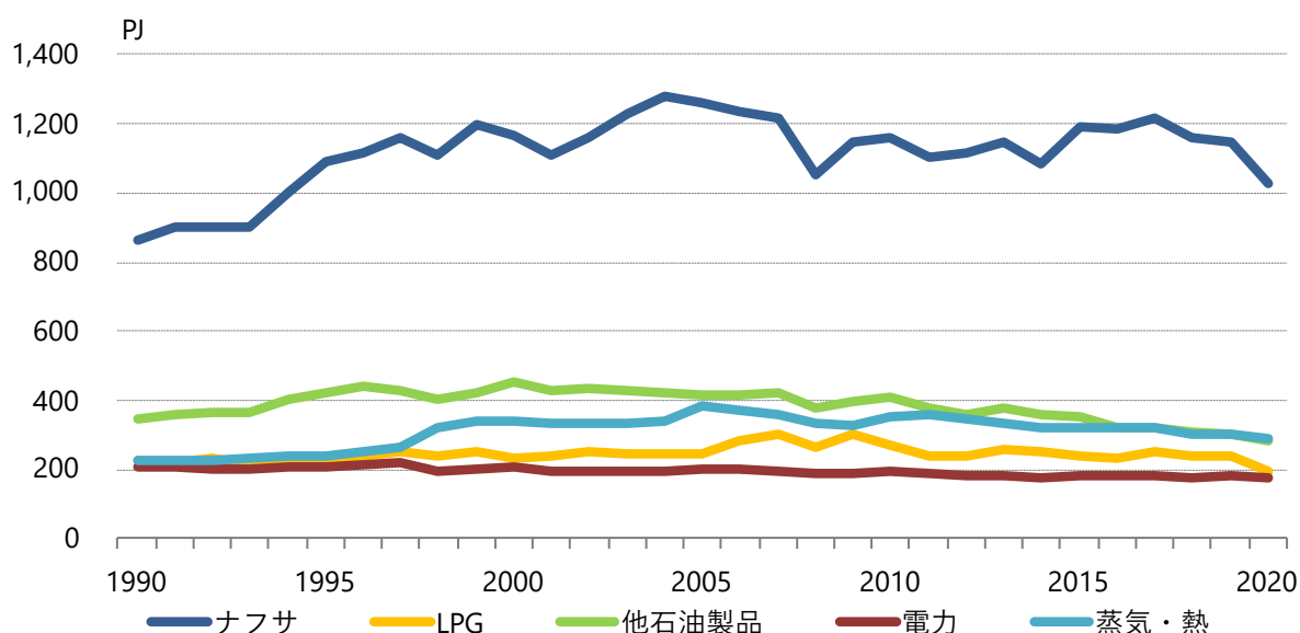
図3.1-24 化学工業の最終エネルギー消費(主要エネルギー源別)
