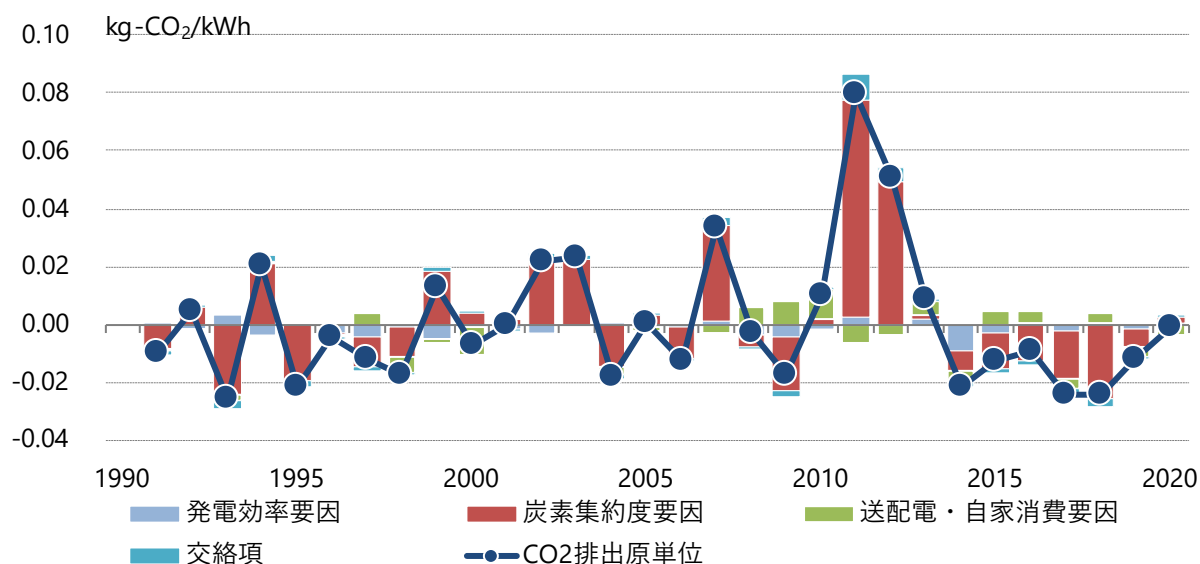
図6.3-18 電力のCO 2 排出原単位(使用端)の要因分解(前年度比)
