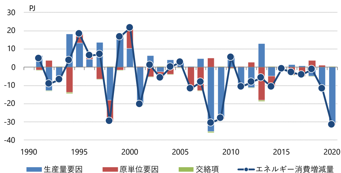
図3.1-30 パルプ・紙・紙加工品工業の最終エネルギー消費の要因分解(前年度比)
