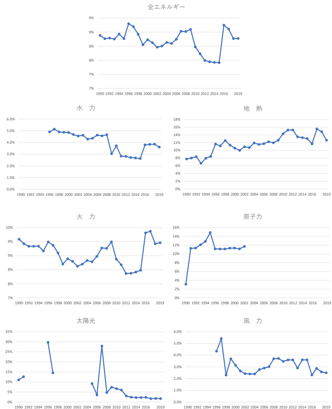
図2.7-2 1,000kW以上の自家用発電の電源種別所内率の推移
