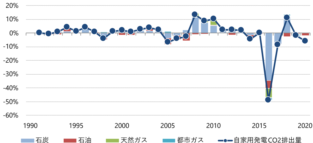
図6.3-25 自家用発電のCO 2 排出量のエネルギー源別寄与度(前年度比)
