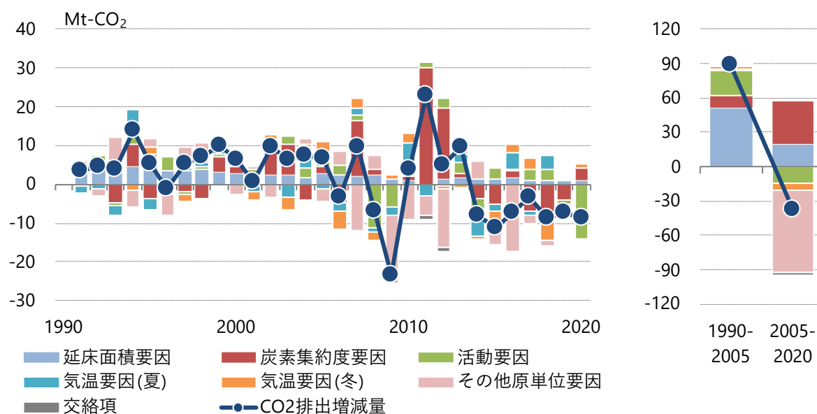
図6.3-7 業務他部門CO 2 排出量の要因分解
