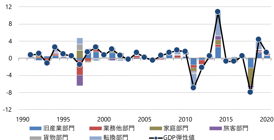
図5.2-2 一次エネルギー国内供給(消費側) GDP弾性値の要因別推移
