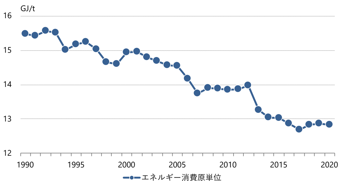
図3.1-29 パルプ・紙・紙加工品工業の紙・板紙生産量あたりエネルギー消費原単位
