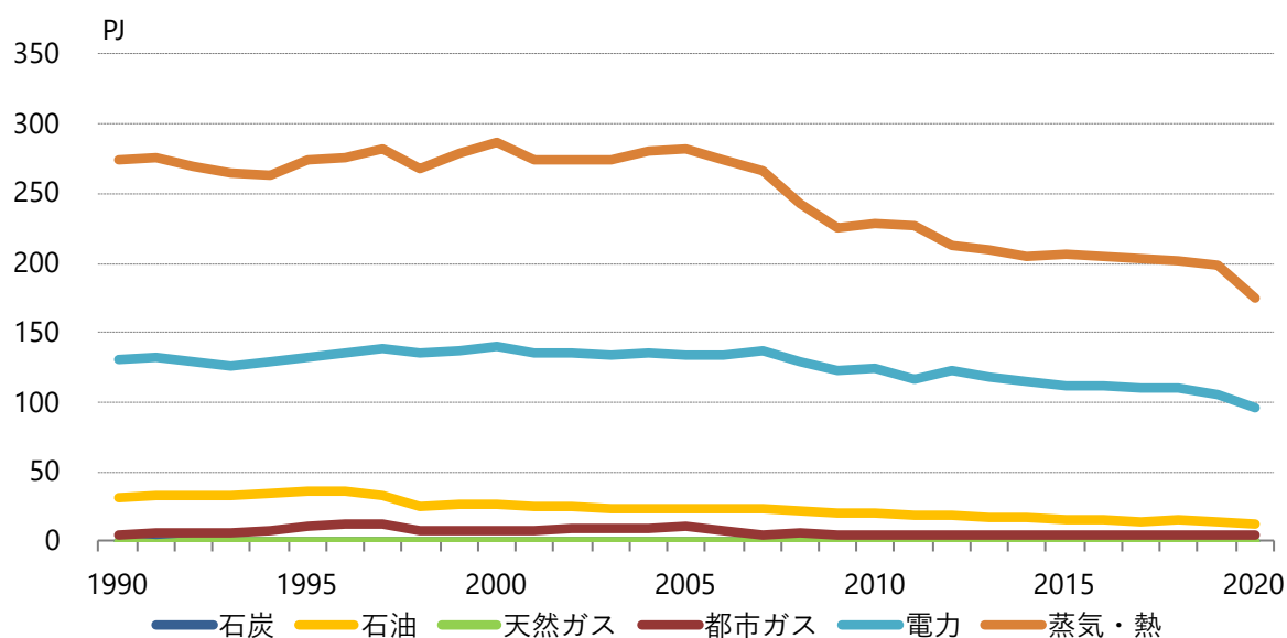
図3.1-31 パルプ・紙・紙加工品工業の最終エネルギー消費(主要エネルギー源別)
