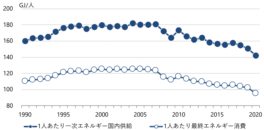
図1.3-2 1人あたり一次エネルギー国内供給・最終エネルギー消費
