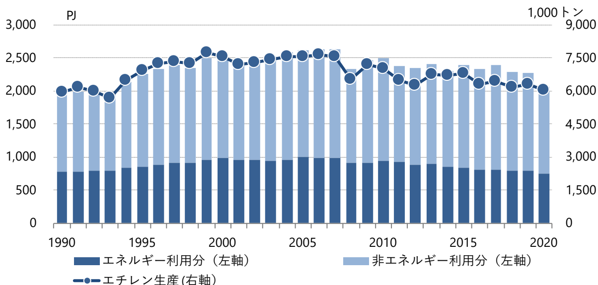
図3.1-18 化学工業の最終エネルギー消費とエチレン生産量
