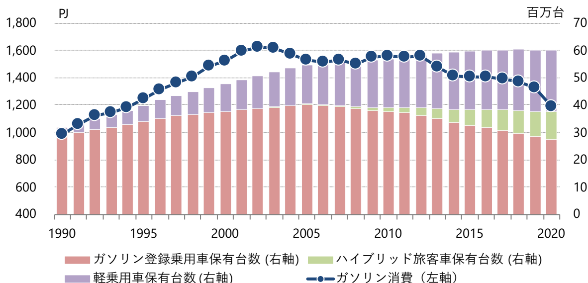
図3.3-10 乗用車ガソリン消費量とガソリン乗用車保有台数
