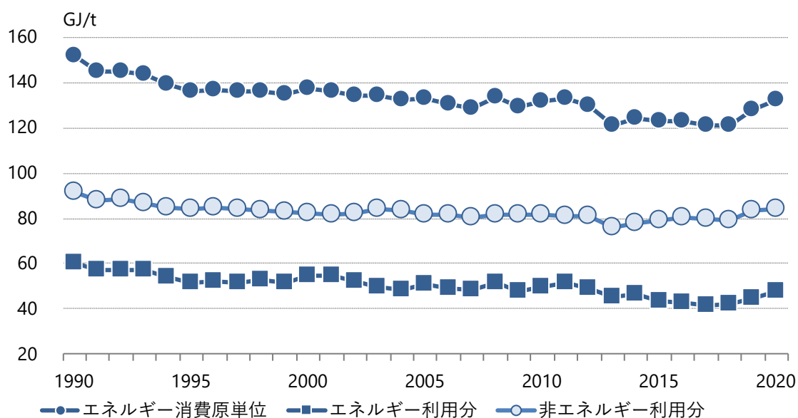
図3.1-20 化学工業のエチレン+BTX生産量あたりエネルギー消費原単位
