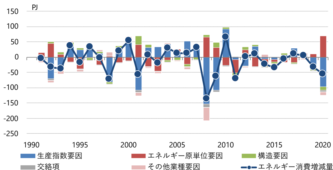
図3.1-10 製造業電力消費の要因分解
