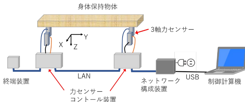
図 7 計測用力センサー全体システム構成概要図
