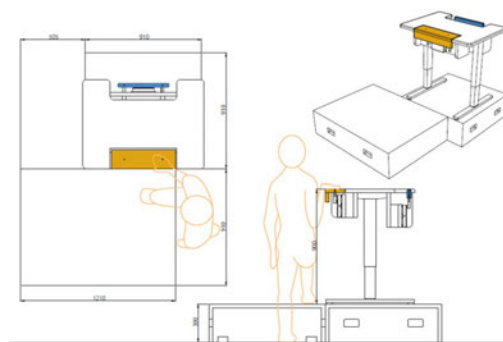
図 4 計測実験イメージ (3)
