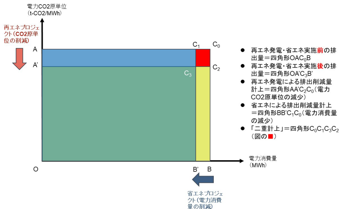
図 2-1 再エネ発電プロジェクトと省エネ(節電)プロジェクトの関係
