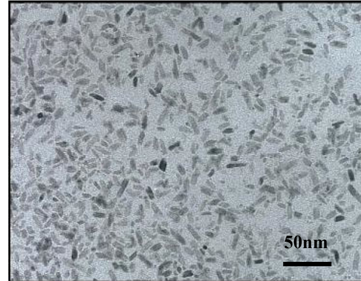
Rutile type TiO 2
