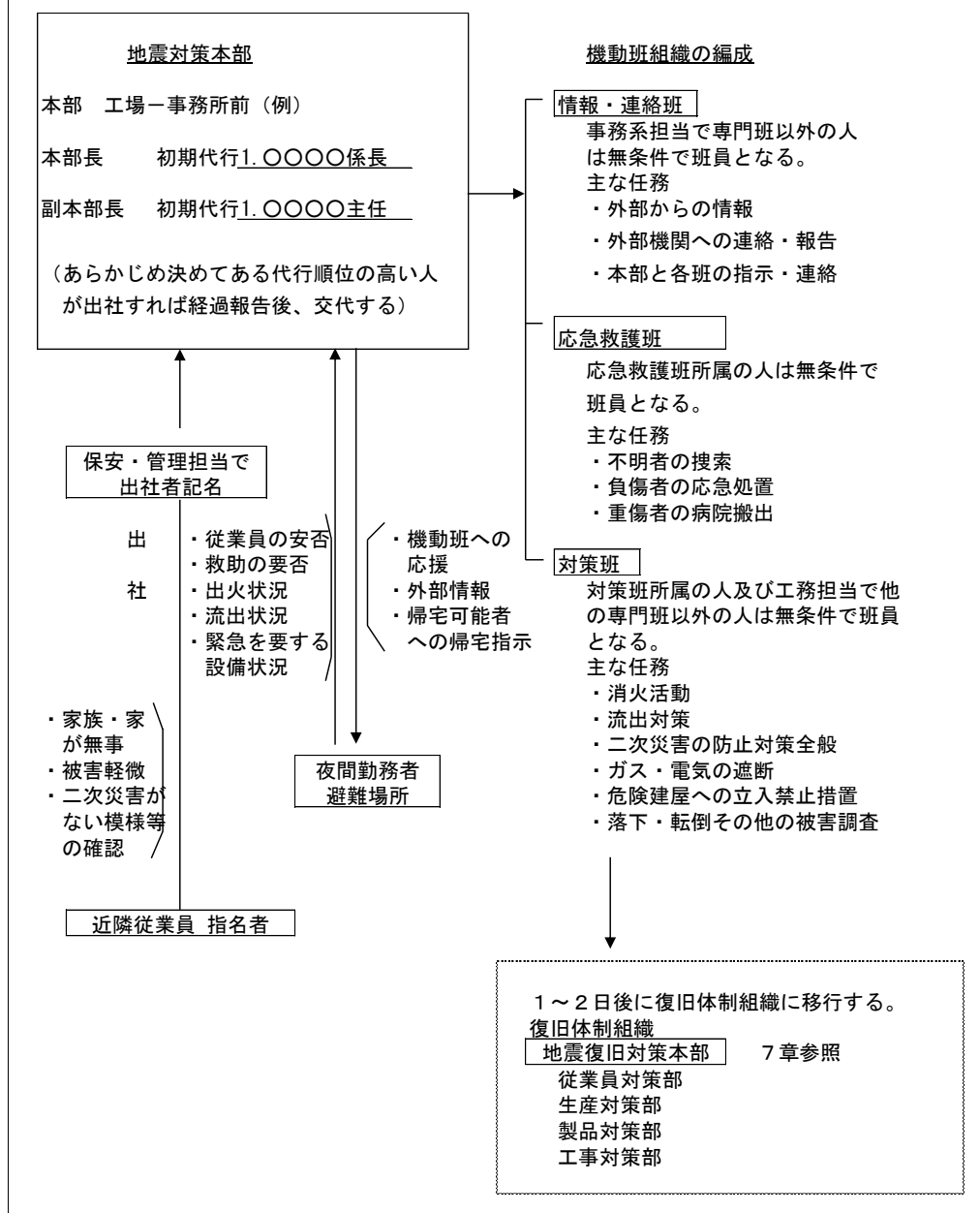
図3 地震発生時の対応体制の例
