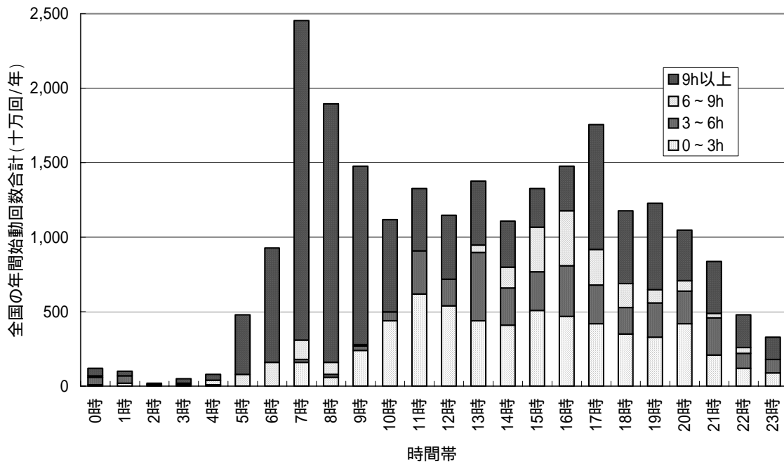
図 12-20 全国における時間帯ごとのソーク時間別年間始動回数の合計の推計結果 (自家用ガソリン小型乗用車、約 2 千 4 百万台)
