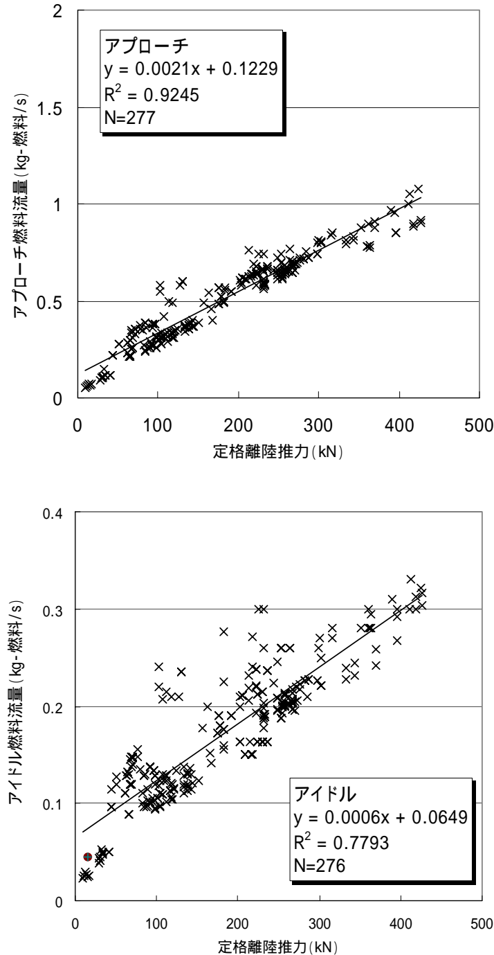
図 17-2 定格離陸推力と燃料流量の関係(アプローチ及びグランドアイドル)
