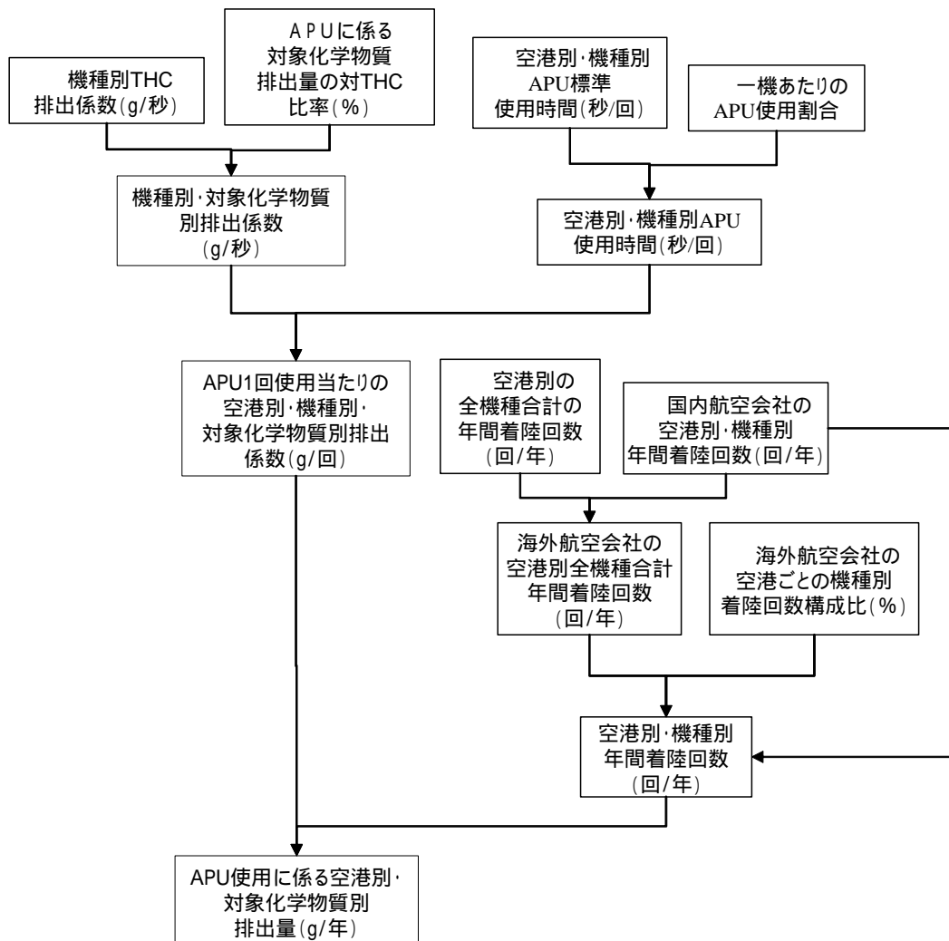
図 17-6 APUに係る排出量の推計フロー
