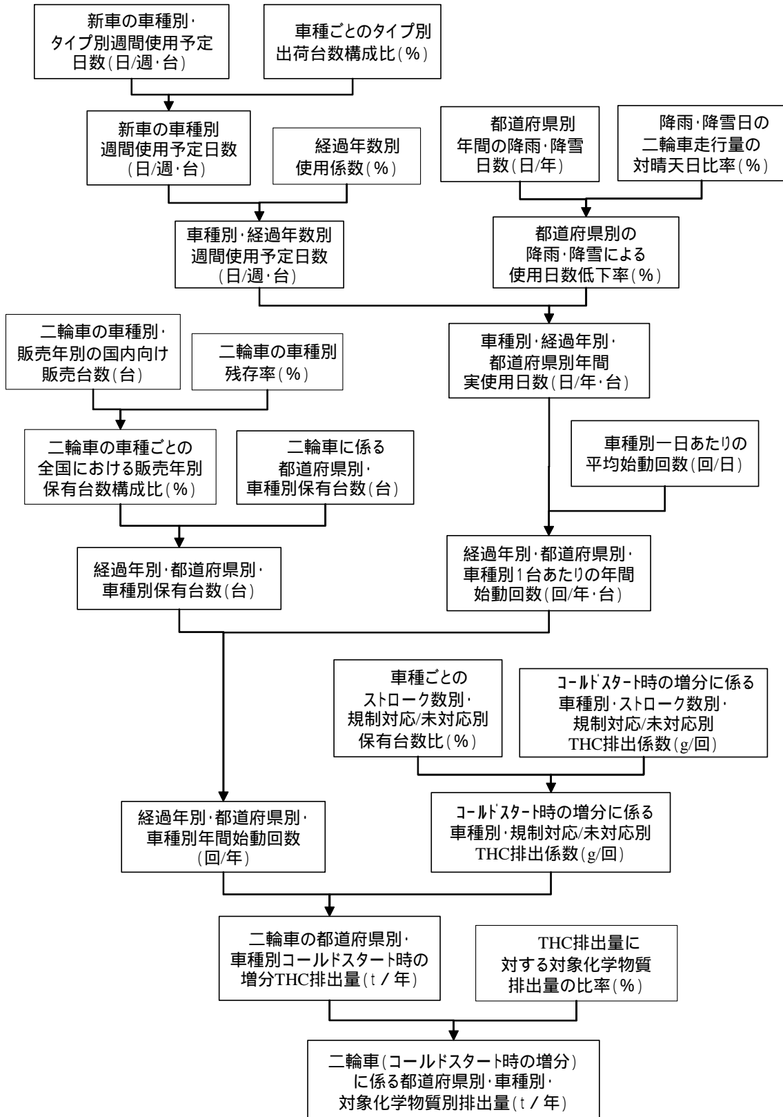
図 13-14 コールドスタート時の増分に係る排出量推計フロー
