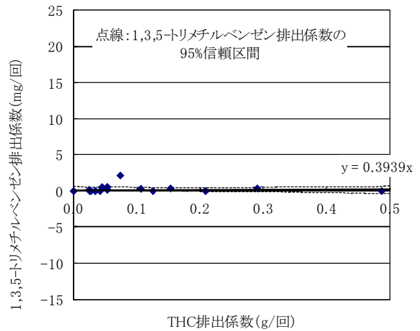
図11-42 ディーゼル自動車(コールドスタート時の増分)に係る THC 排出量と 対象化学物質別排出量の比率(その1)
